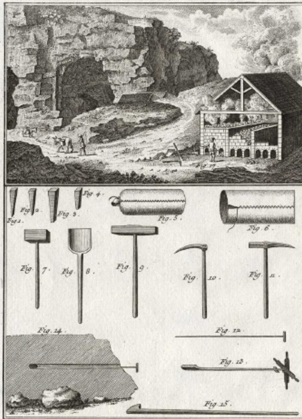
Architecture Maçonnerie, carrier - Plâtrier.
