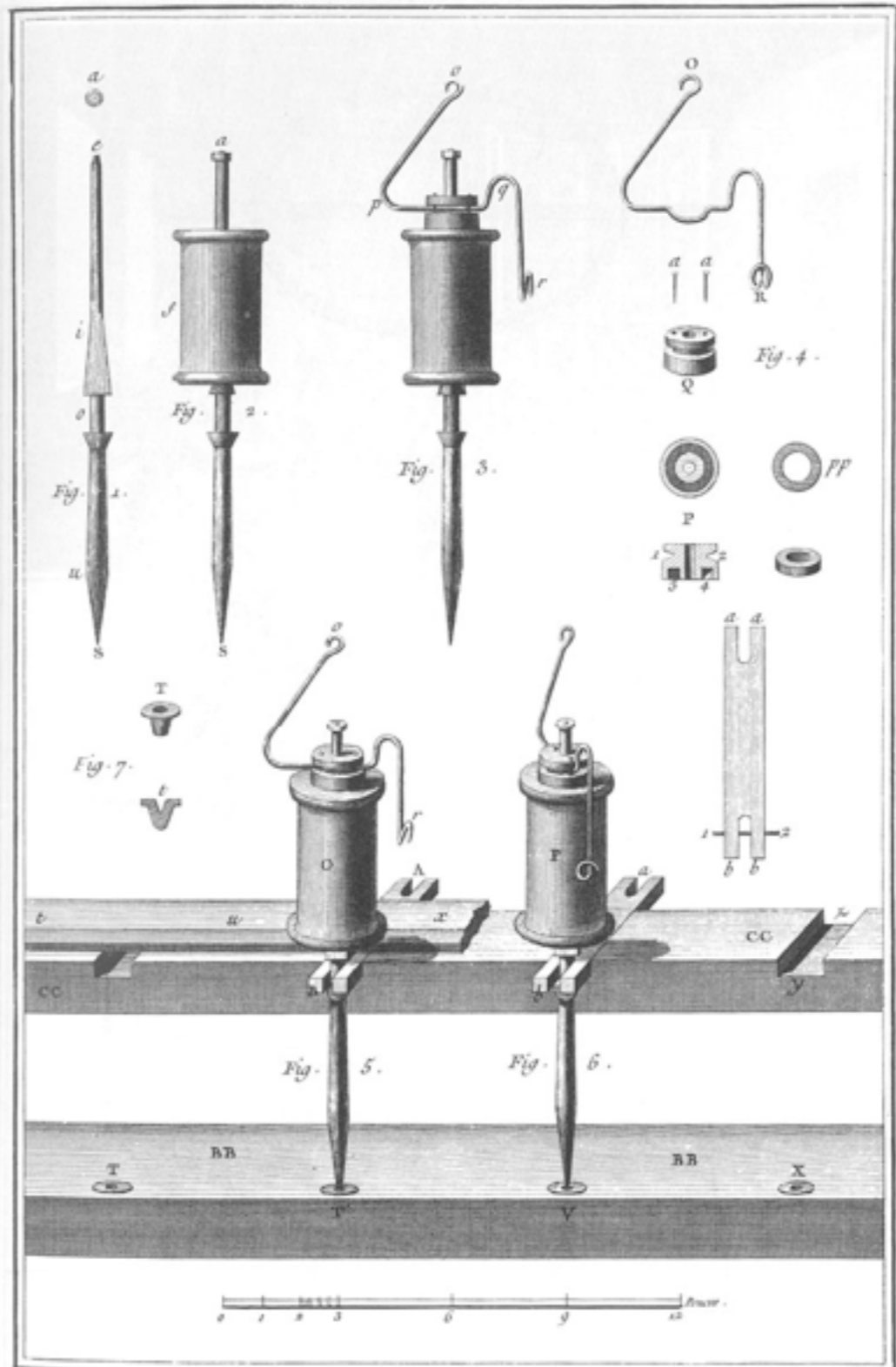
Soierie, Moulin pour Organiser les Soies, Construction et Développement des Fusées. P
