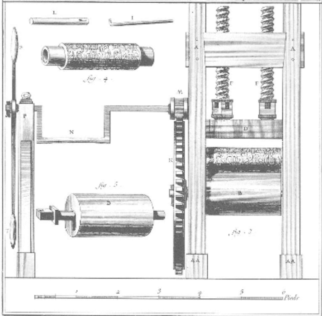
Découpeur et Gausseur.
