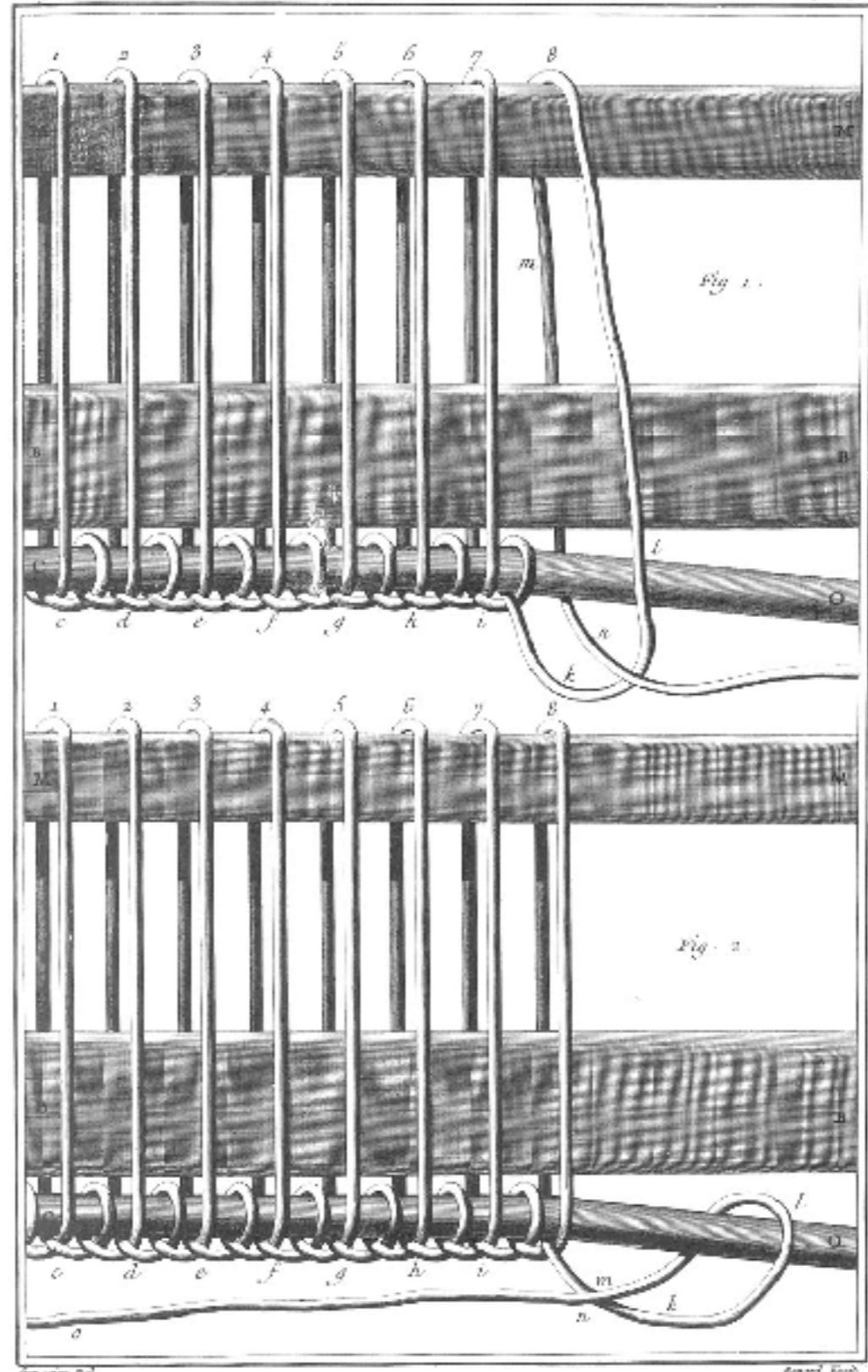
Soierie, Formation du Bas des Lissas et Maniere de Natter. kkkk
