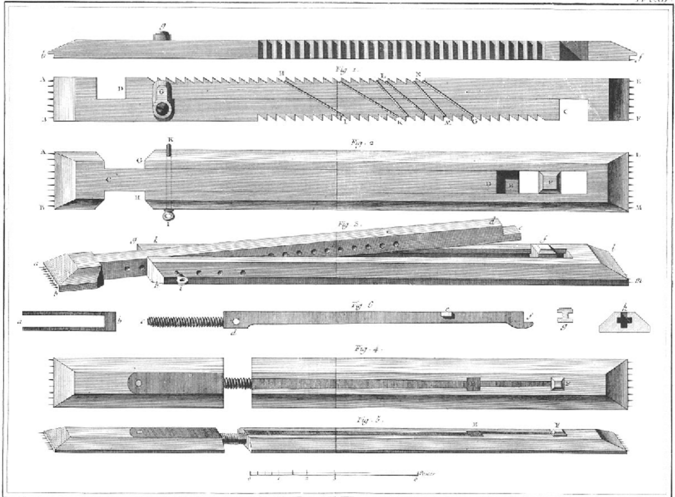
Soierie, Tempia de différentes sortes, Tempia à Corde, Tempia à Bouton et Tempia à Vis.
