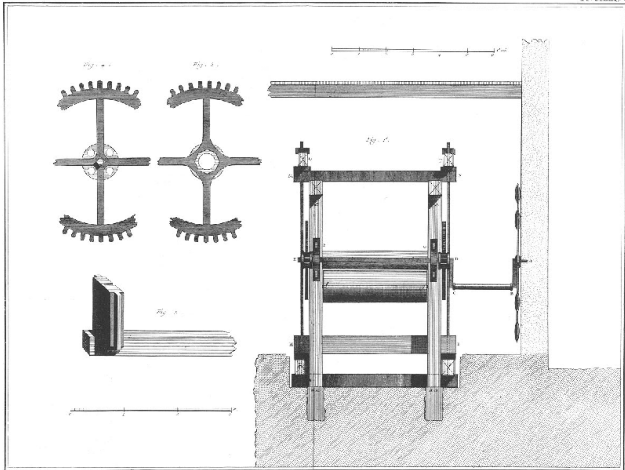
Soierie, Révélation antérieure de la Machine servant à dévider les Bâffes et Développemens de quelques uns de ses Parties. U U U U
