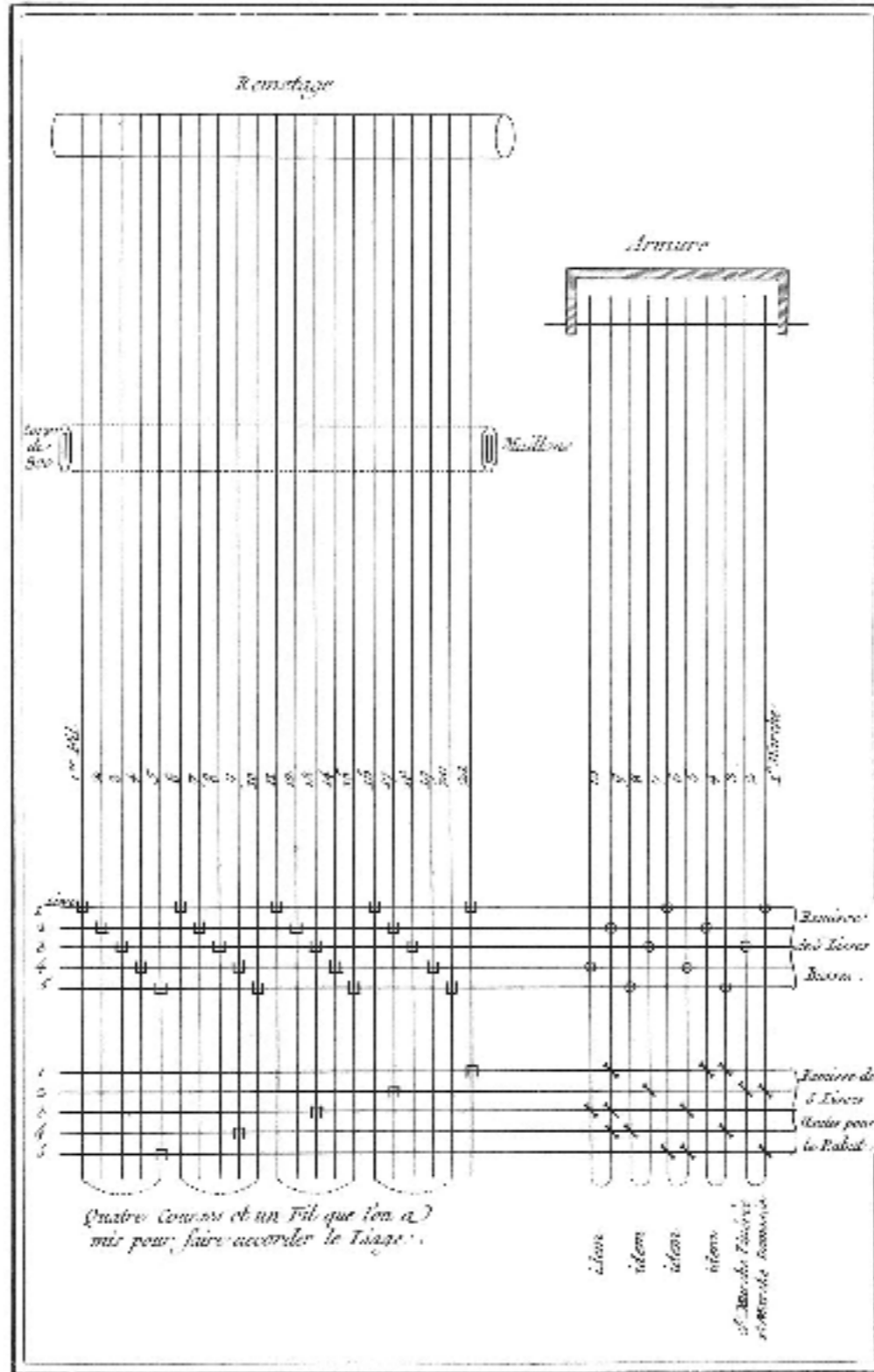
Soierie, Florentine Damassée avec un Lizere
