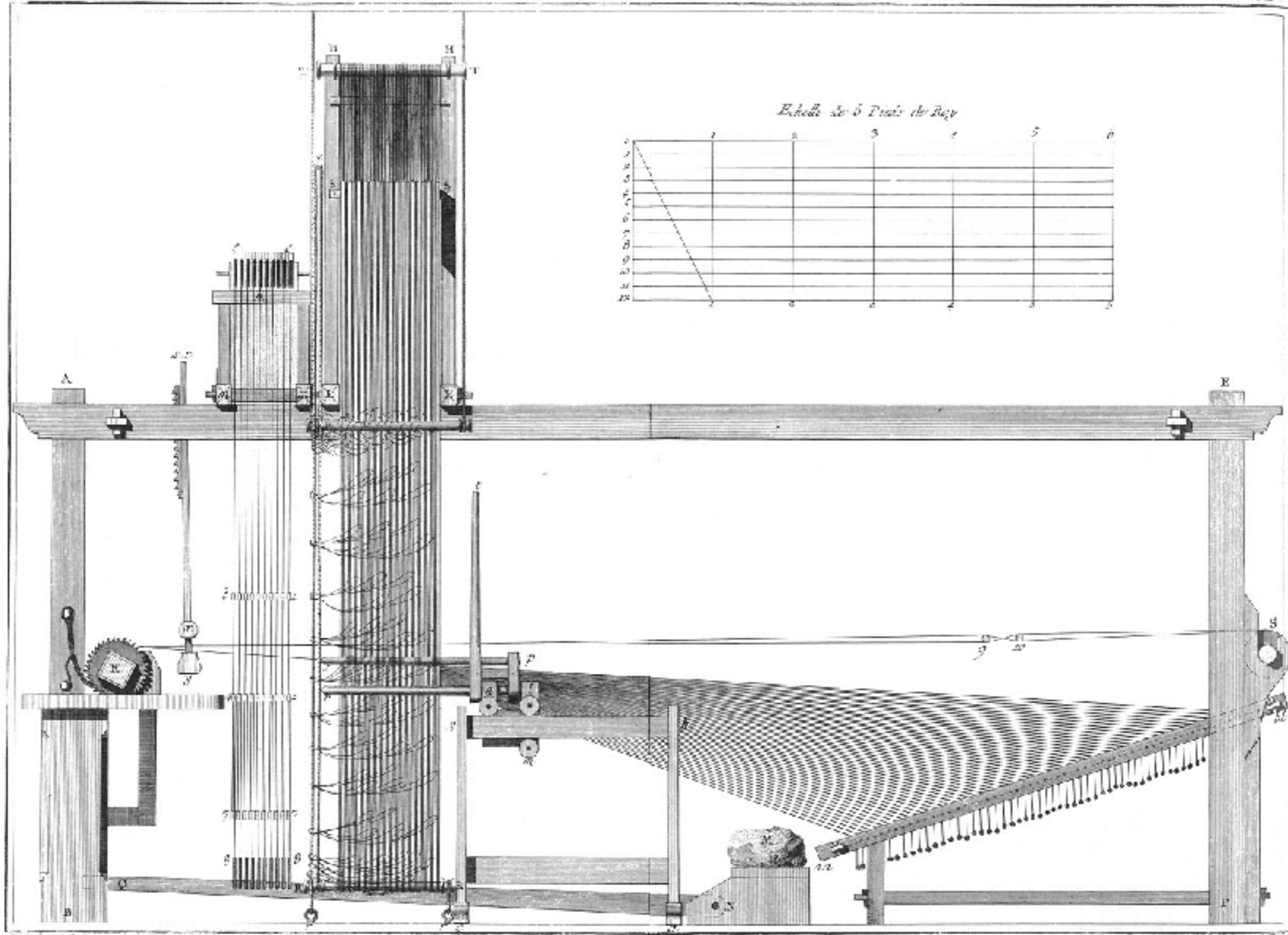
Soierie, Velours. Elevation Latérale du Mûrier pour fabriquer le Velours Ciselé. Vu dans l'instant qui précède celui de la Ture.
