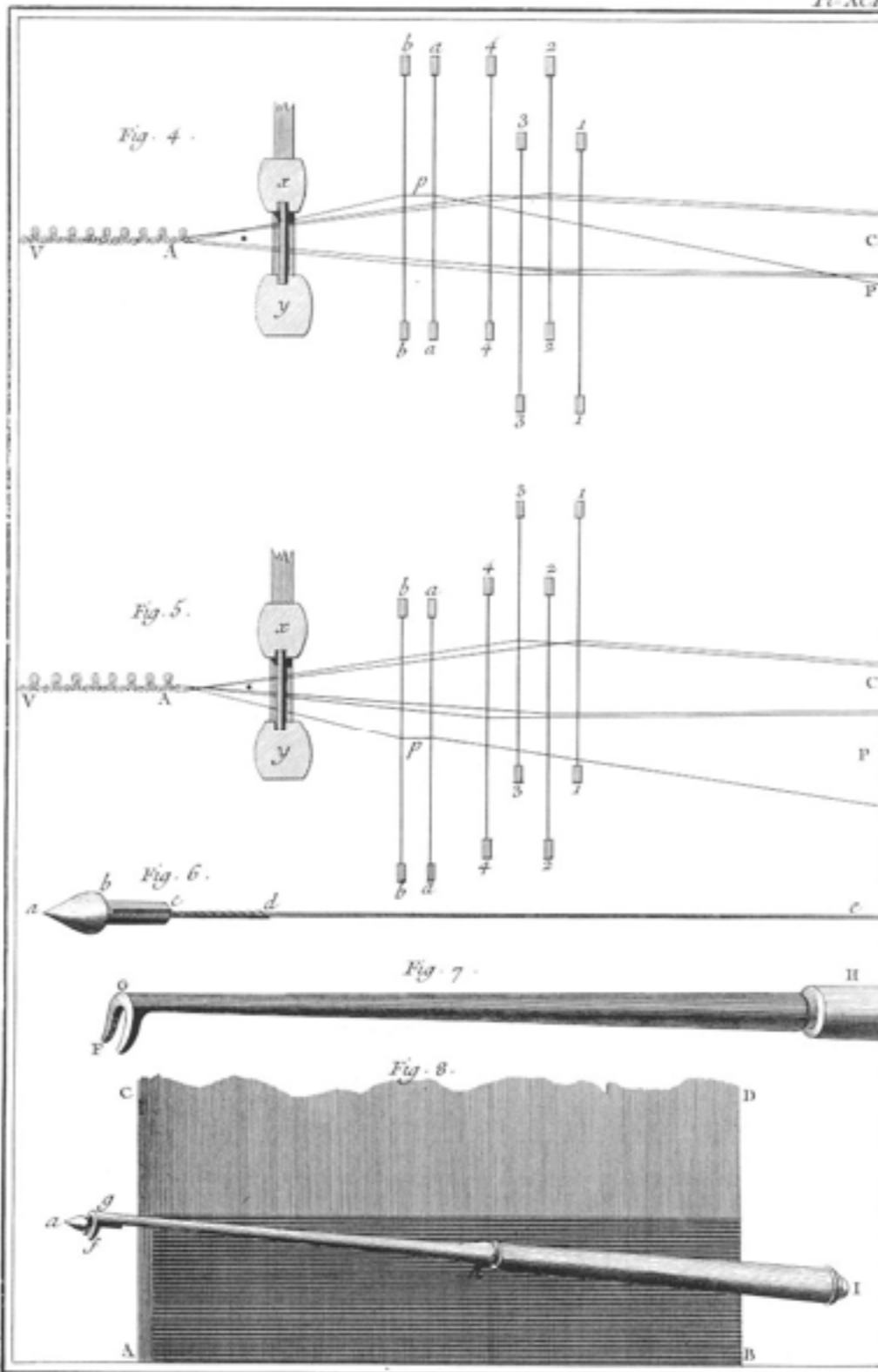
Soierie, Velours Frizé. 4°. second Coup de Navette. 999. 5° troisième Coup de Navette, Fers de Frizé garnis de leurs Pedonnes.
