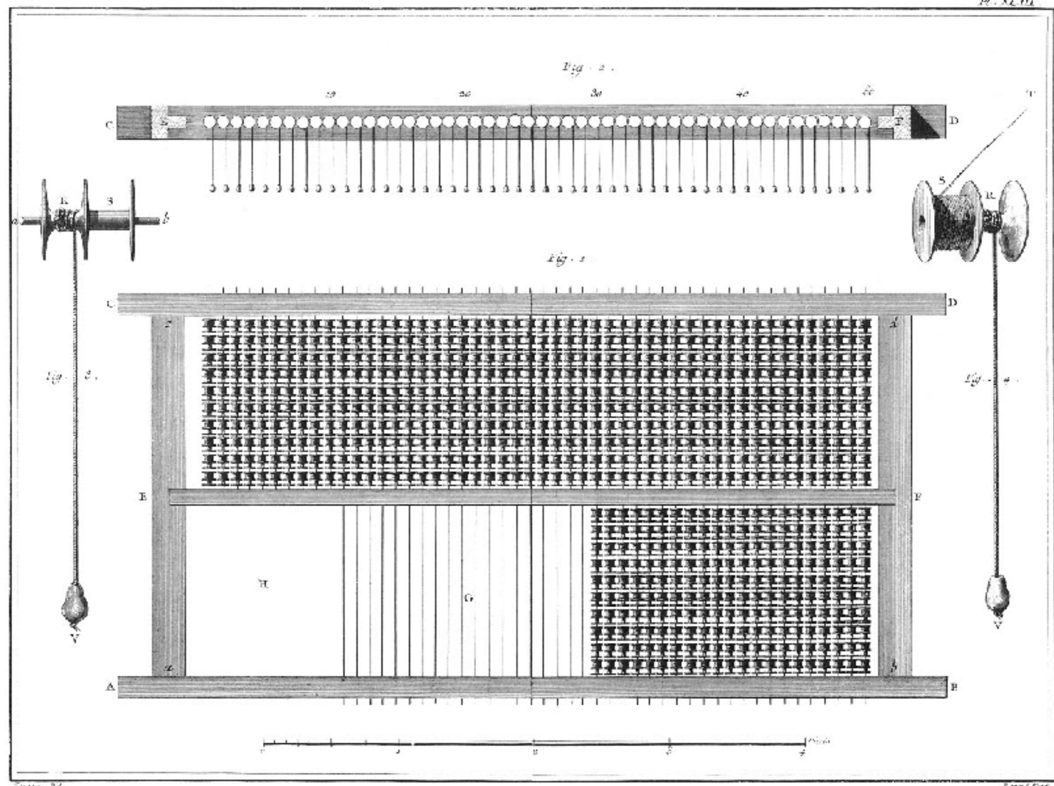
Soierie, Velours Ciselé. Plan de la Cantre et Développement des Bouquets.
