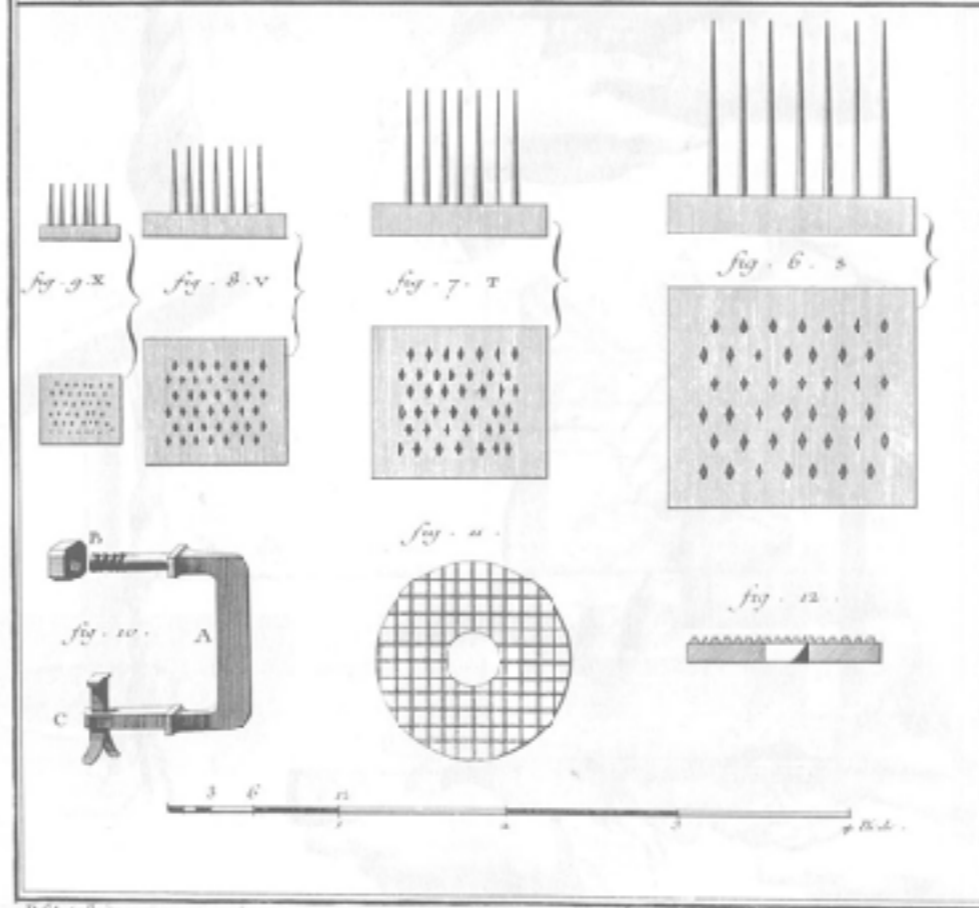
D'États OÉconomie Rustique, Culture et Travail du Chanvre.
