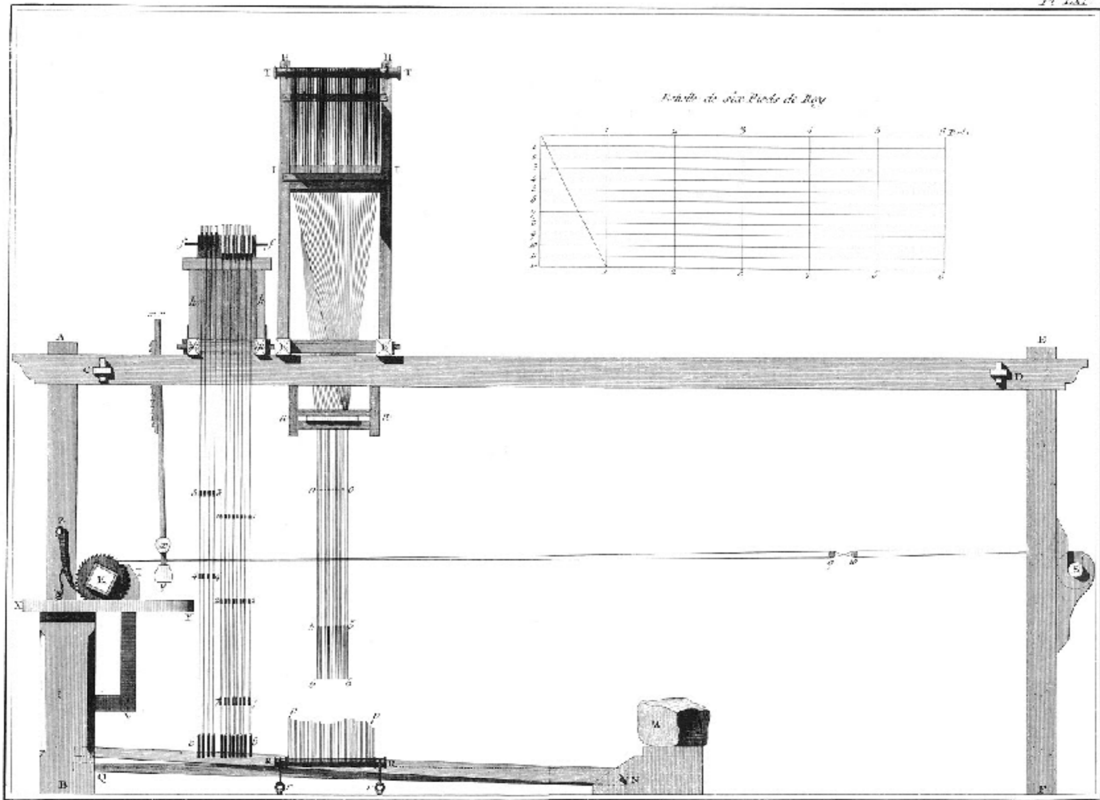
Soierie; Étoffes Brochées. Élévation Latérale du Métier pour fabriquer les Étoffes Brochées.
