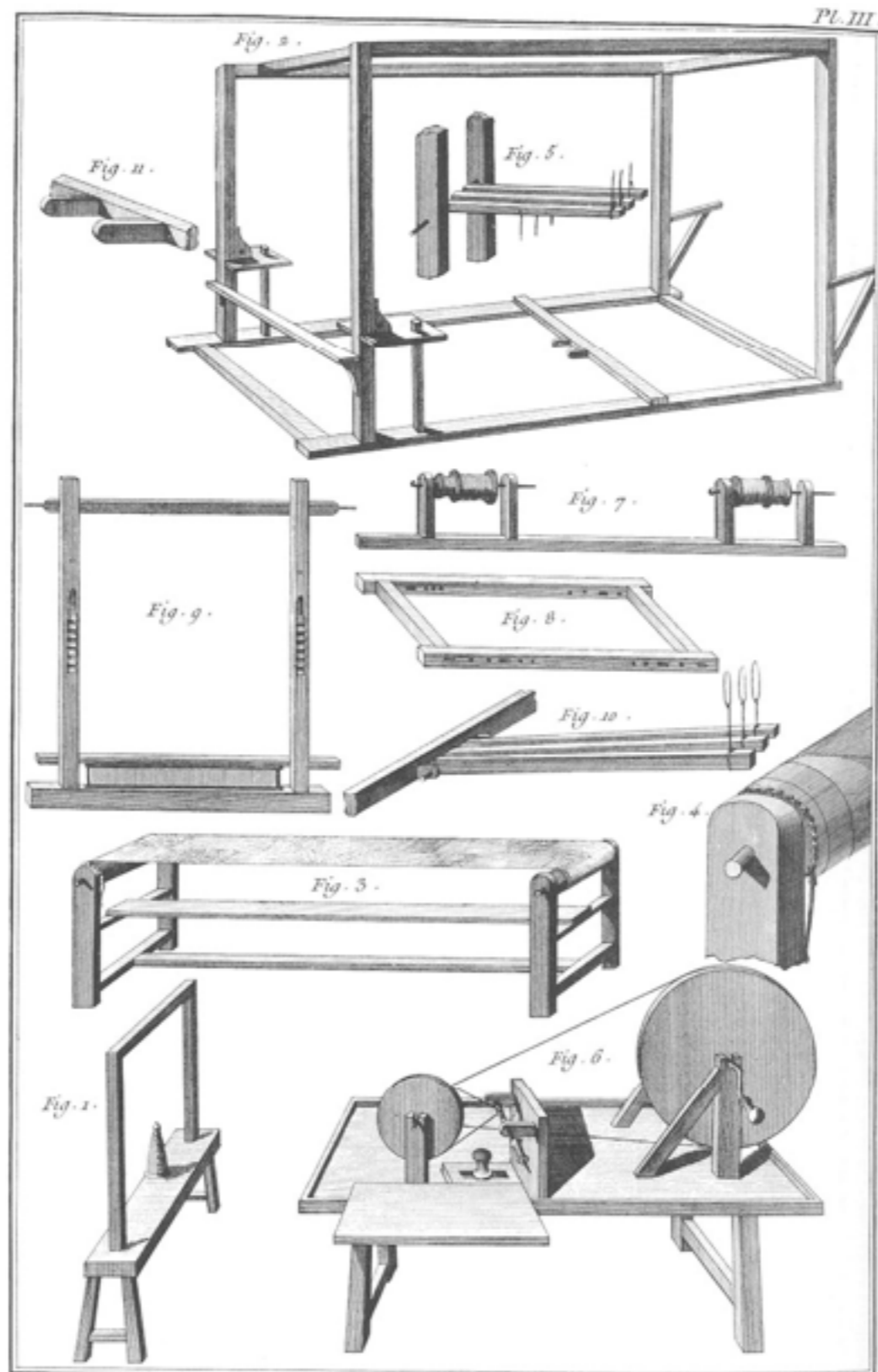
Gazier, Développement du Mélier à Gaze &c.
