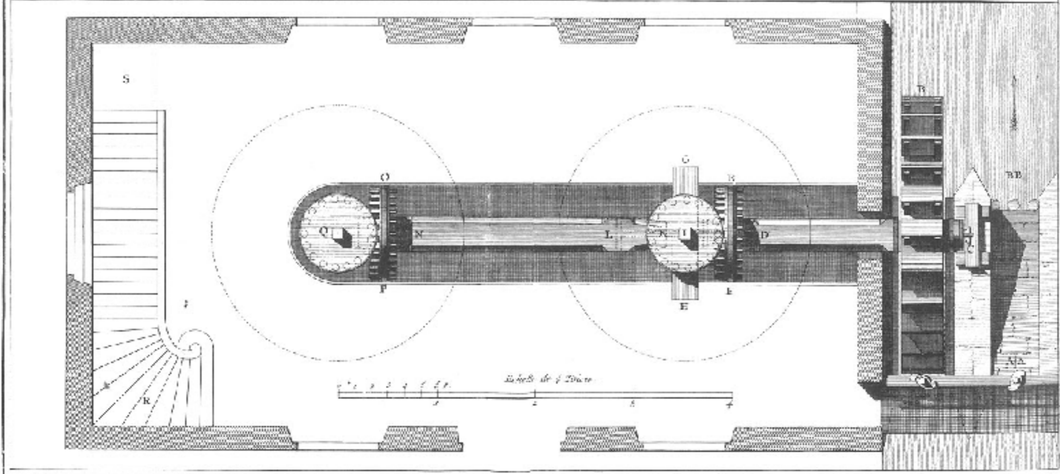
Soierie, Moulin de Piedmont en Perspective, et Plan de la Mécanique au-dessous du Rez de Chaussée. F
