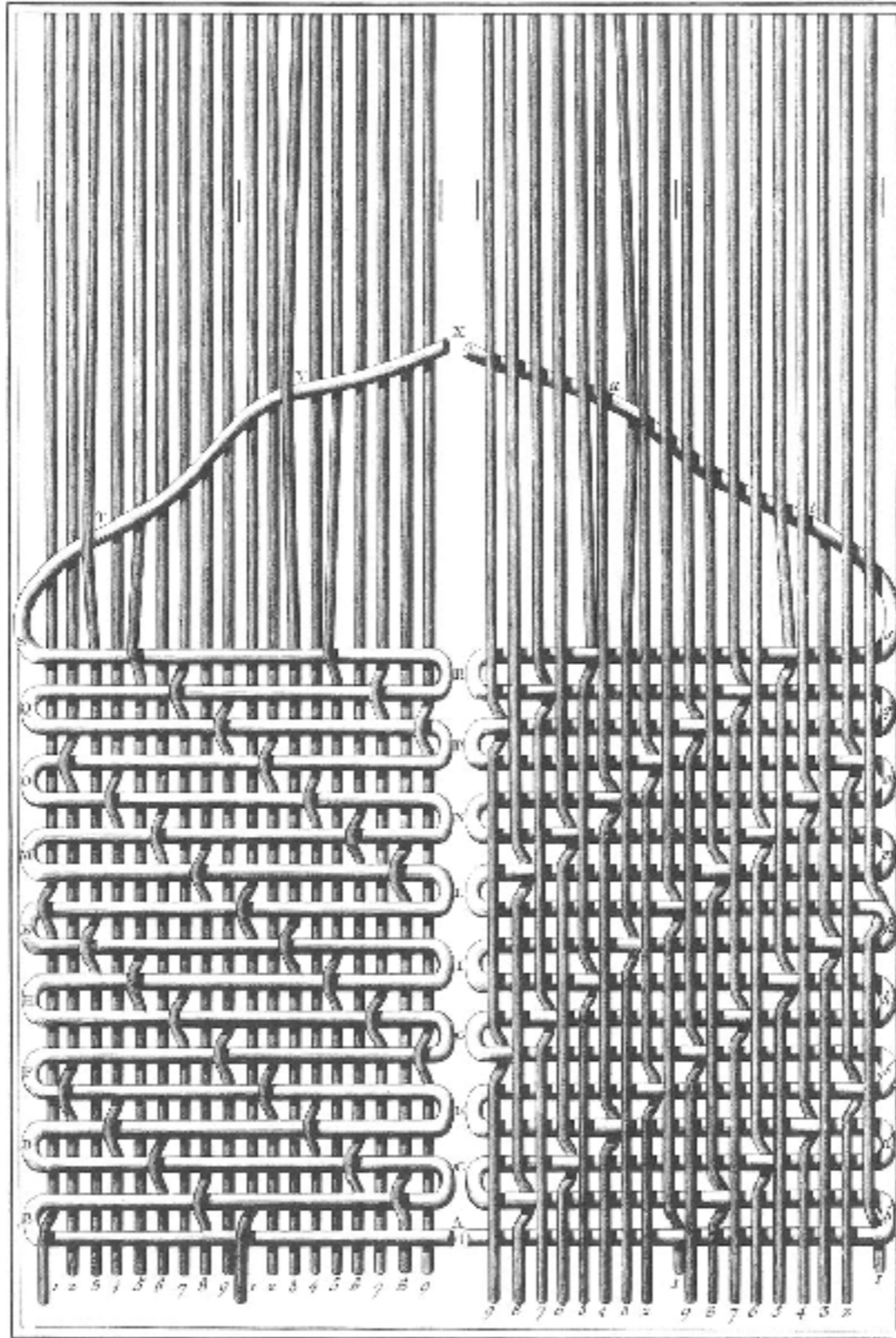
Soierie, satin à 9 lisses vu du côté de l'envers et du côté de l'endroit.
