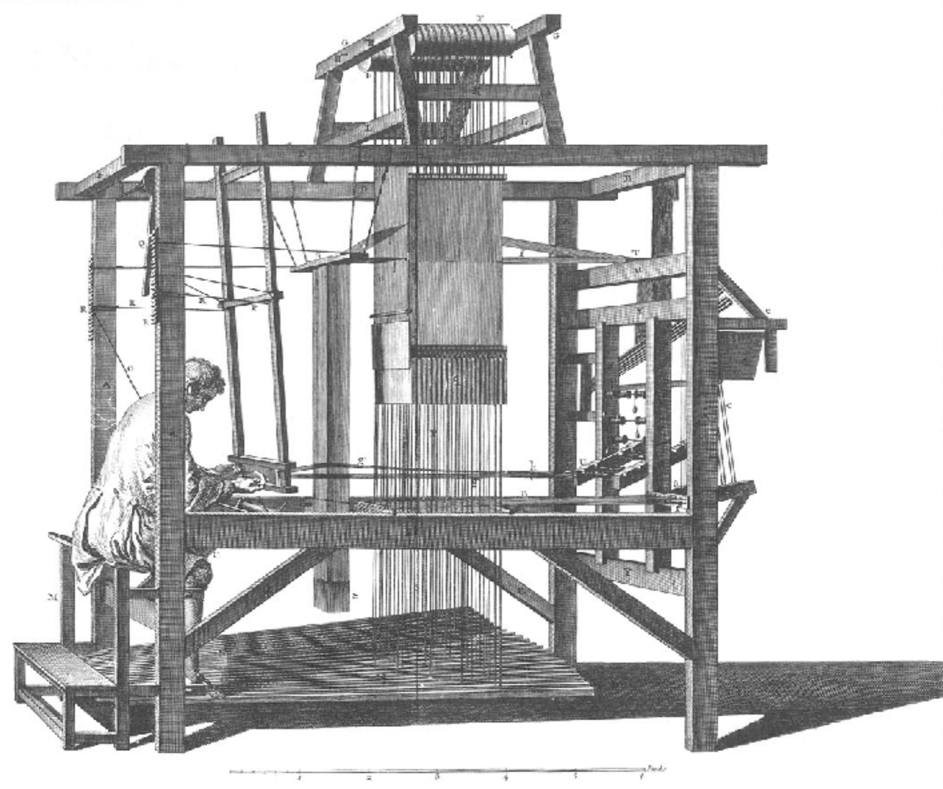
Passementerie, Mètier à faire le Galon, ? .
