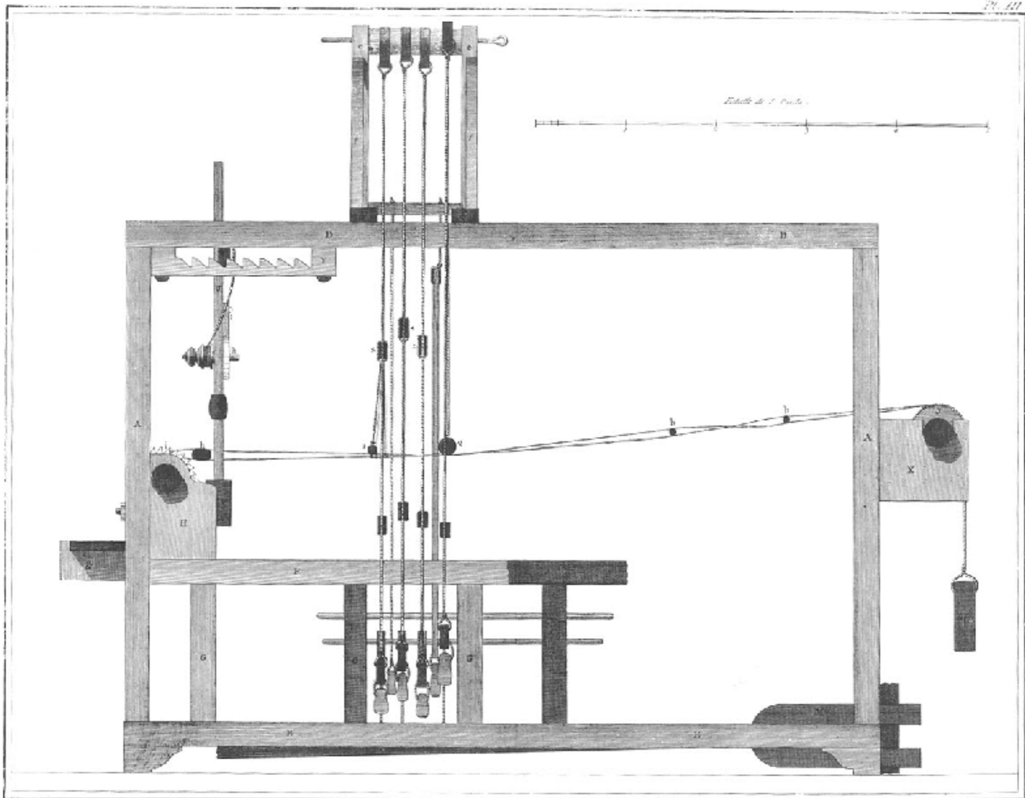
Élévation Latérale du Métier à Marli.
