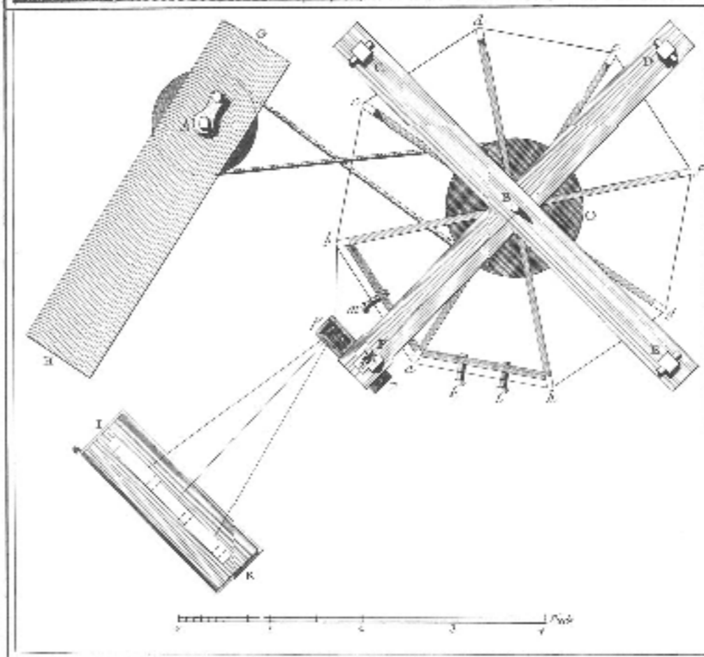
Soierie, l'opération d'ourdier la chaîne des litesffes. 2.
