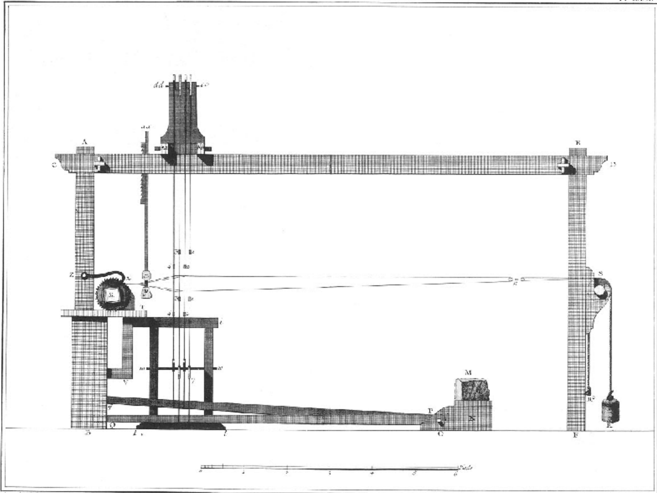
Soierie, Elevation Géométrale de la partie Lateralle du Mélier pour fabriquer les Basses unies comme Tuffetas, Satin et Serge II
