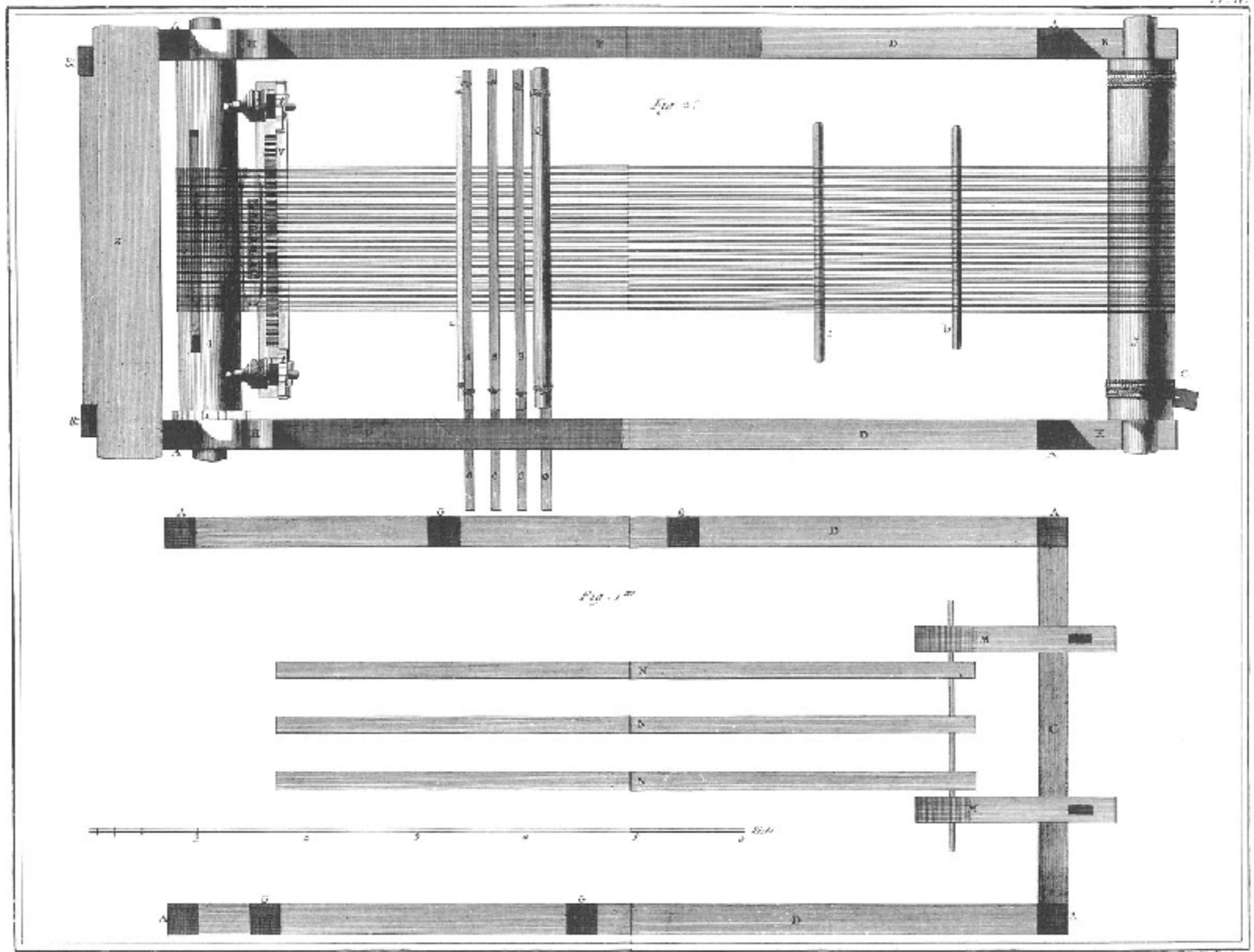
Plans du Métier à Marli.
