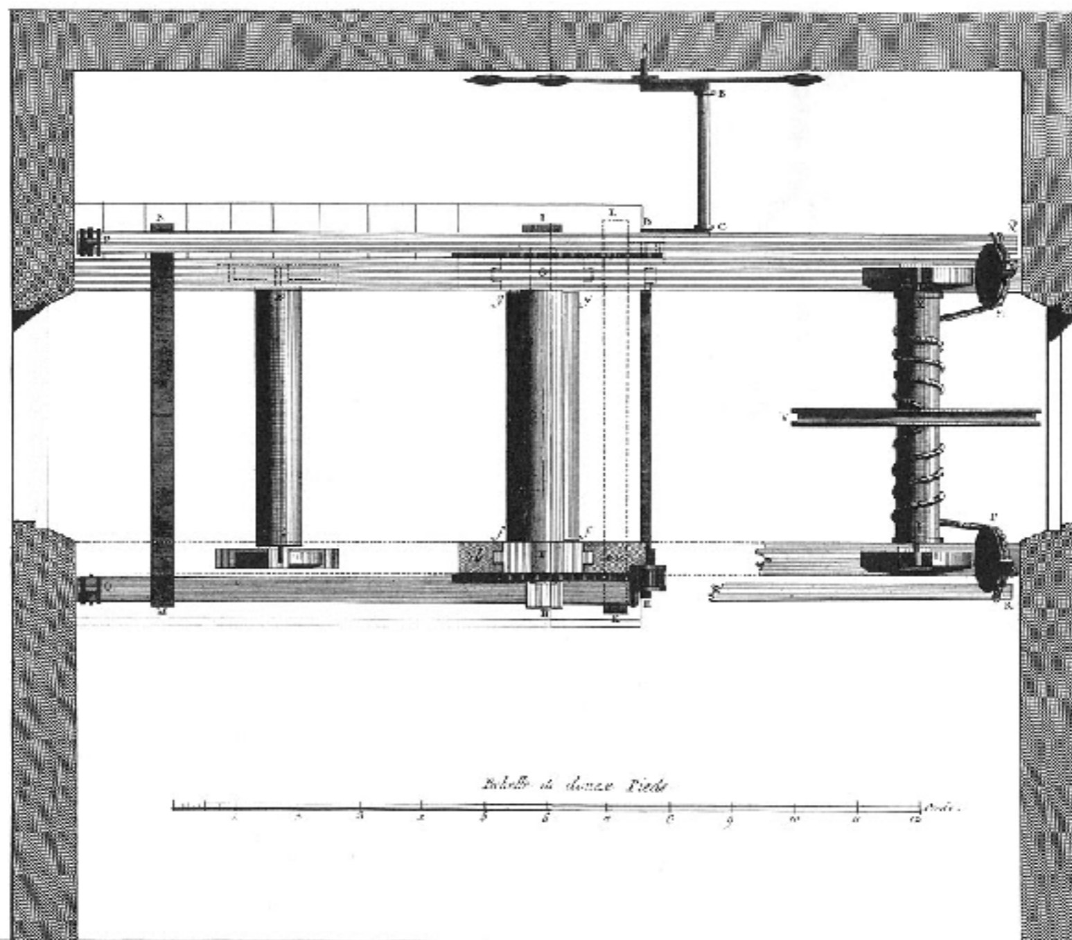
Soierie, Plan de la Machine servant à Cilindrer les Étoffes.
