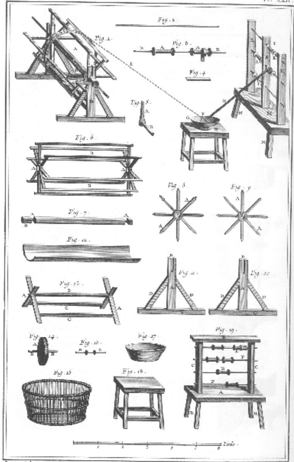
Passementerie, détails des Outils propres à faire la Nonpareille.
