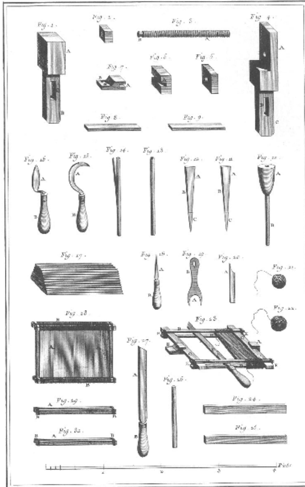
Passenterie, détails pour la façon des Peignes.
