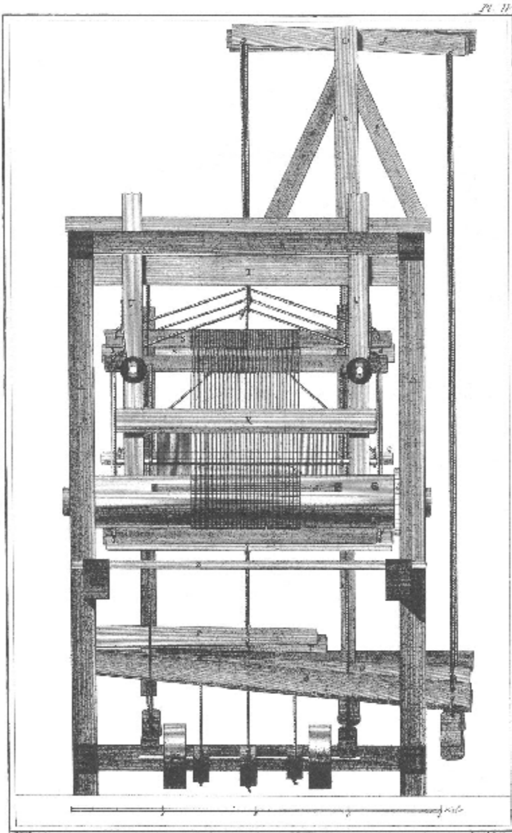
Élévation en face du Métier à Marley.
