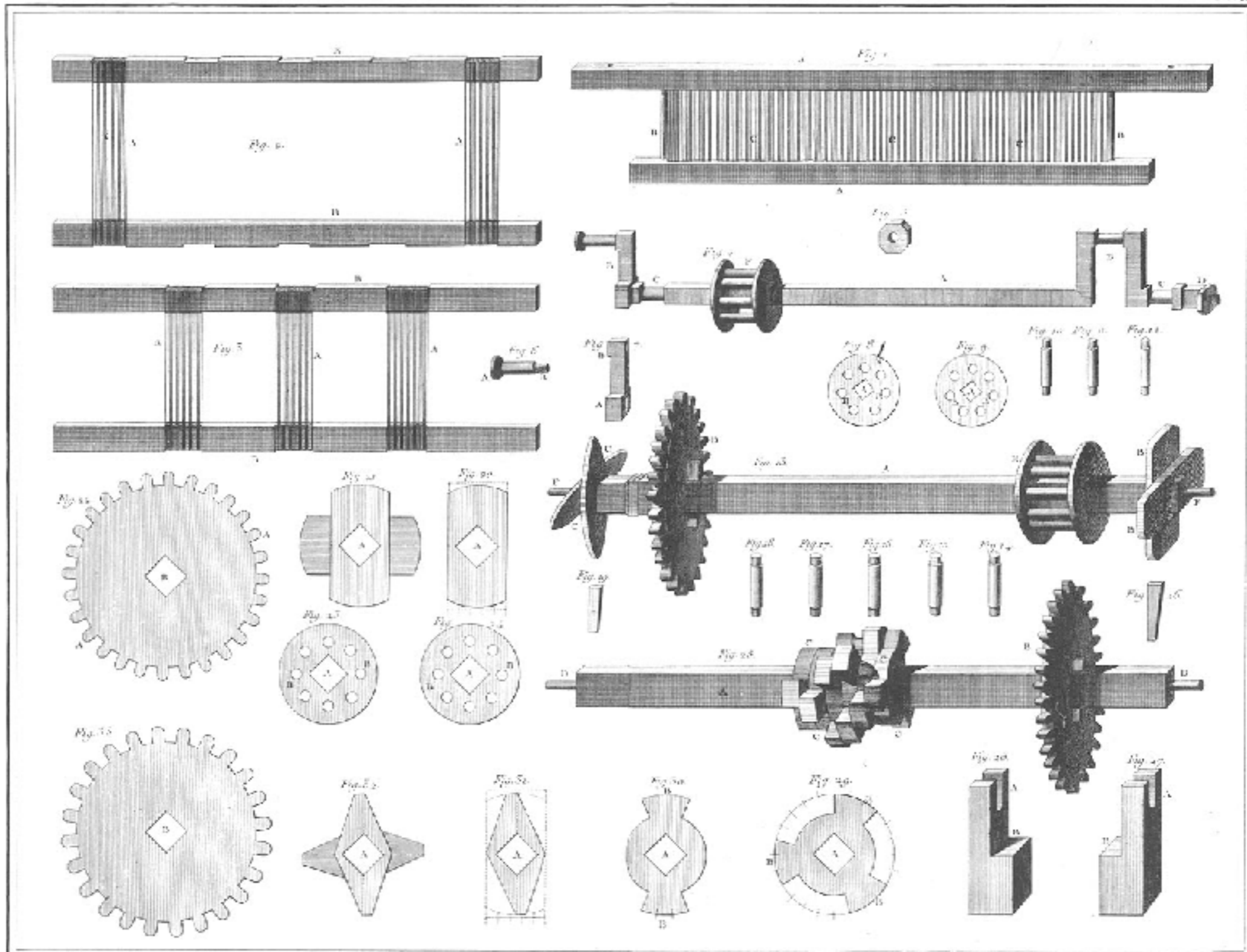
Métier à faire le Ruban, Développement.
