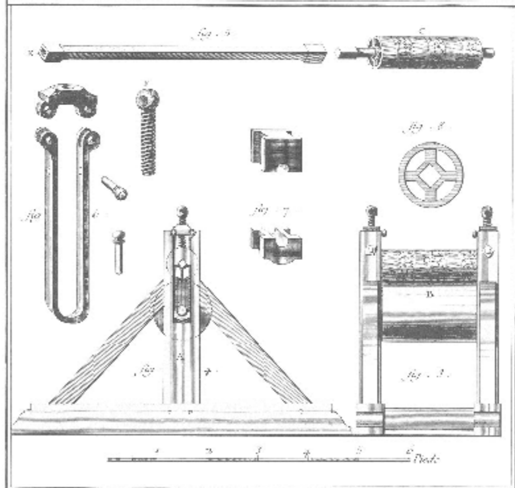
Découpeur et Gouffreur.
