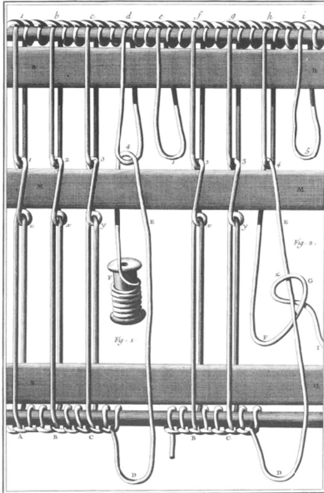
Soierie, Lisses à noeuds premier et second temps de la formation de la maille.
