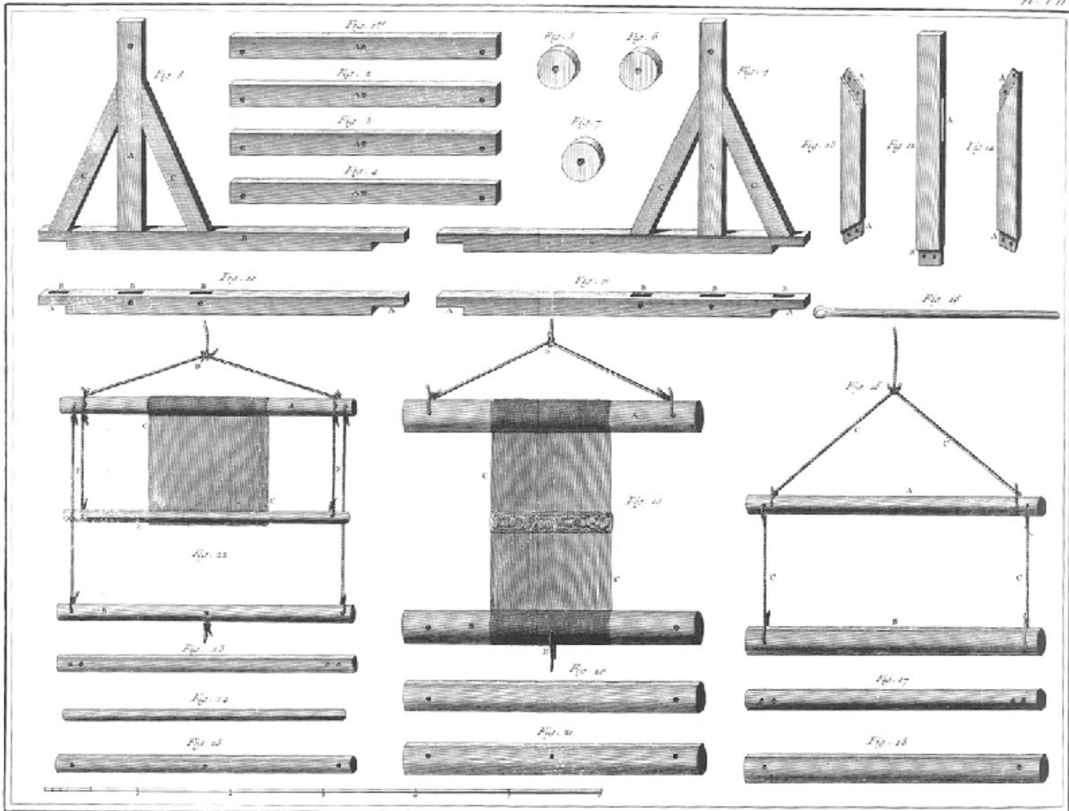
Détail des Pièces du Métier à Marli.
