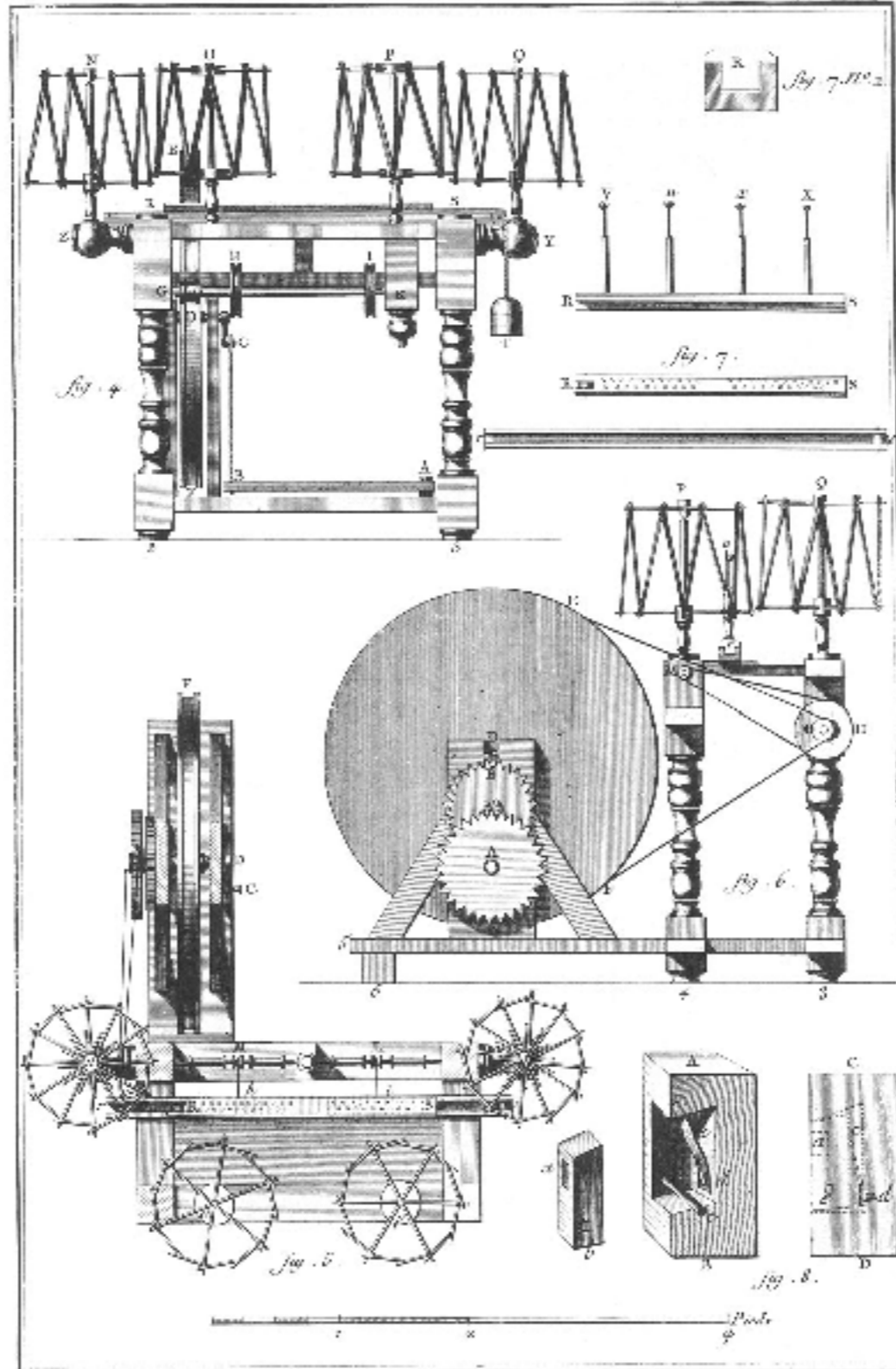
Soierie, Rouet de Lion, Développemens. Y
