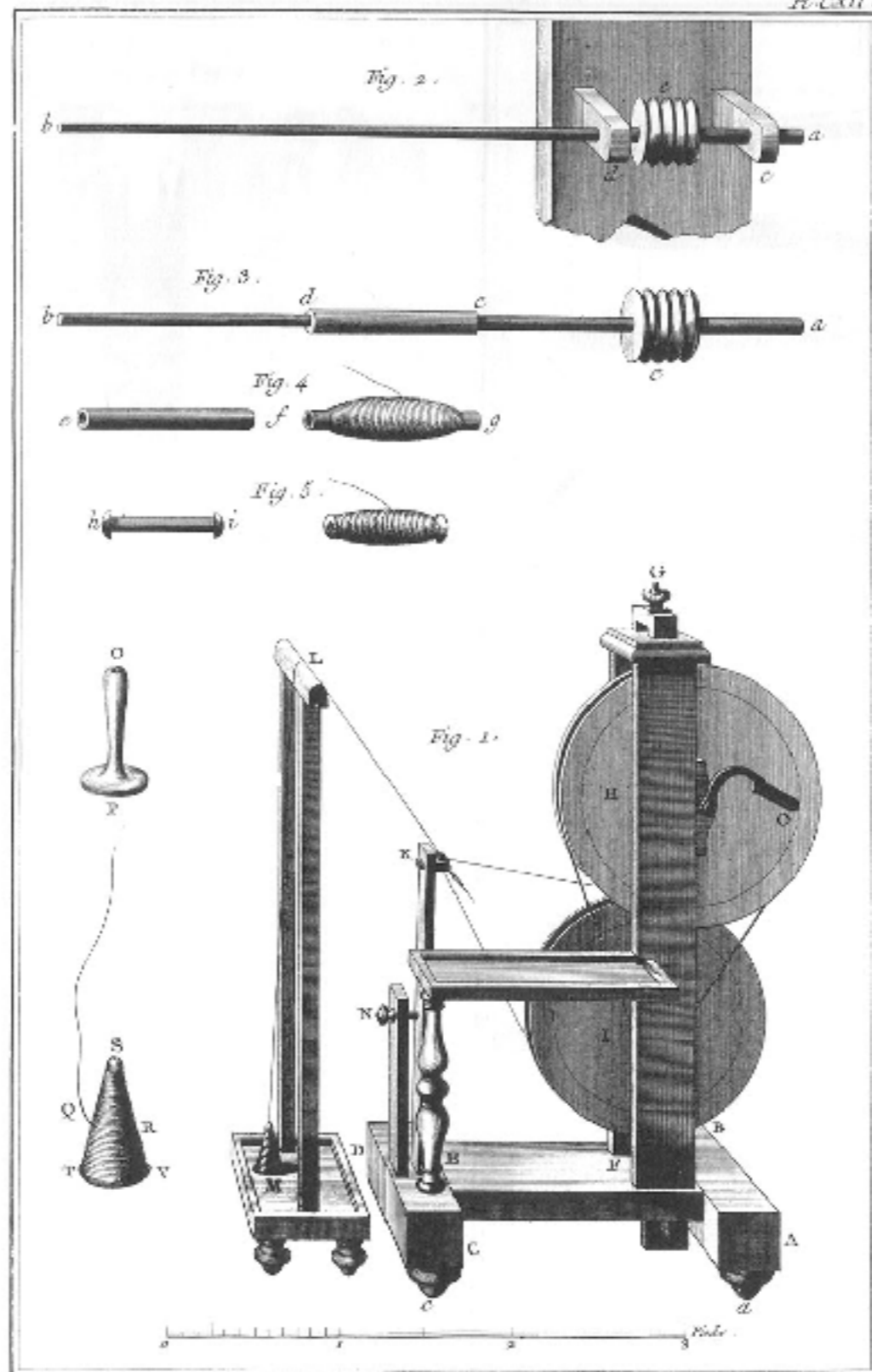
Soierie, Rouet à Cannelles
