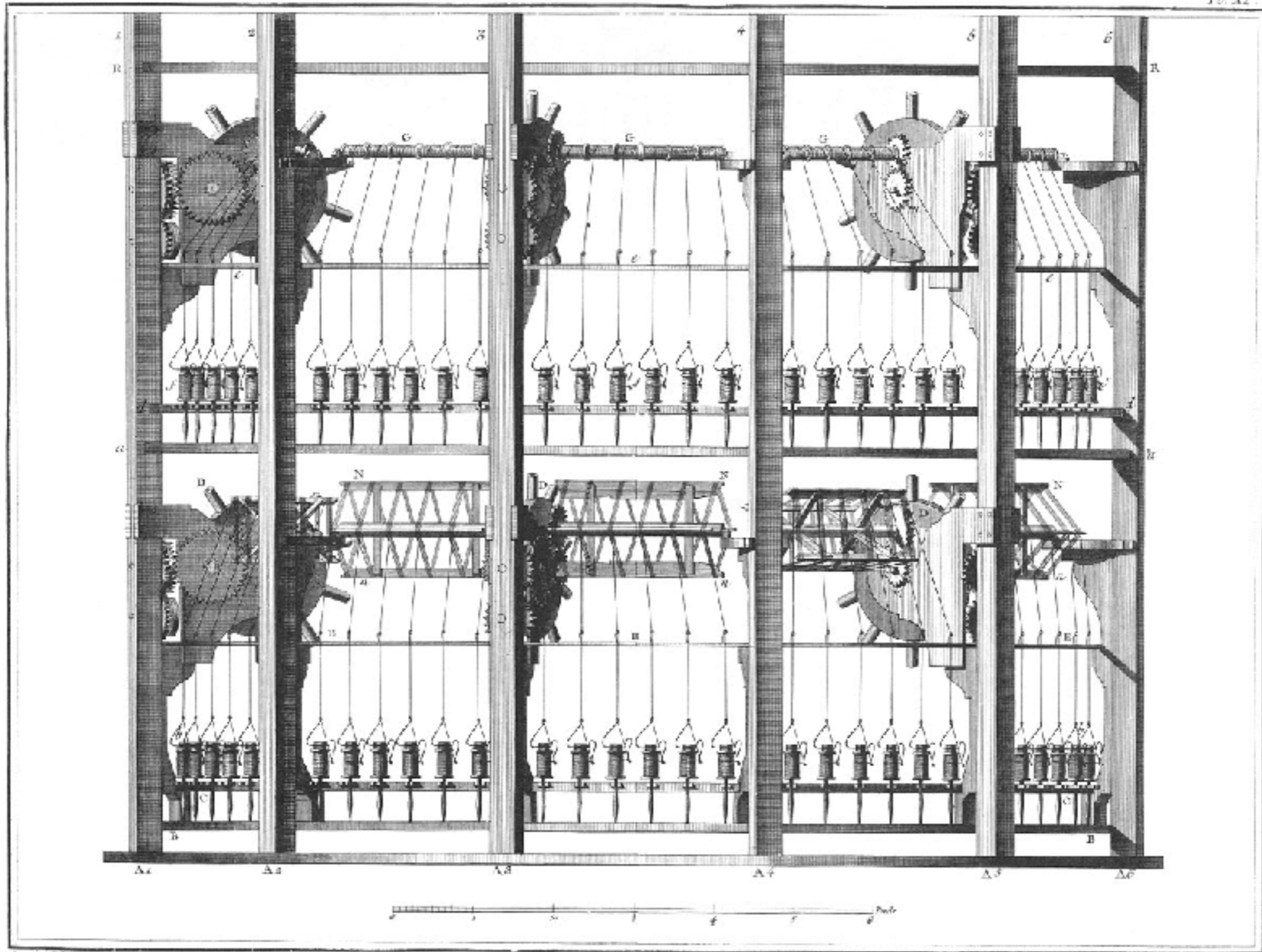
Soierie, Elevation Géométrale du Moulin de Prémont, pour Organiser les Soies.
