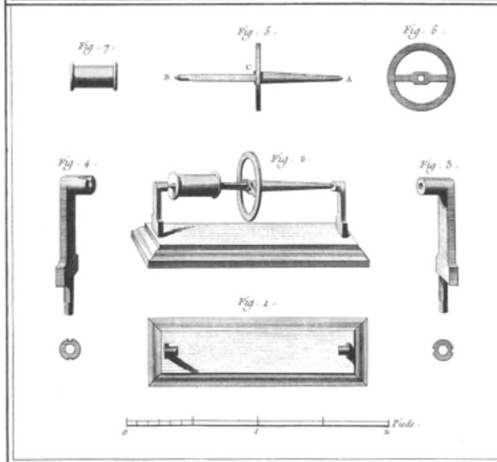
Soierie, névidage de la soie sur le Tour d'Espagne, Doublage et développement de l'Escaladou.
