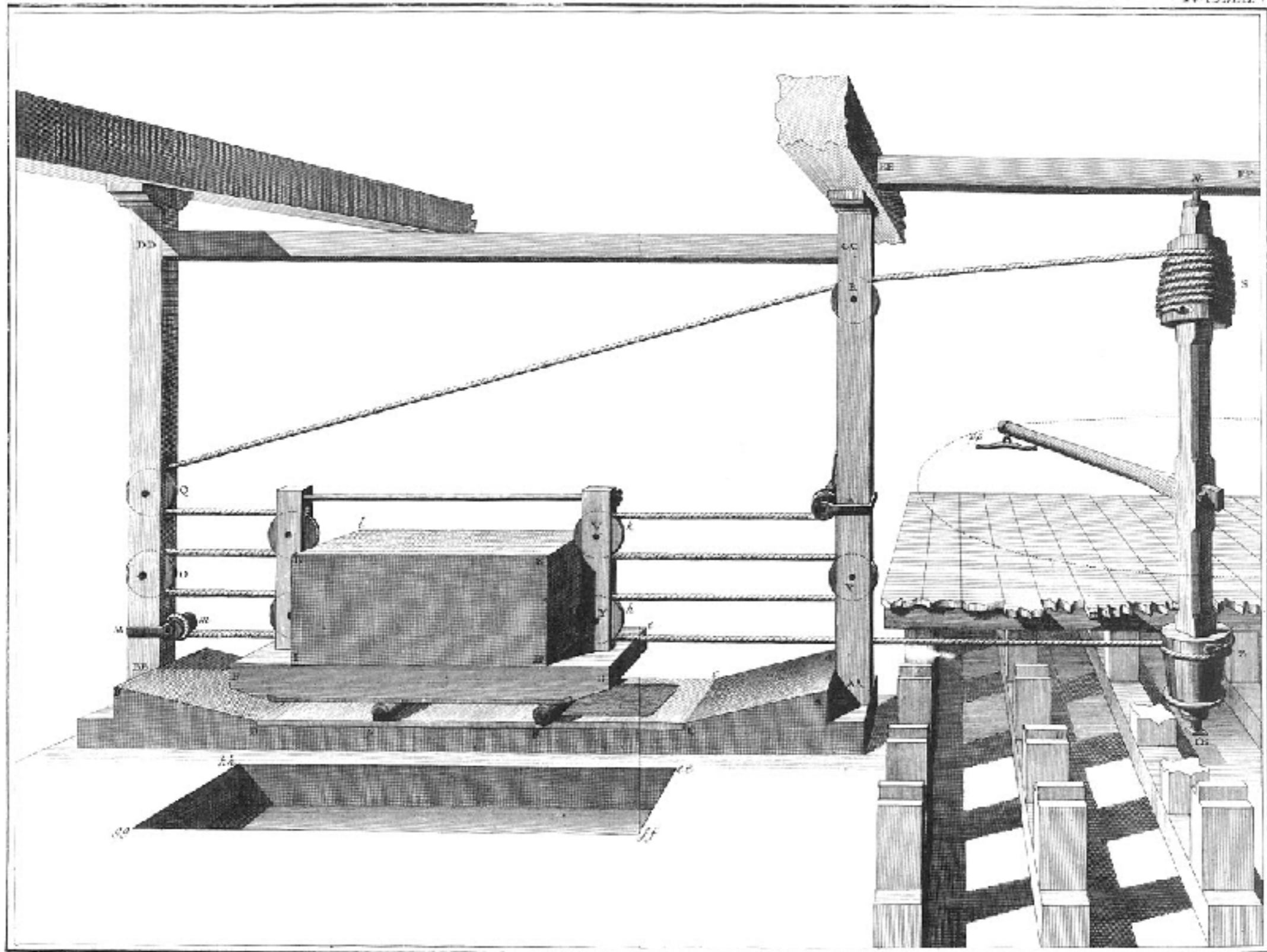
Soierie, Calandre Royale ou Calandre Angloise.
