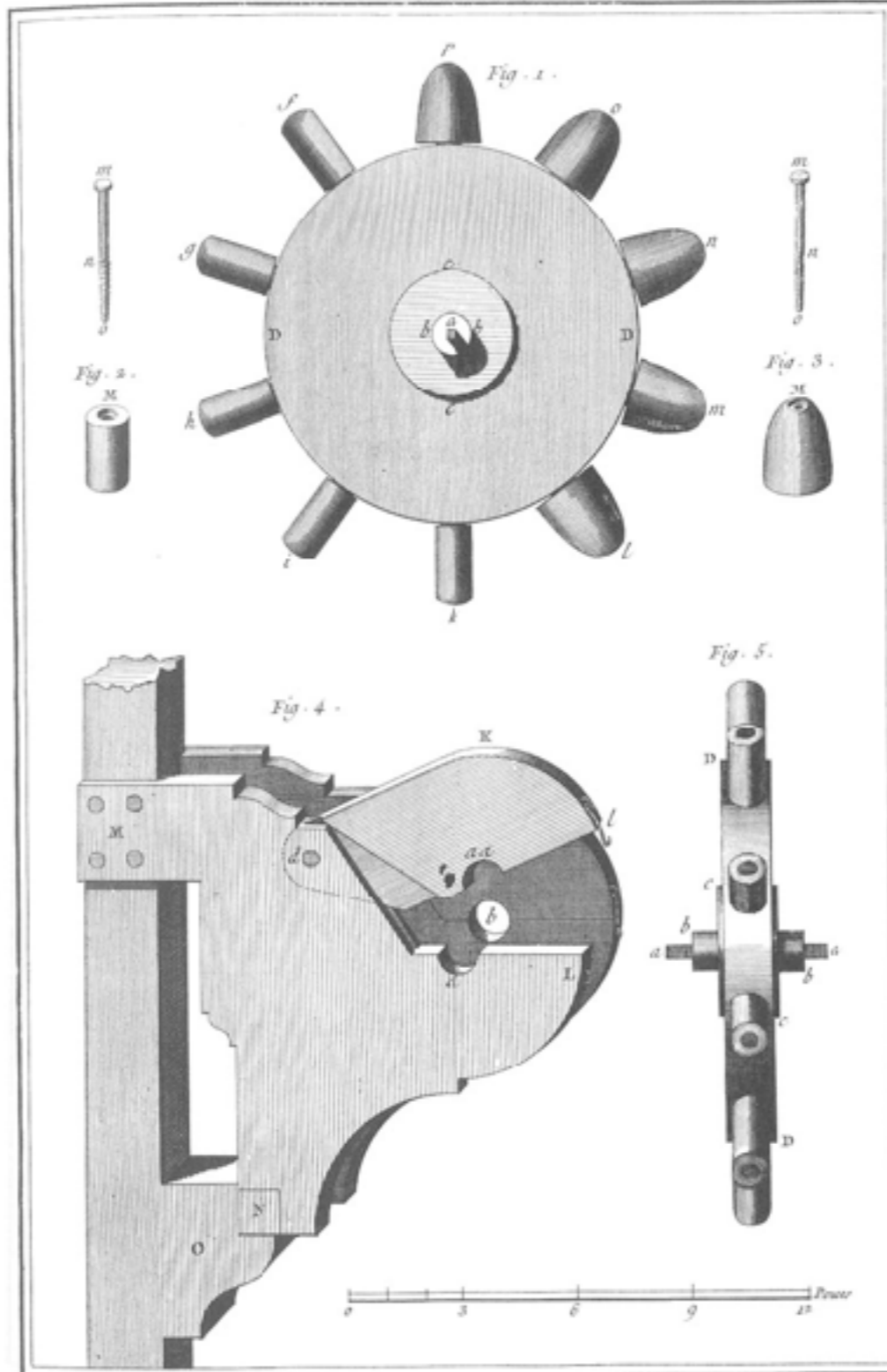
Soierie, Moulin de Piémont pour Organiser les Soies, Construction et Développement des Ponçonelles.
