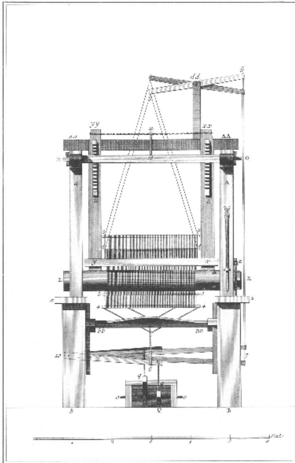
Soierie, Élévation Géométrale de la partie antérieure du métier pour fabriquer les étoffes unies, comme Taffetas, satin, et Serge. KK
