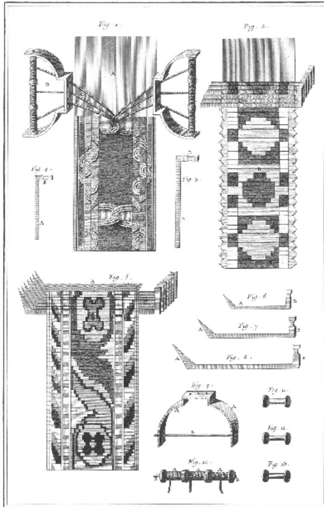
Passenterie, noueurs de Galons.
