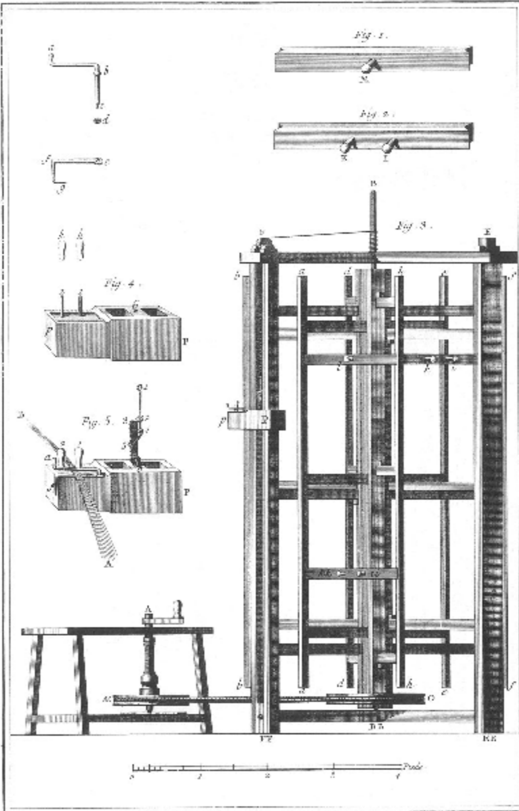
Soierie, Développement de l'ourdissage.
