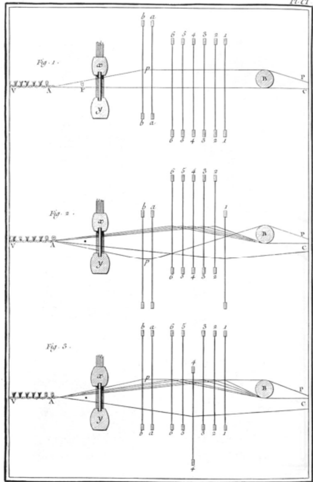
Soierie, Velours Coupé, iii 1 o Passage du Fer, 2 o premier Coup de Navette, 3 o second Coup de Navette.
