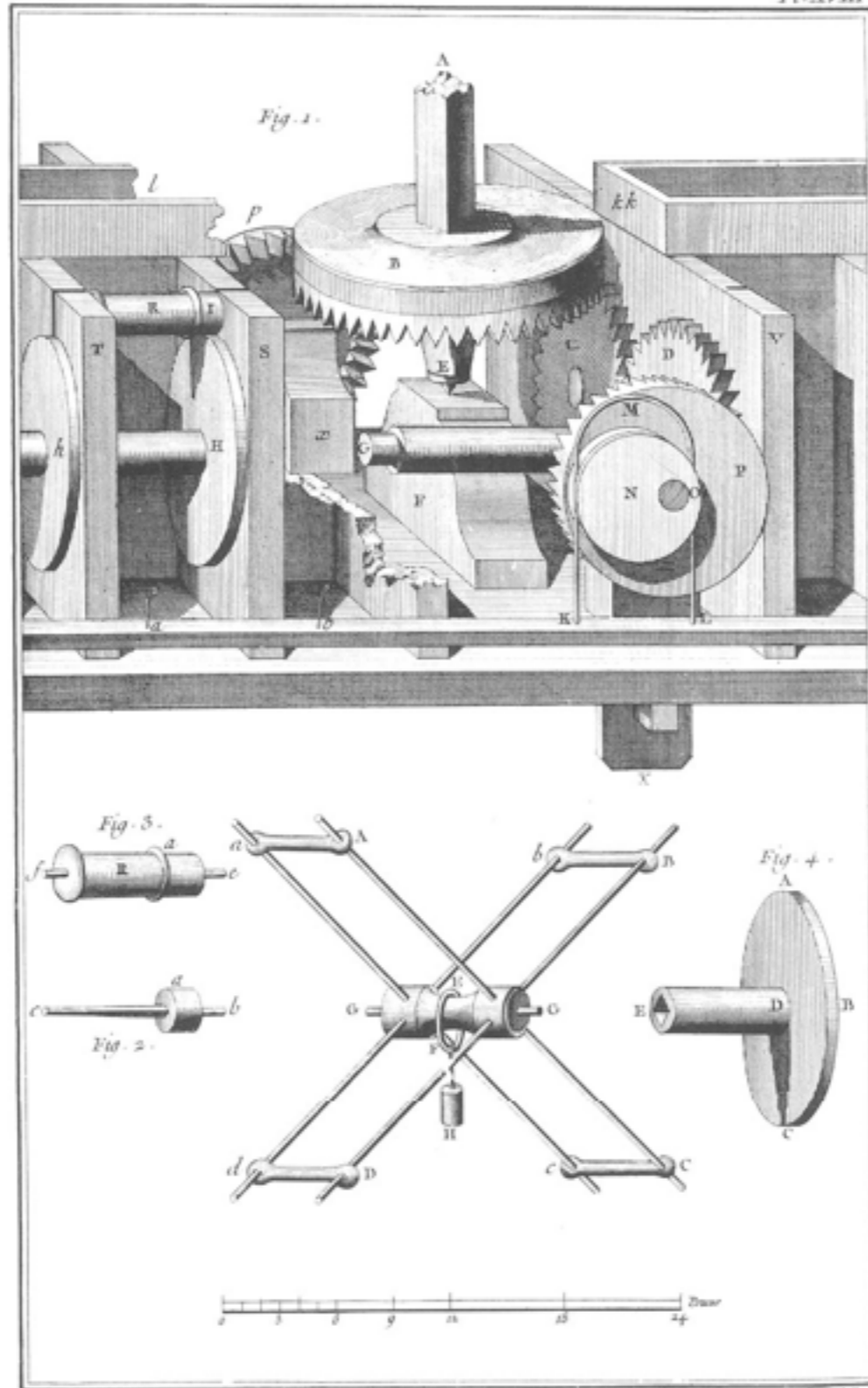
Soierie, Développement du Va - et - Vient du Devidage &c. S
