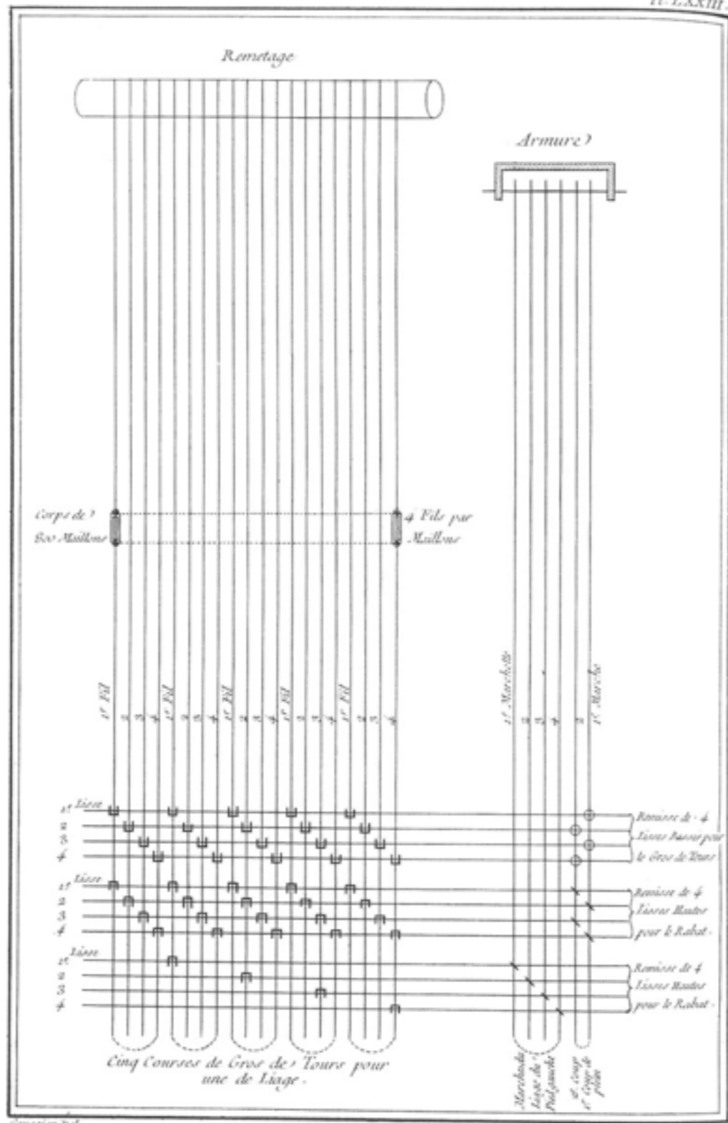
Soierie , Gros de Tours Broché avec un Liège de 4 le 5. dd
