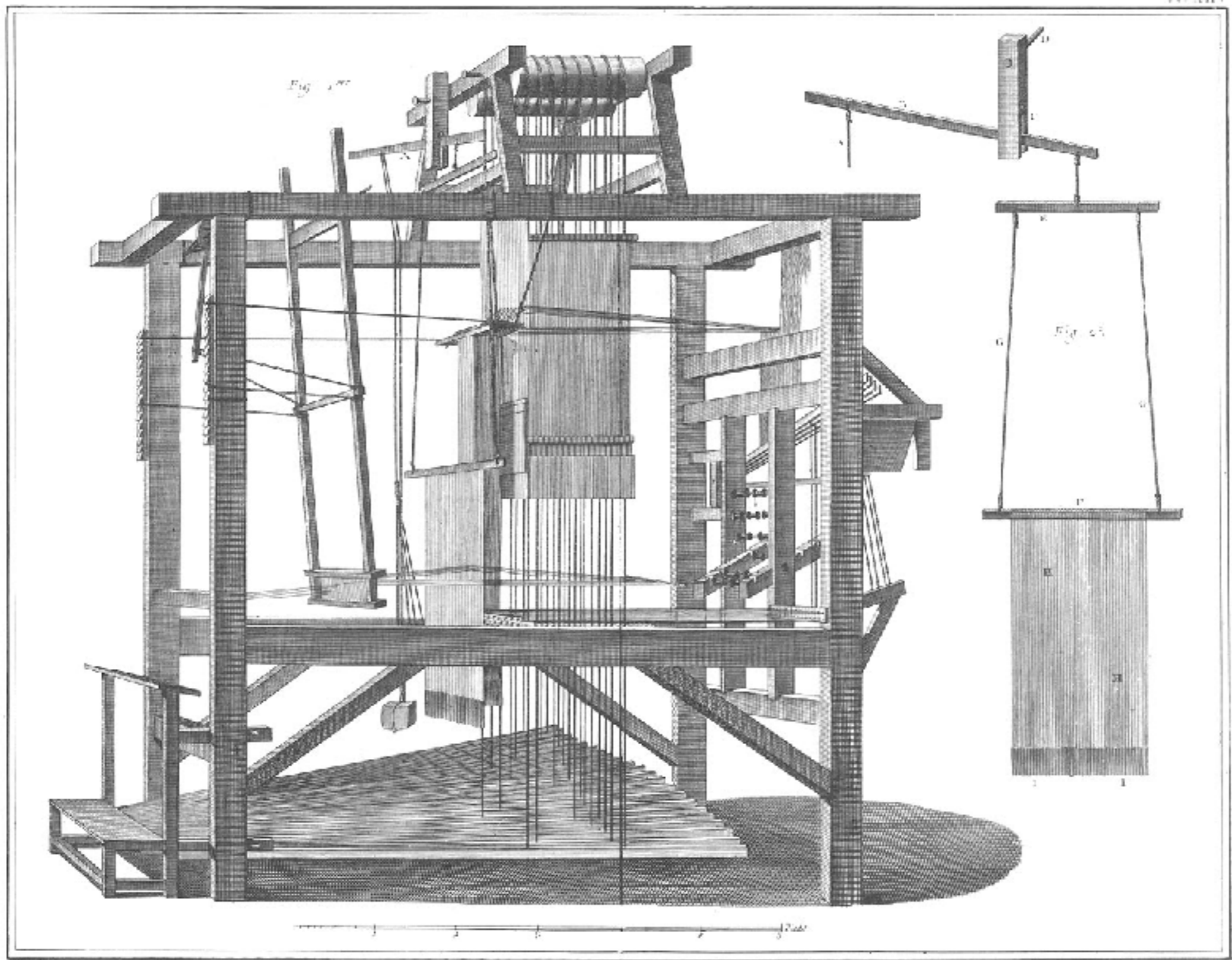
Passementerie, Matic du Ruban figure.
