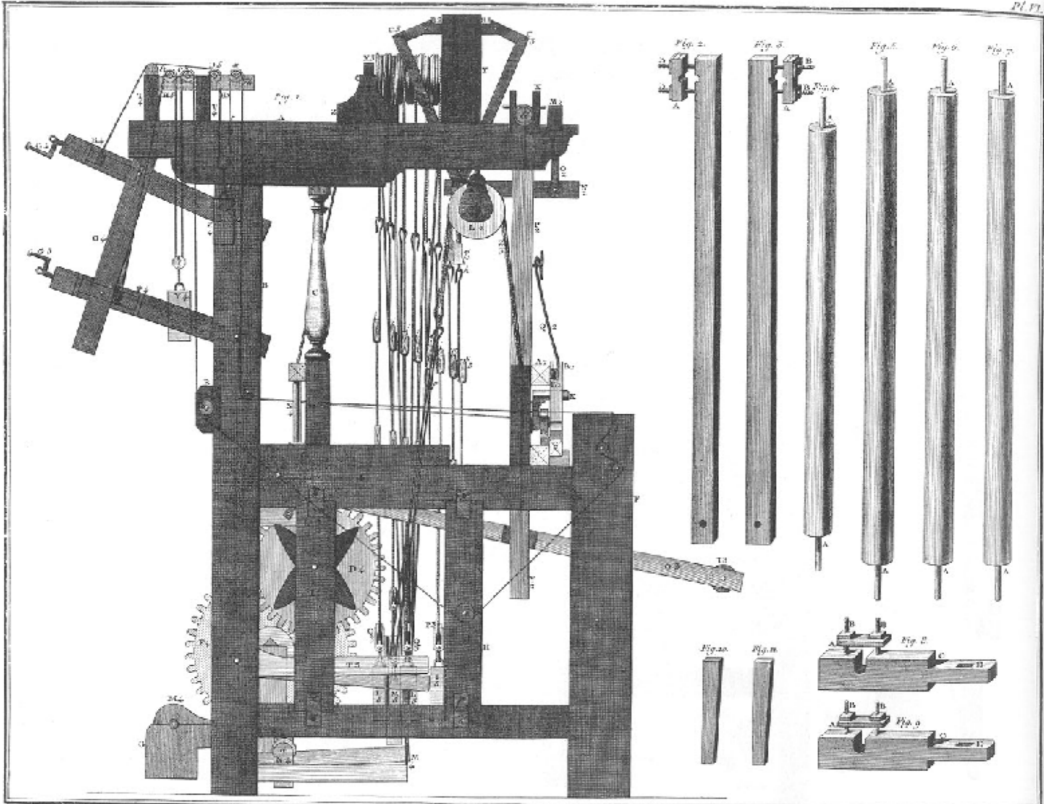
Métier à faire le Ruban, fabrication latérale.
