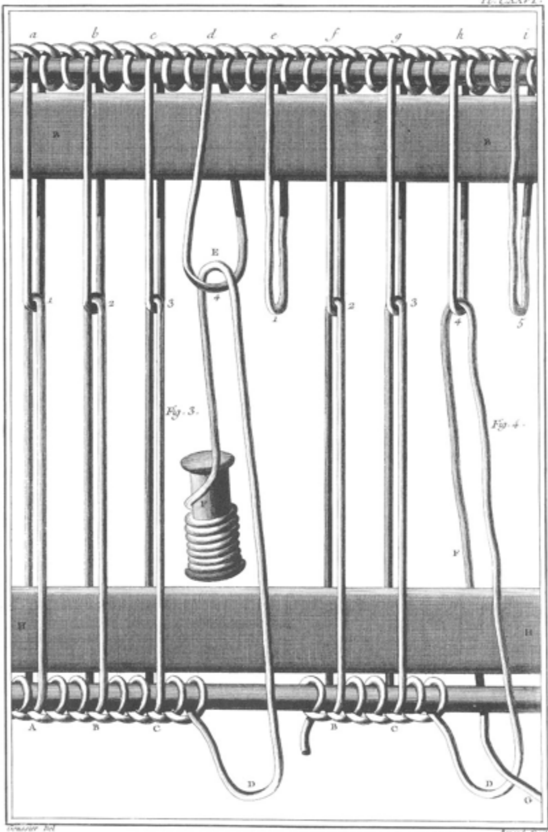
Soierie Tissus à Crochets ; premier et second temps de la formation de la Maille . IIII
