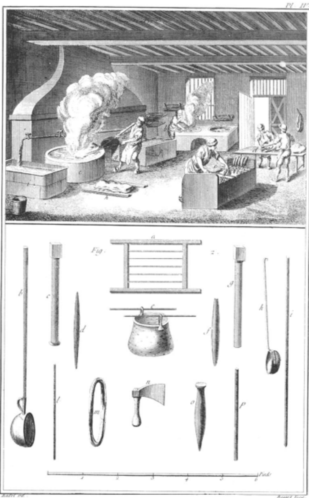
Teinturier, atelier et Outils.
