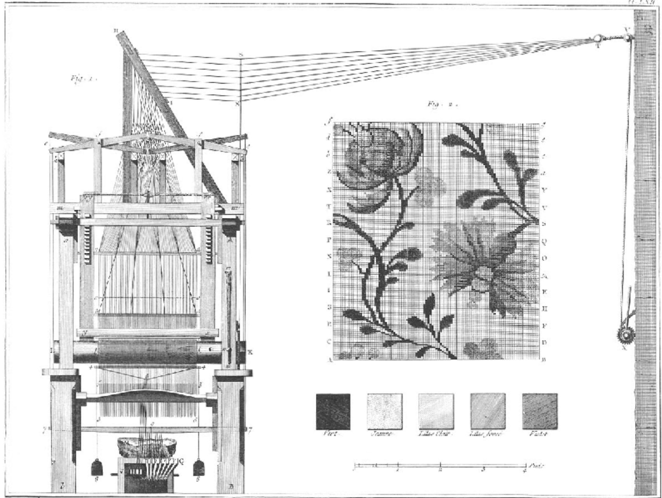
Soierie, Étoffes Brochées, Élévation Géométrale du devant du Méier pour fabriquer les Étoffes Brochées.
