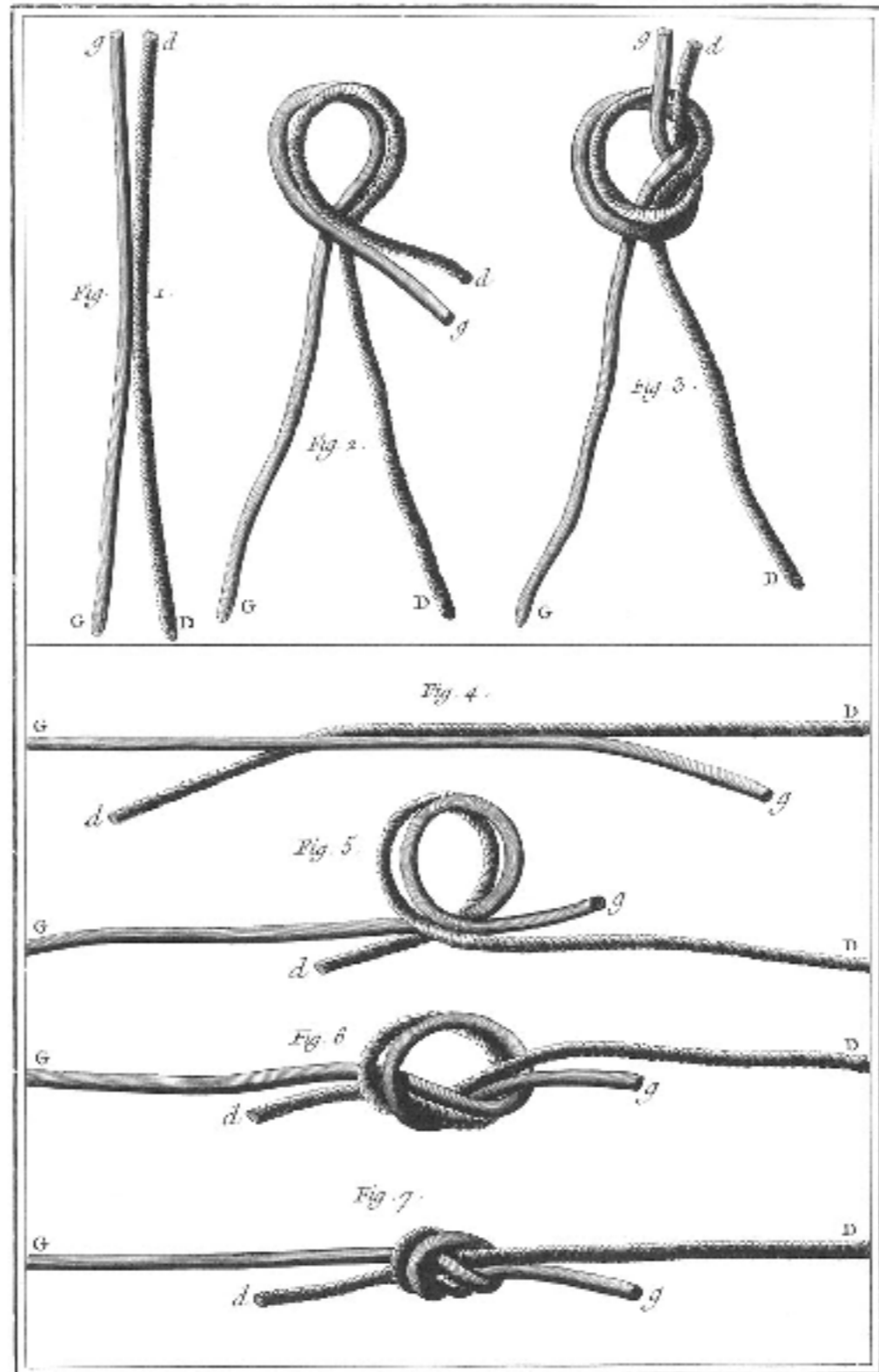
Soierie, nœuds à petites queues et à grandes queues. les différens temps de leur formation.
