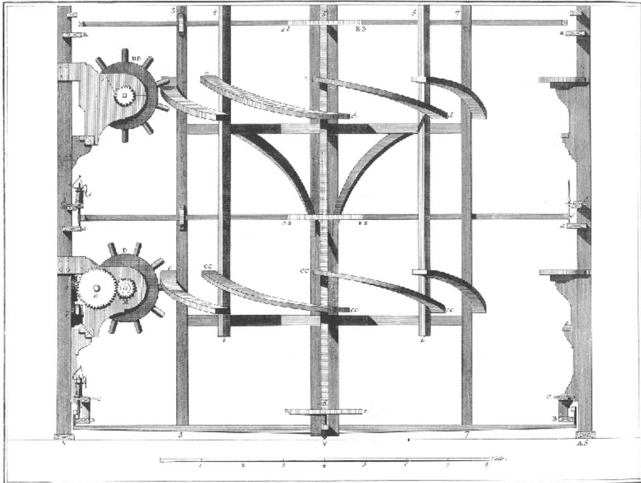
Soierie, Coupe Diamétrale du Moulin de Fismont et Élévation de la Lanterne qui est dans l'Intérieur.
