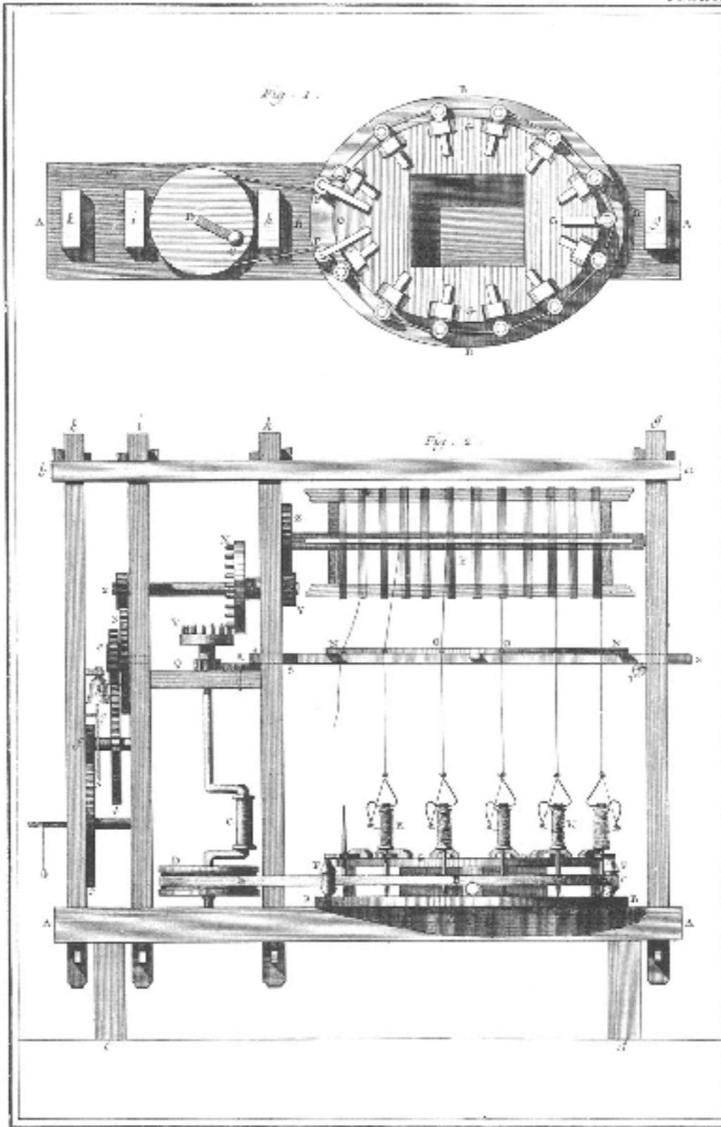
Soierie, Ovale Plan et Elevation.
