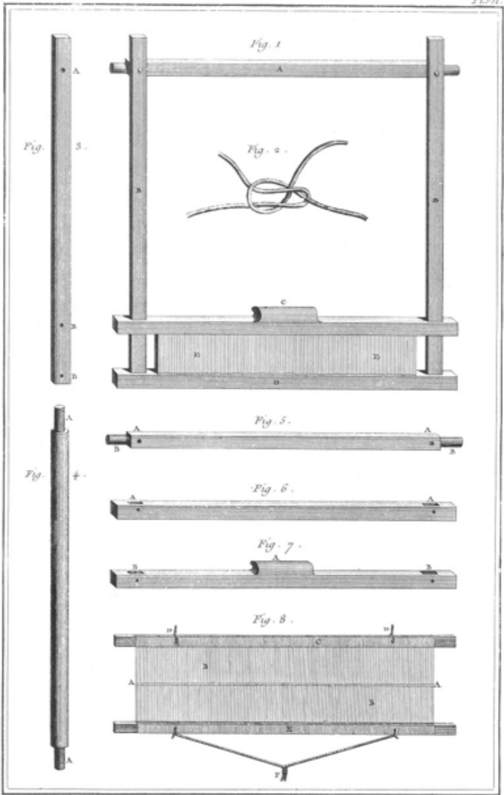
Tisserand, Détails du Métier à faire la Toile.
