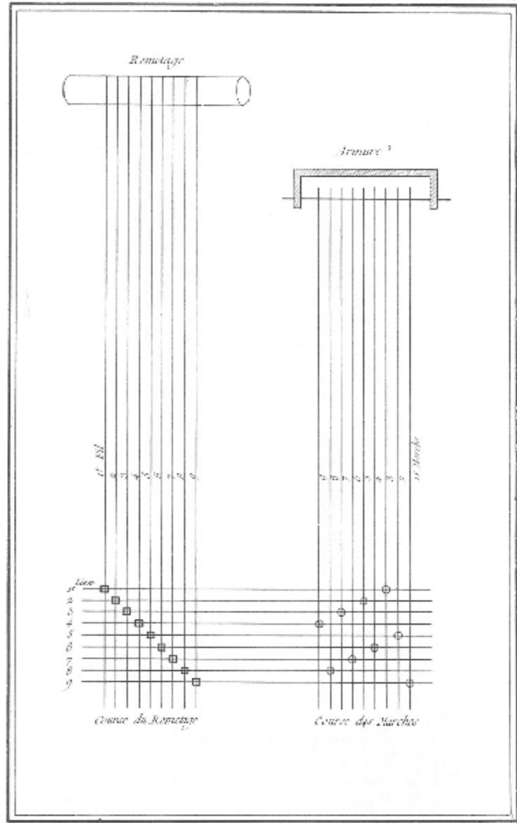
Soierie, satin à 9 Lisses. b
