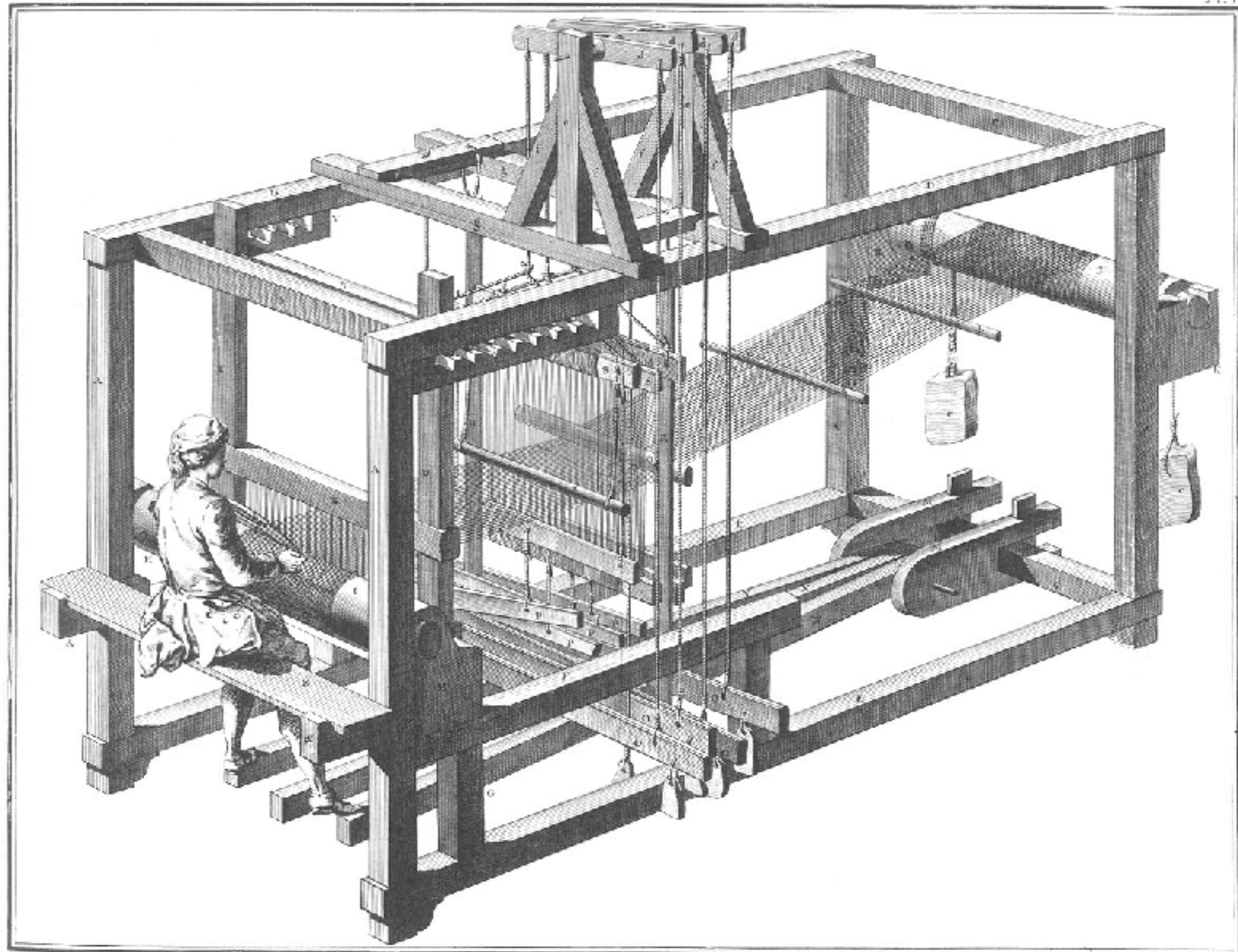
Mètier à Marly.
