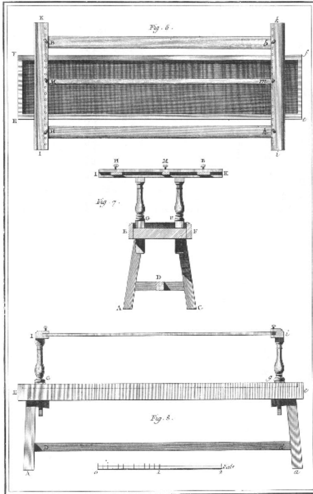
Soierie, développemens du Lassoir.
