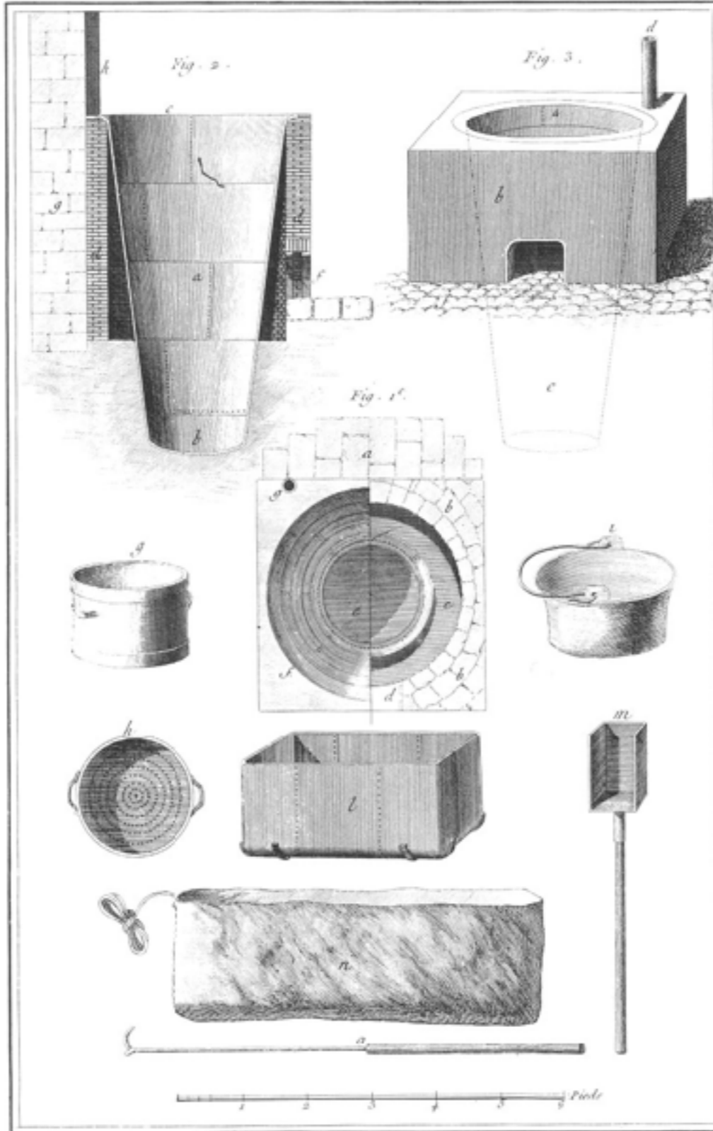
Teinturier de Riviere, Plans, Coupe et Élévation de la Cuve pour l'Indigo.
