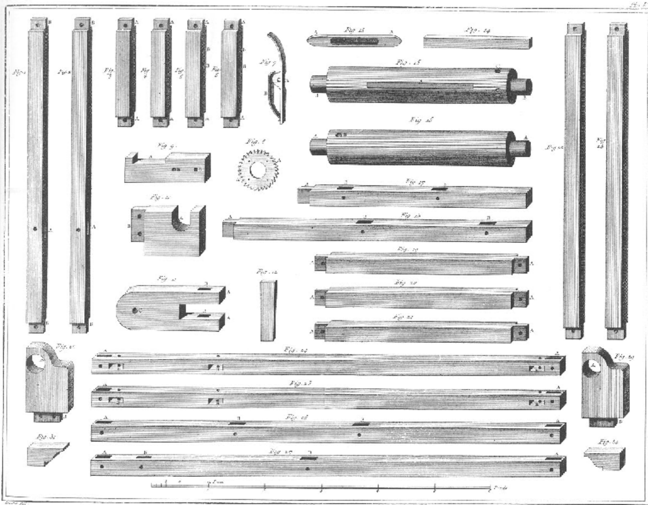
Détail des Pièces du Métier à Marly.
