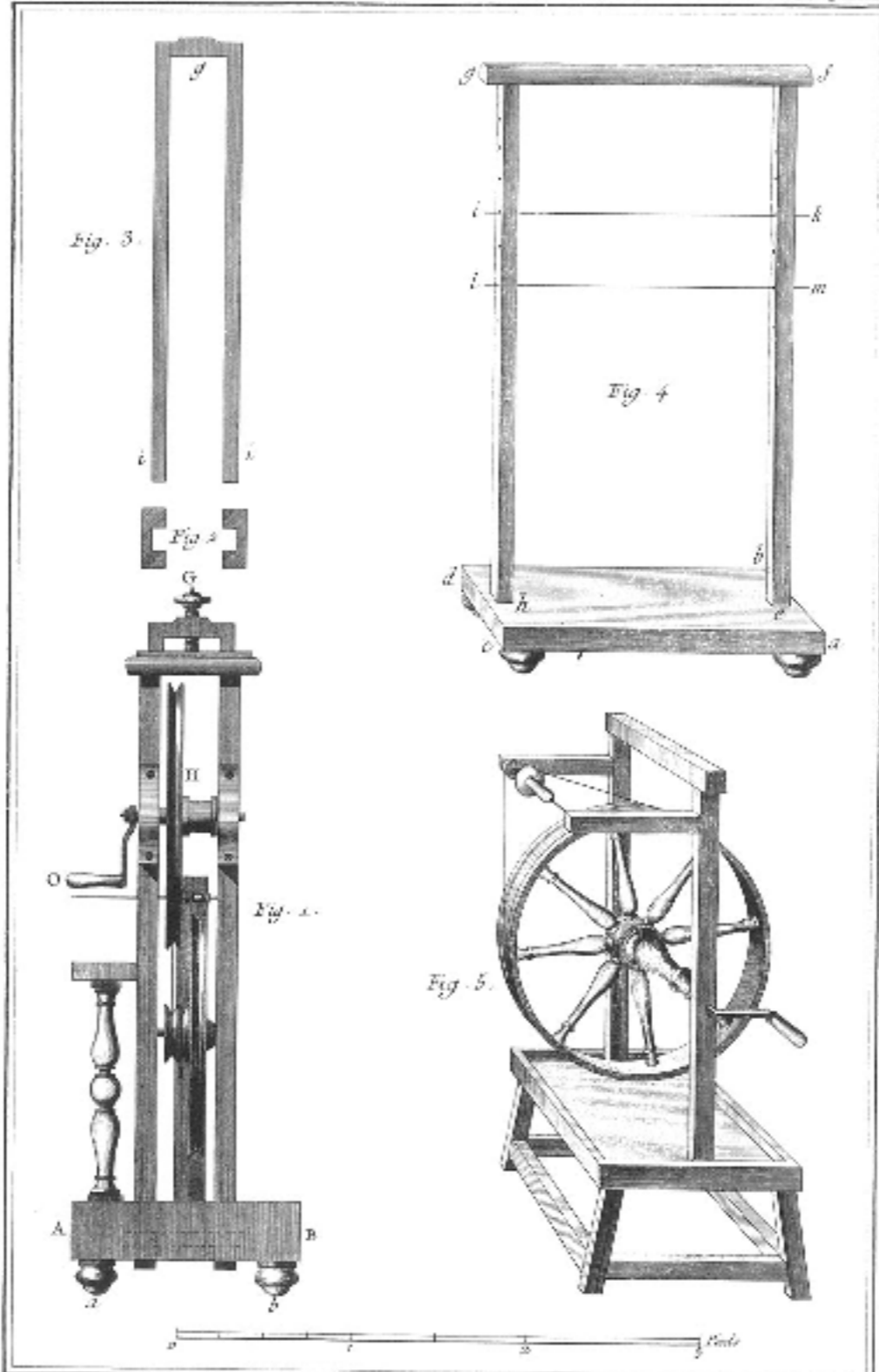
Soierie, Développemens du Rouet à Canettes et le Rouet servant à garnir les Tôlans.
