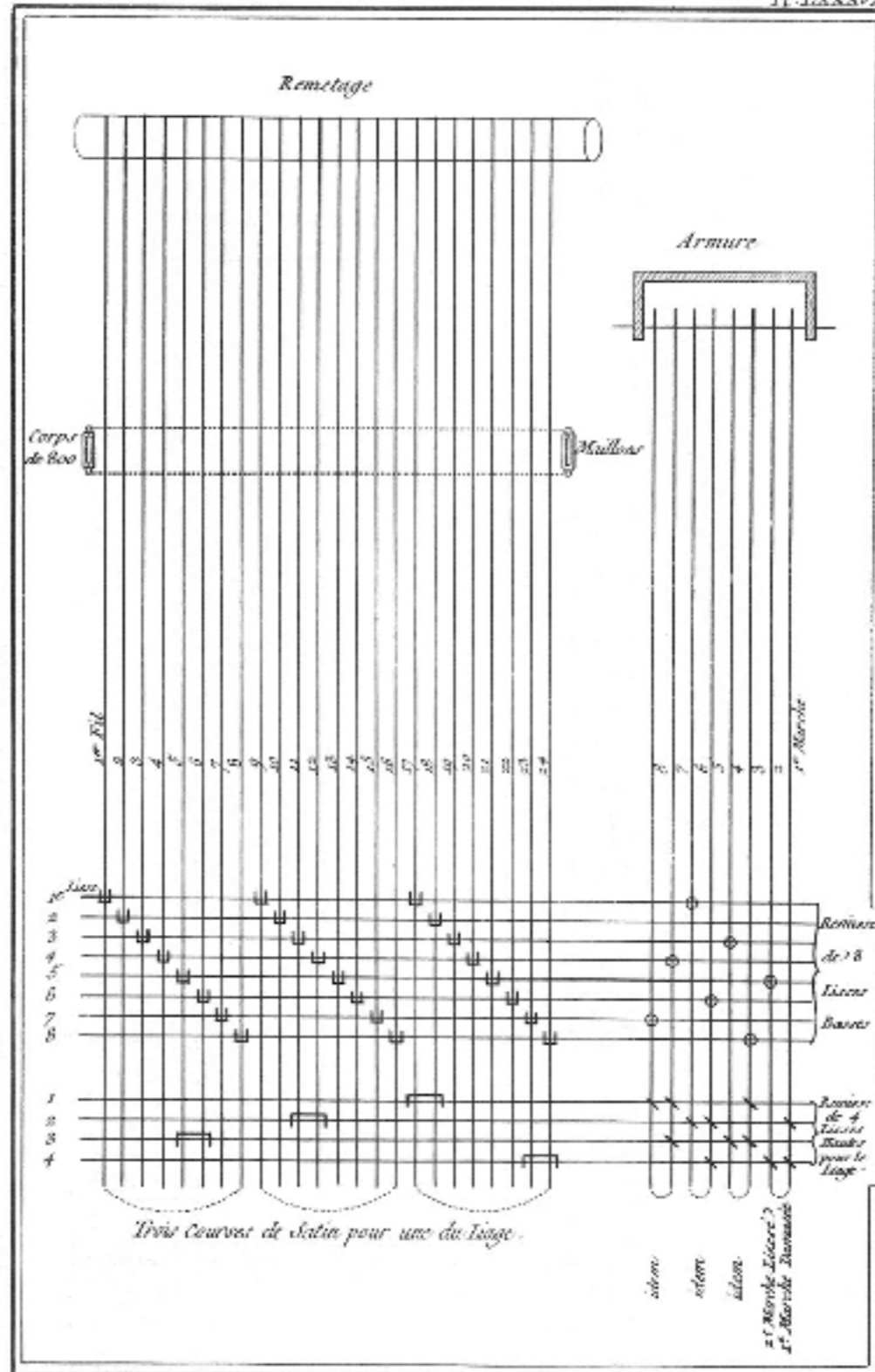
Soierie, Florentine Damassée avec un Lixier et un Linge.
