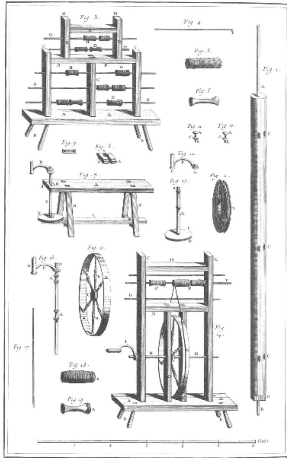
Passementerie, Ourdissoir, Banque d. Rouet.
