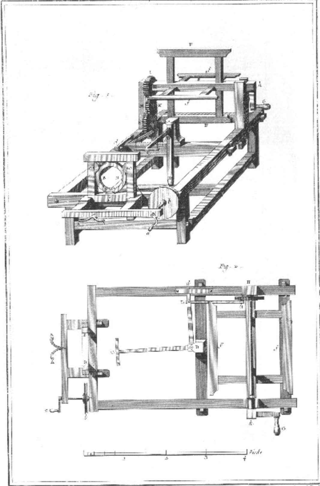
Soierie, Tour de M. de Vaumason.
