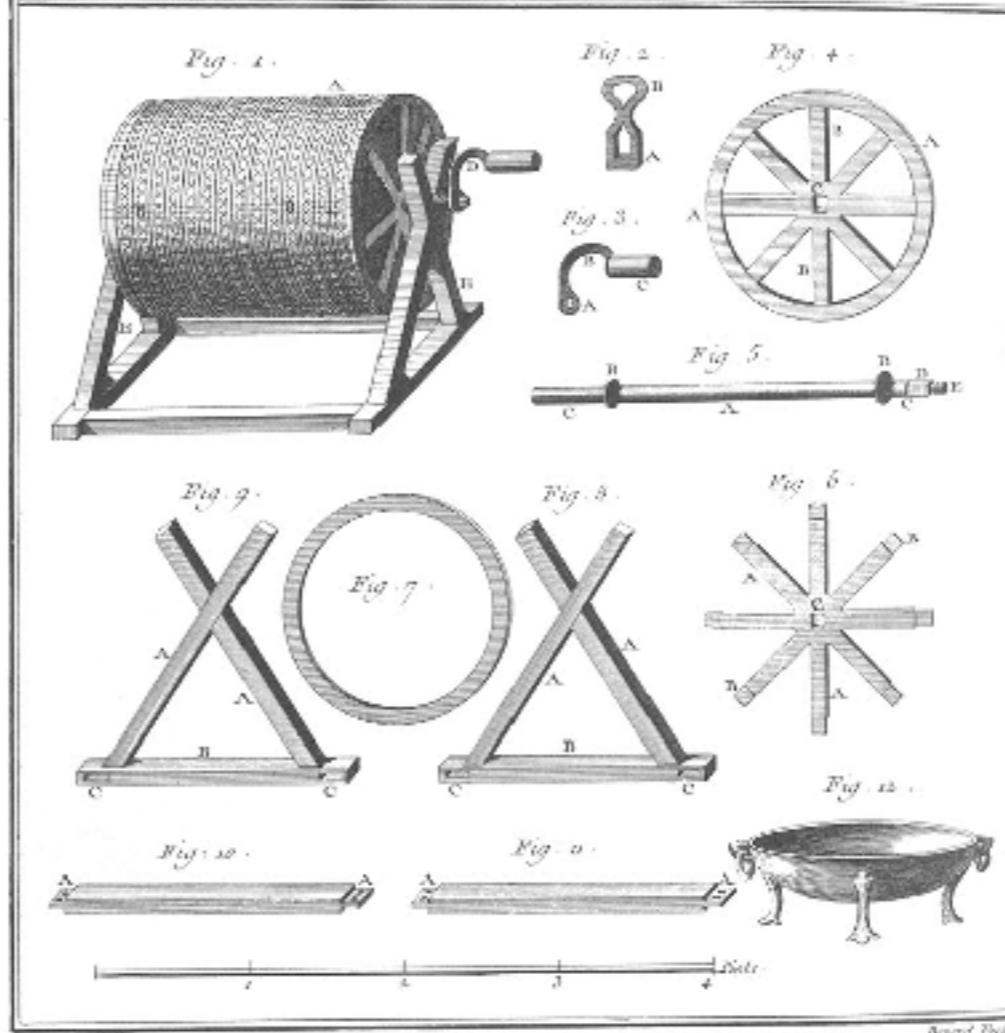
Passenterie, Fumage du Galon ?
