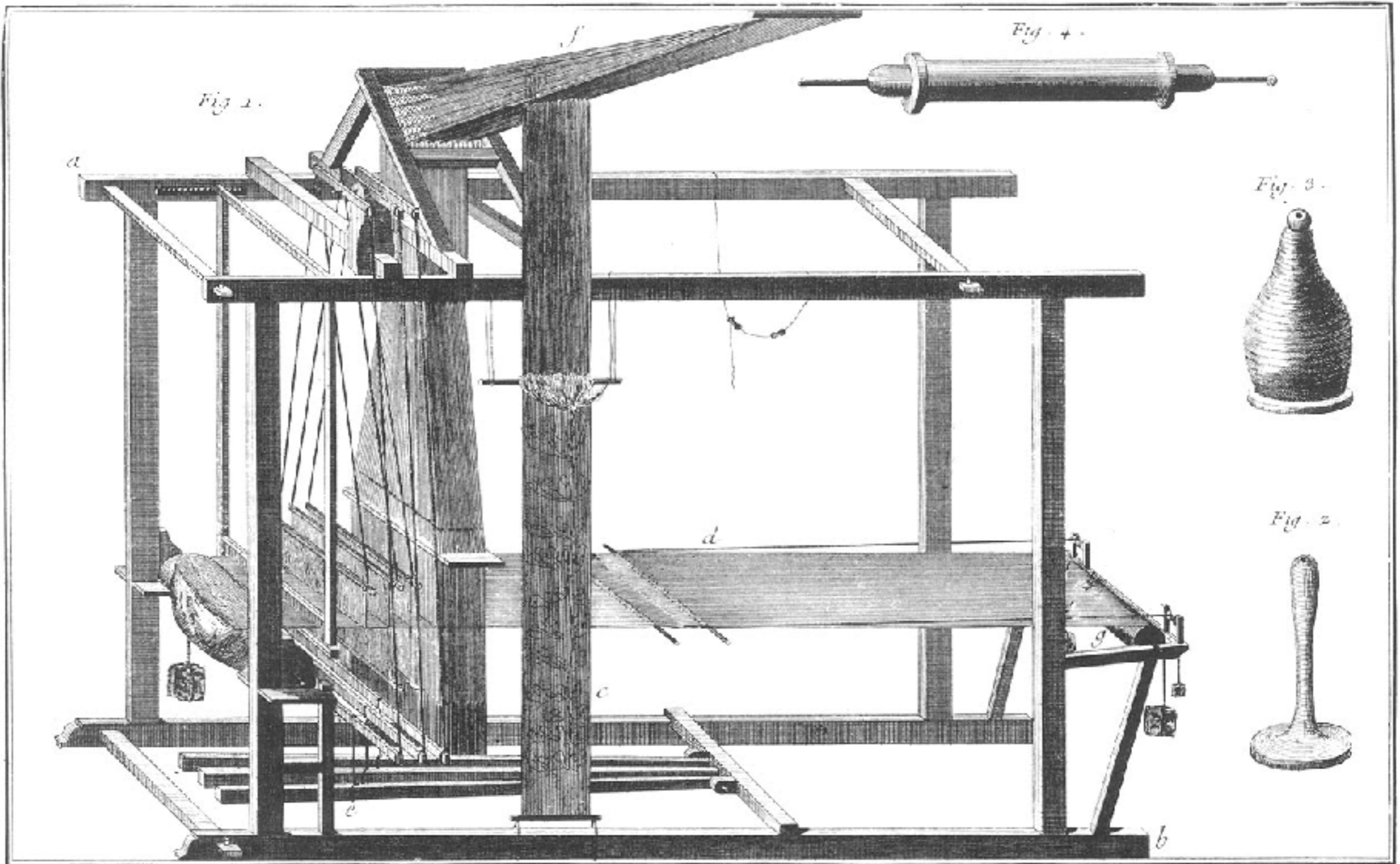
Gazier, Métier à Gaze vu sur la longueur et Détails.
