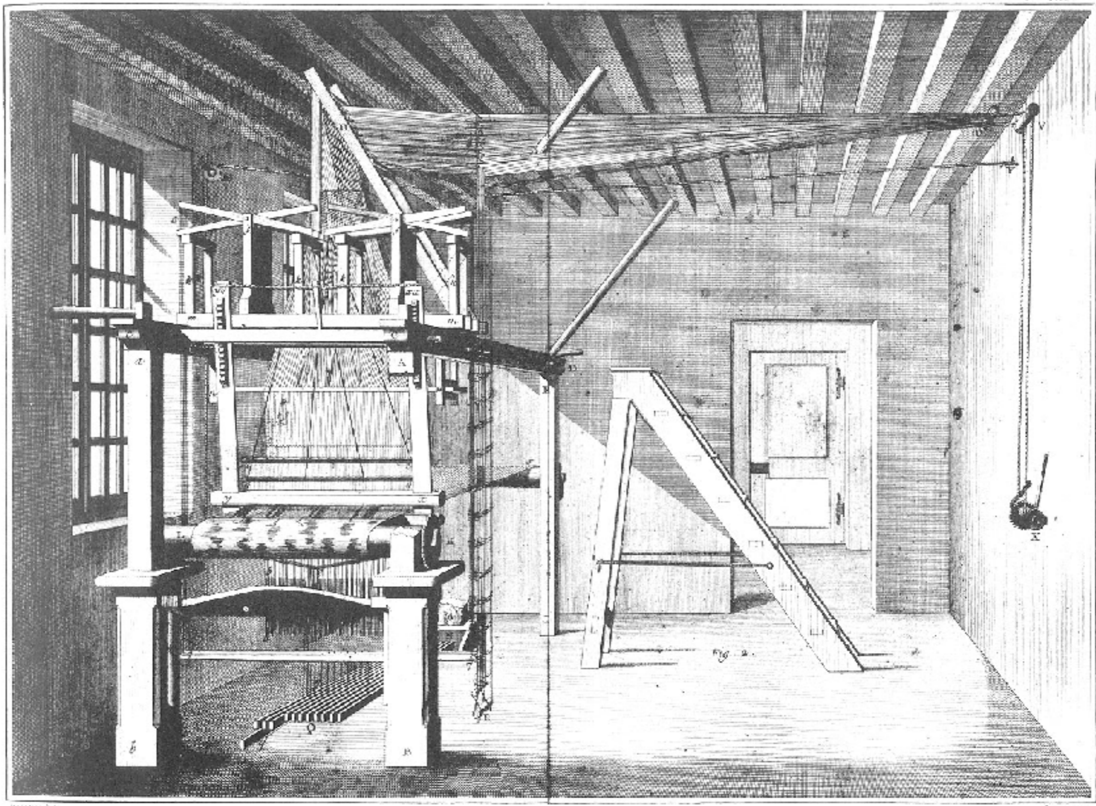
Soierie, Truffes Brochées élévation Perspective du Méier pour filer que les Truffes Brochées garni de tous les cylindres et autres
