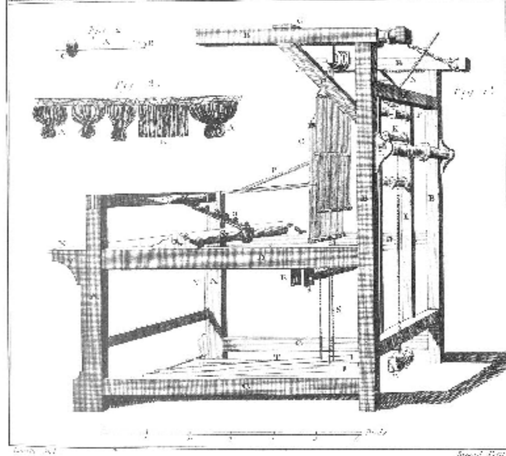
Passementerie, Machine à Passer.
