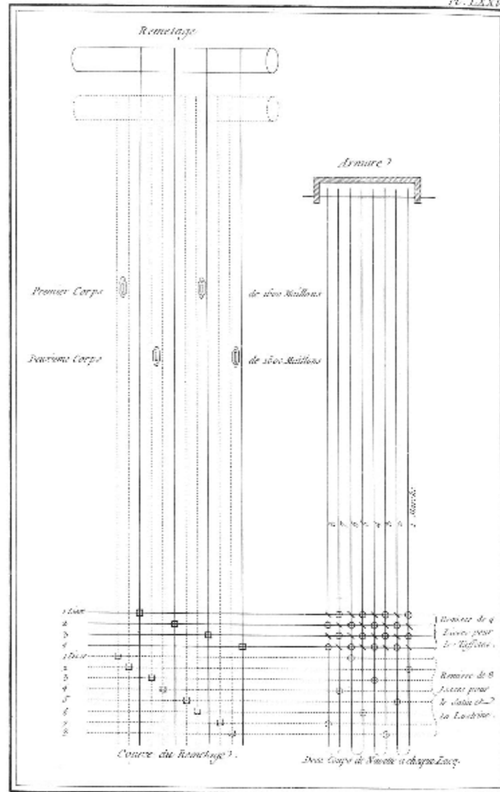
Soierie, Drognet Lustriné Double Corps.
