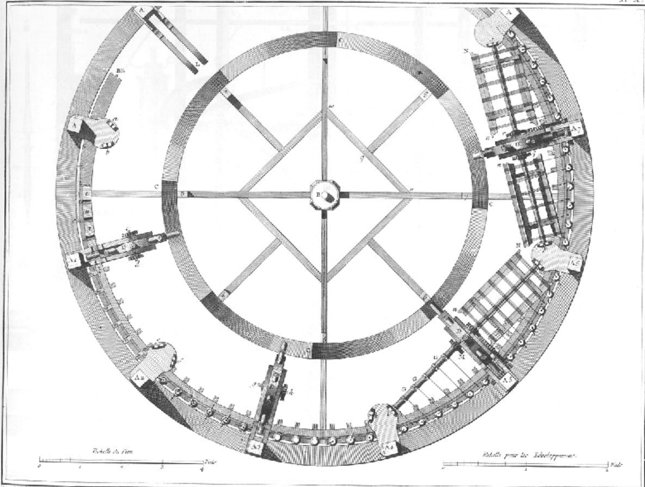
Soierie, Plan du Moulin de Piémont, à Strafine pour Organiser les Soies.
