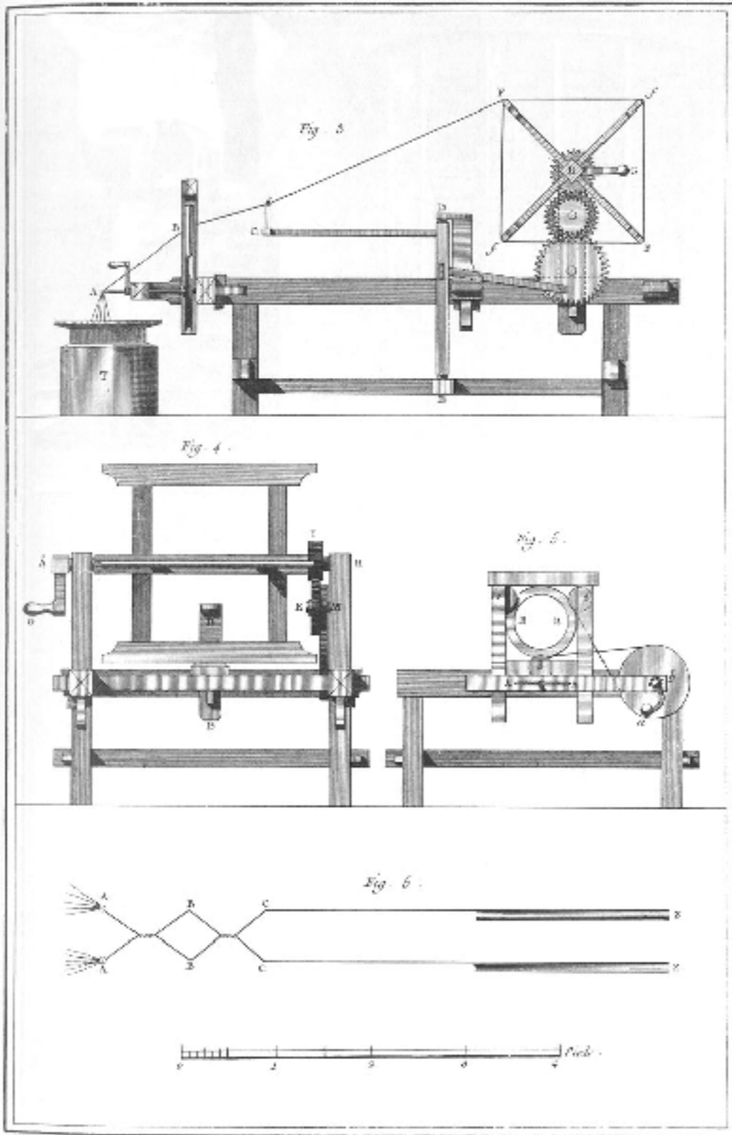
Soierie, Developpemens du Tour de M r de Vaucanson
