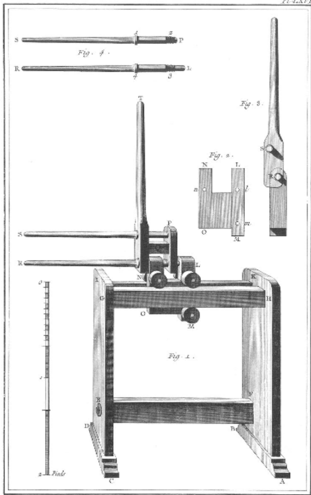
Soierie, construction de la Machine pour la Tire. W
