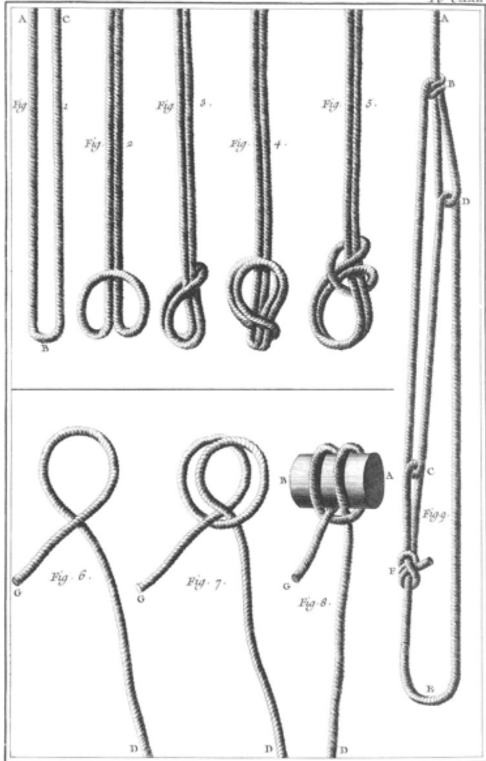
Soierie , Noeud de Sangle et de Rame ou à double Boucle, Noeud de la Charrue, Noeud à Crémaillère. les différens temps de leur formation. 9999
