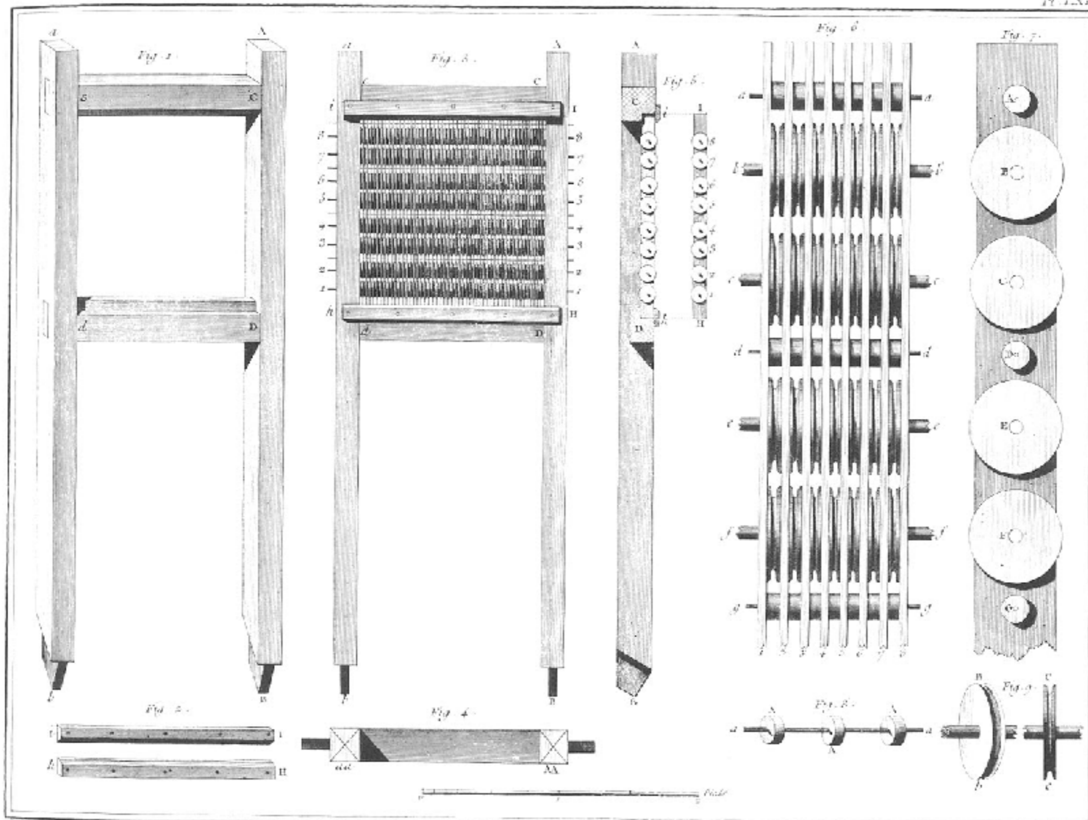
Soierie, Étoffe Brochiée, Élévation et Développement du Cassin.
