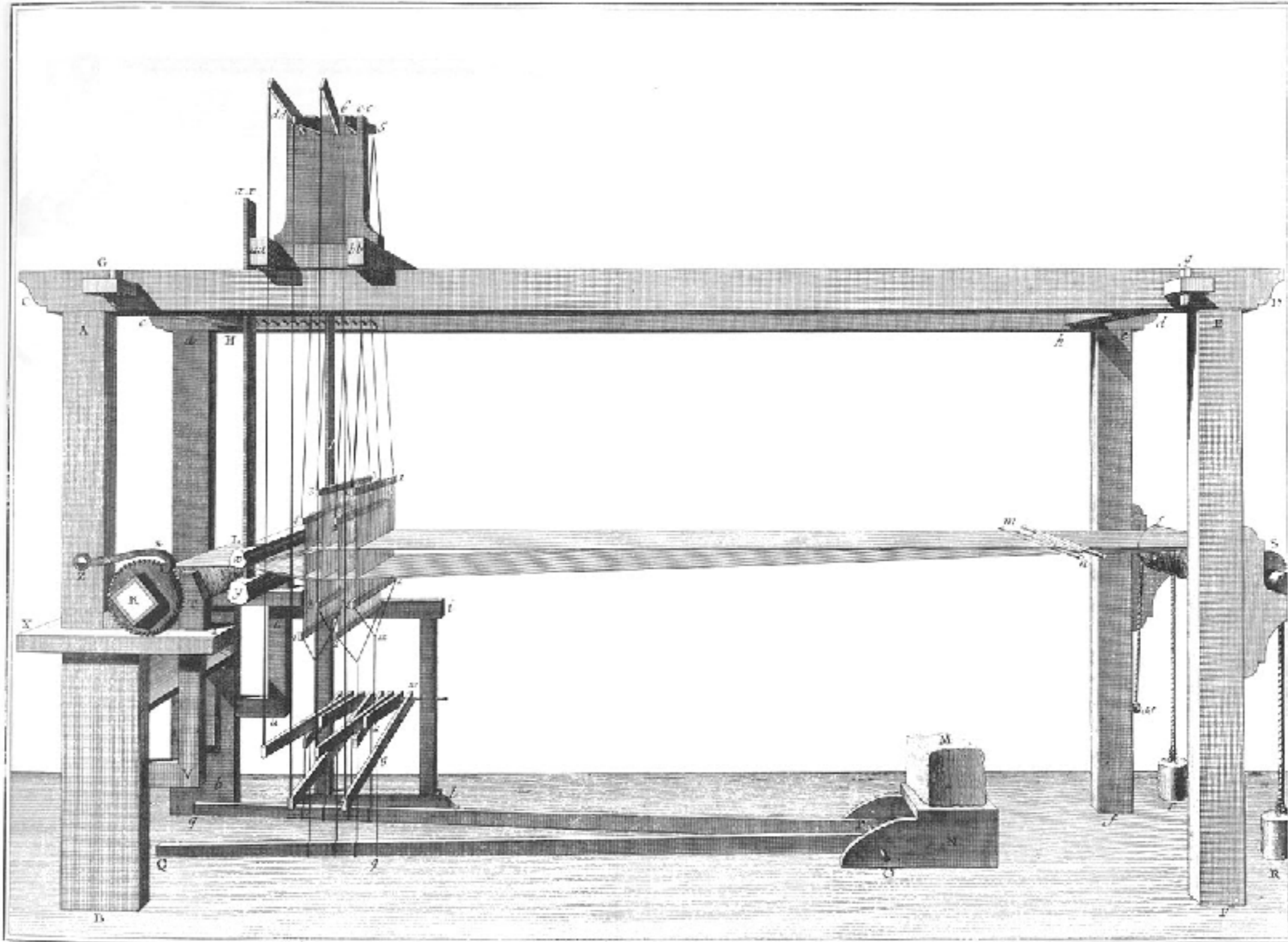
Soierie, Vue Perspective du métier pour fabriquer les Étoffes unies. Comme Taffetas, Satin et Serge, la chaîne ouverte au premier coup du Taffetas. HH
