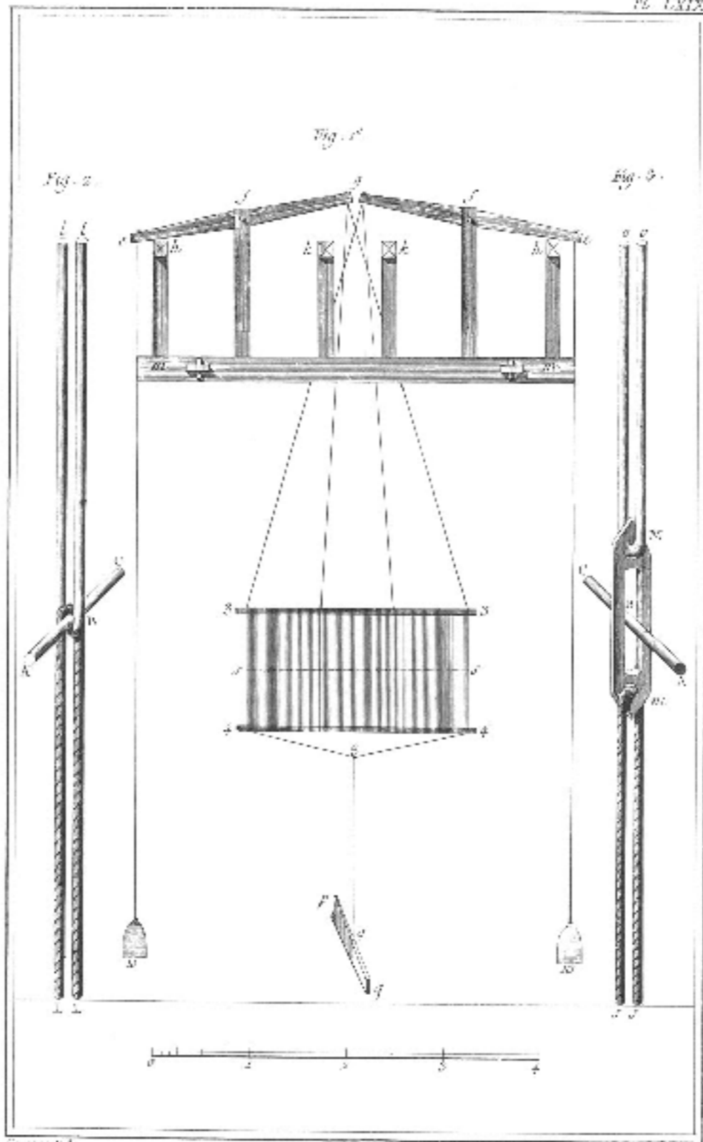
Soierie, Stoffes Brochés. Développement des Trains de Laine.
