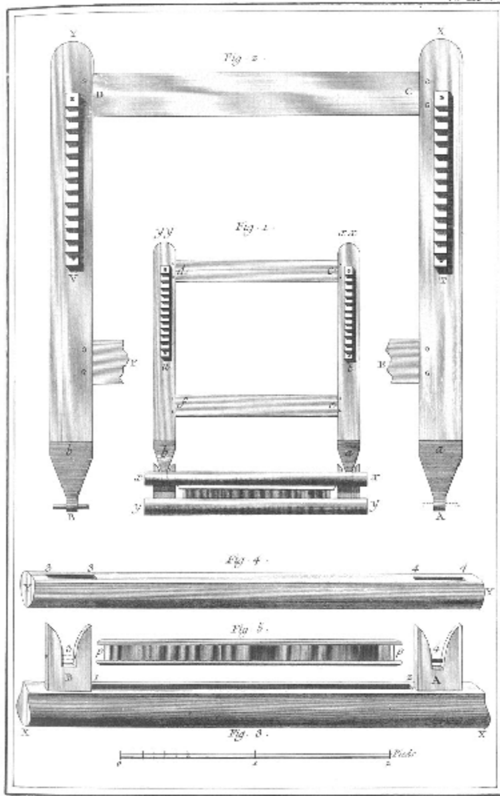
Soierie. Velours, Développement du Battant brisé du Métier à Velours. bbb
