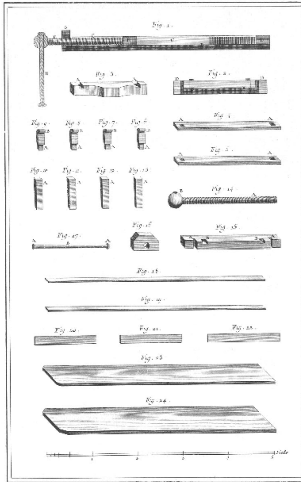
Passementerie; D e tail de la Machine à monter les Triguans à la manière Angloise.
