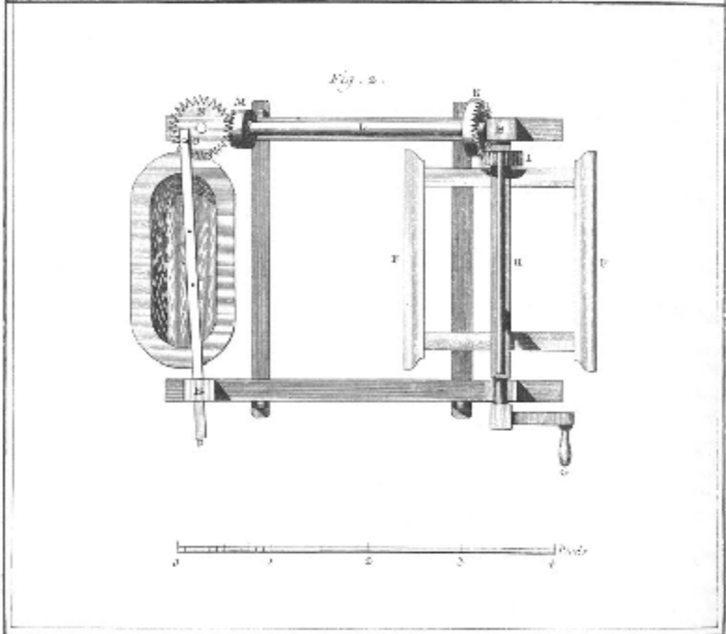
Soierie, Tirage de la Soie et Plan du Tour de Piemont. A
