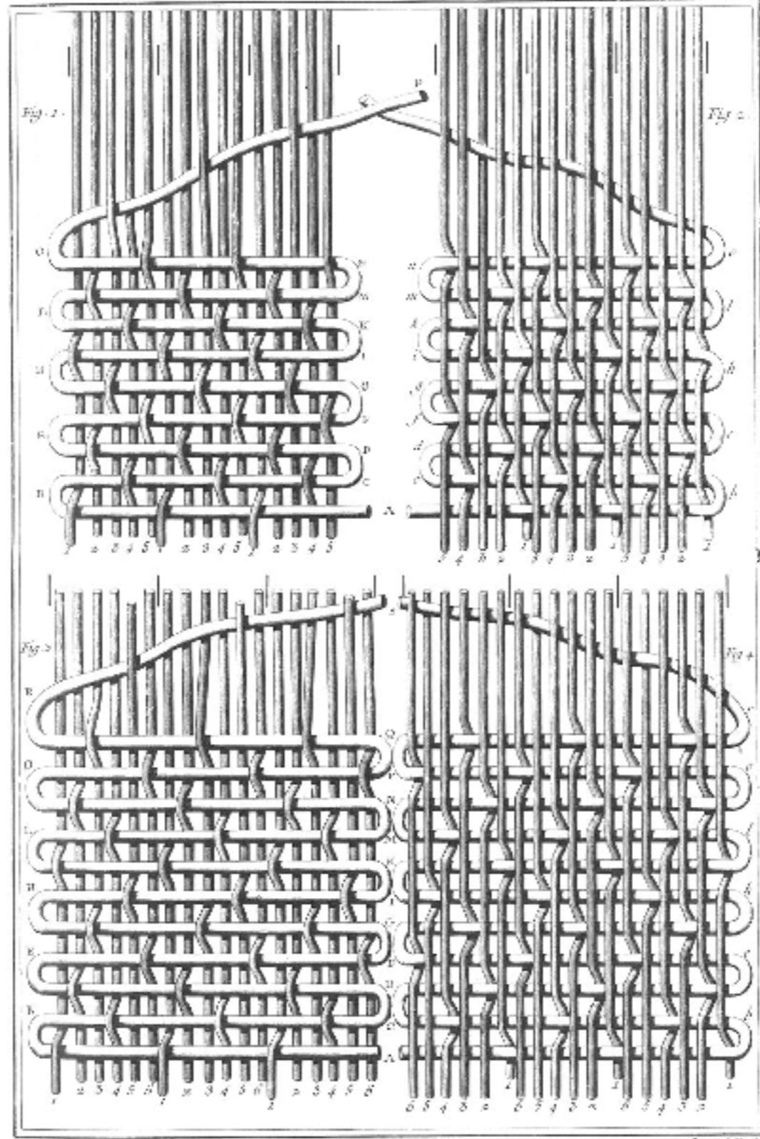
Soierie, Étoffes en Plein, satin à 6, à 6 Lisses vue du côté de l'envers et du côté de l'endroit.
