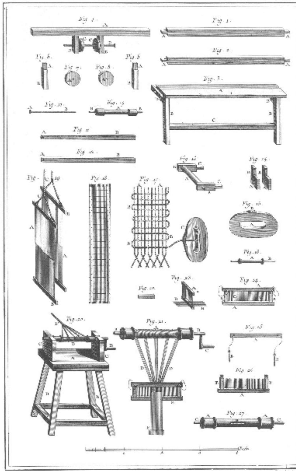
Passementerie, détail du Métier à la Raie Laine et du Ployoir.
