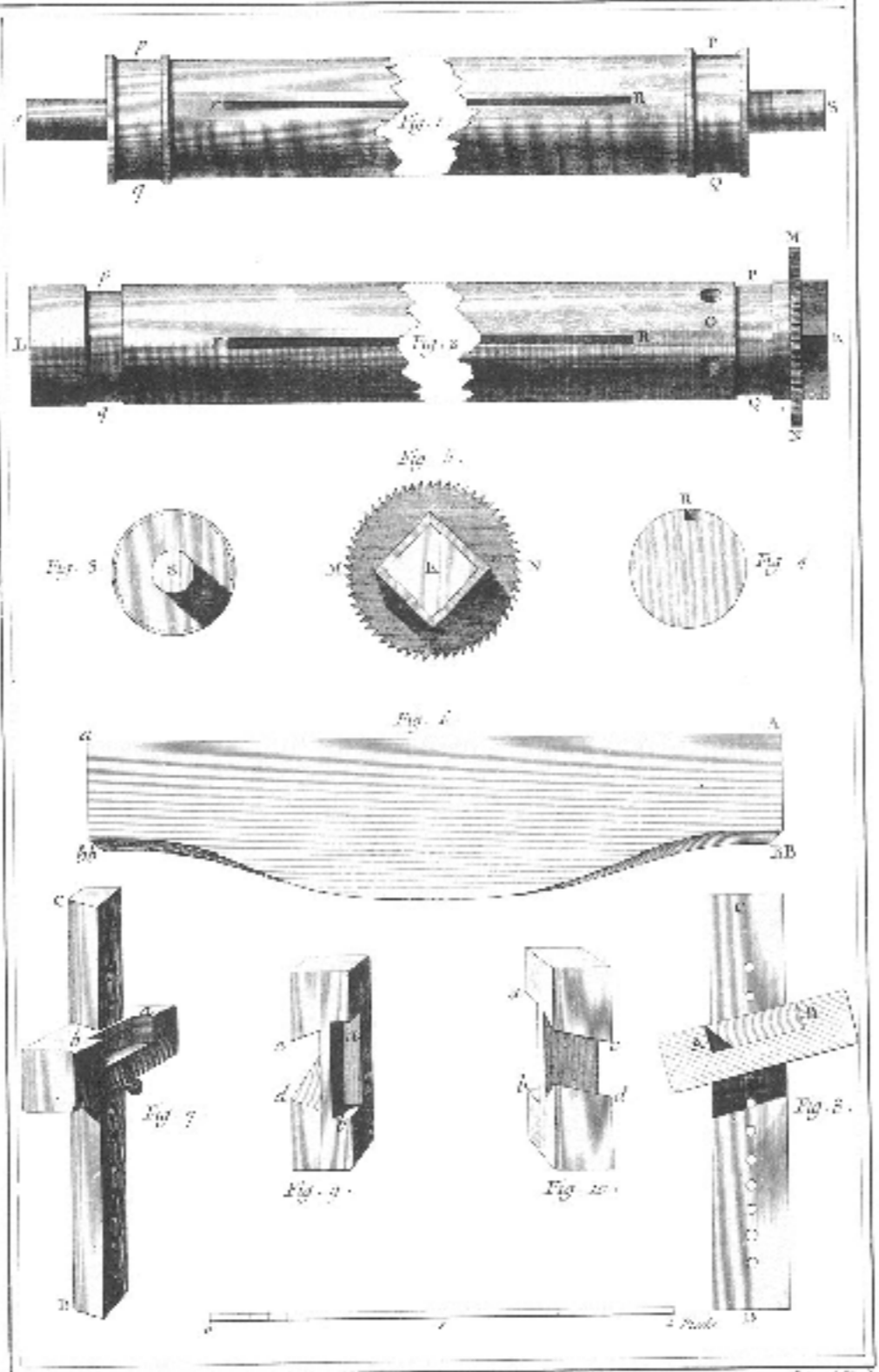
Soierie, développement des Envelopes du métal pour fabriquer les Etoffes, et Construction du tronc de l'Ourier.
