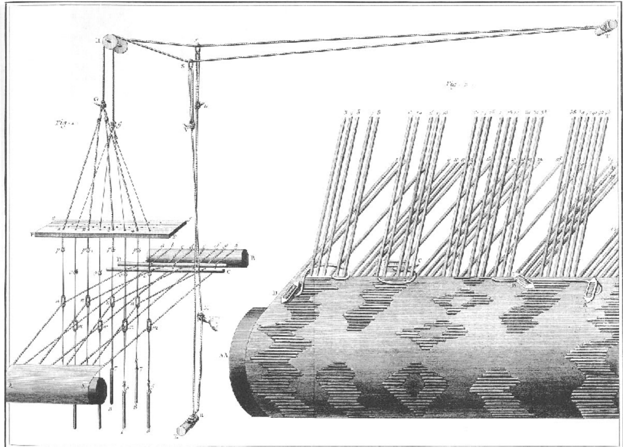
Soierie, Développement des Cordes de Ramme et de Sample et leur action sur les Vils de la Chaîne des Étoffes Brochées ou le Poil des Velours frizés et Coupés. Partie d'Étoffe Brochée Vue du côté de l'envers et au microscope.
