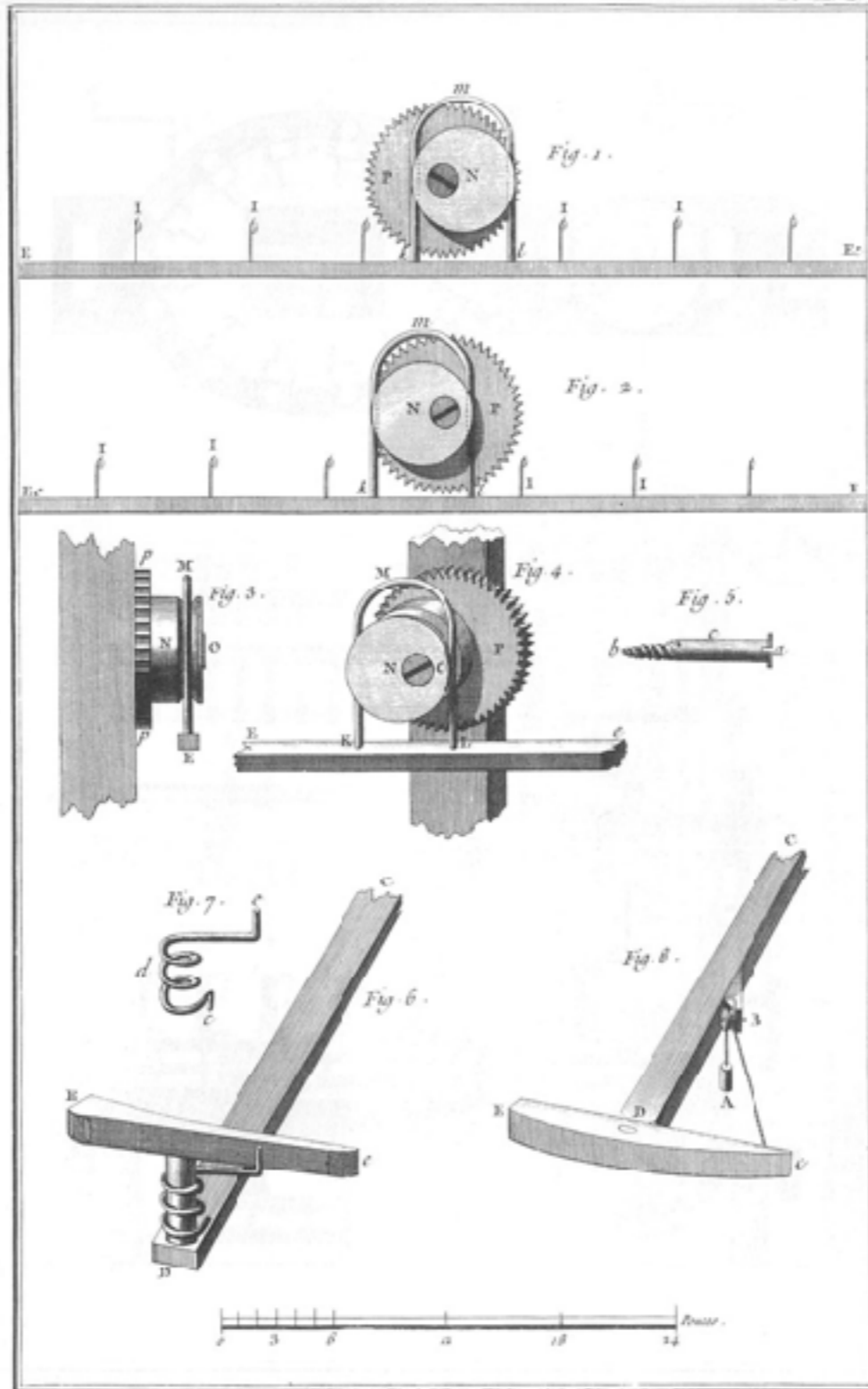
Soierie, Moulin pour Organsiner les Soies, Développement du Fâ-à-Vent, et des surfiles.
