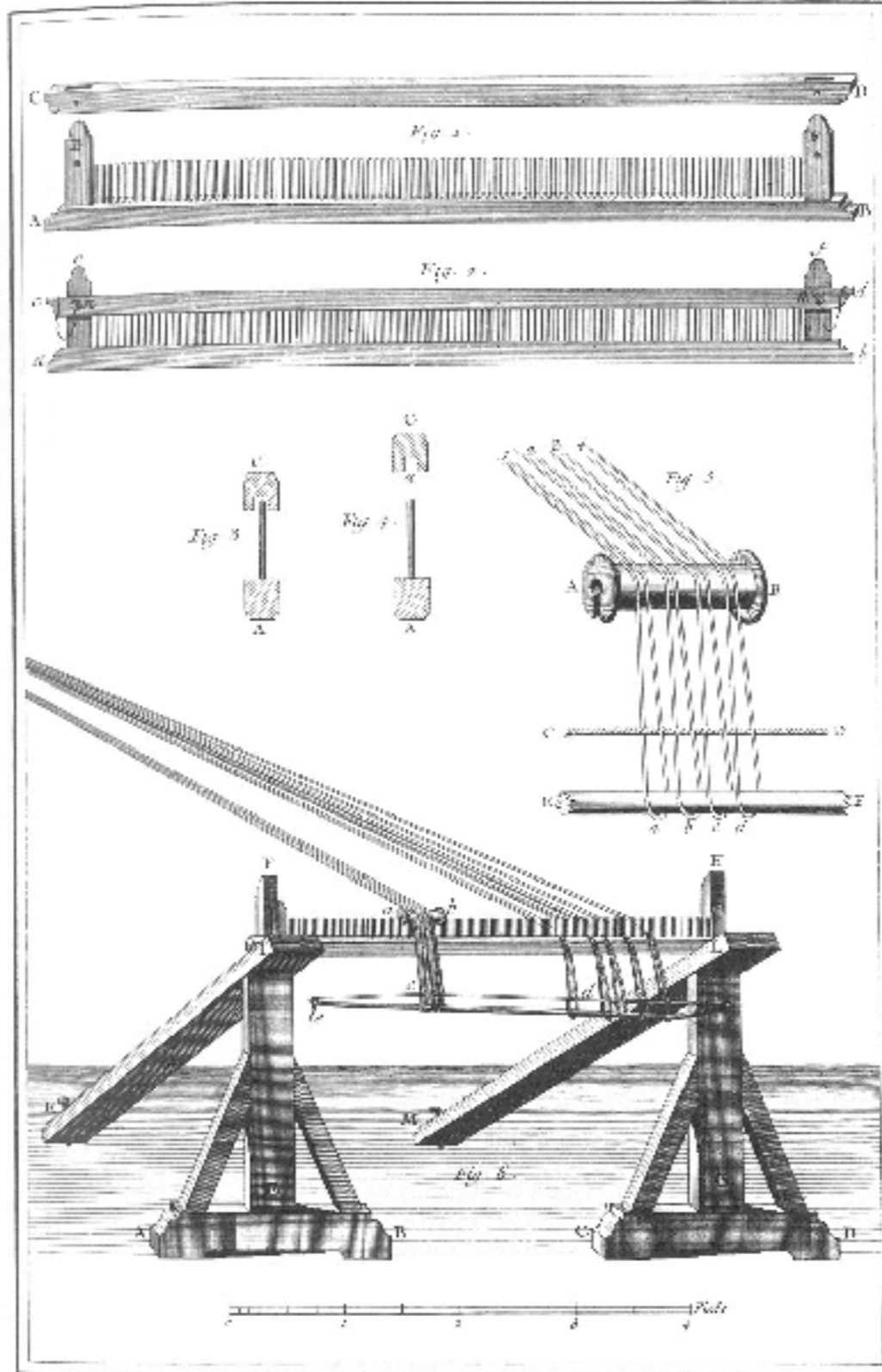
Soierie, l'opération de Ployer et Développement du Ratoum. FF
