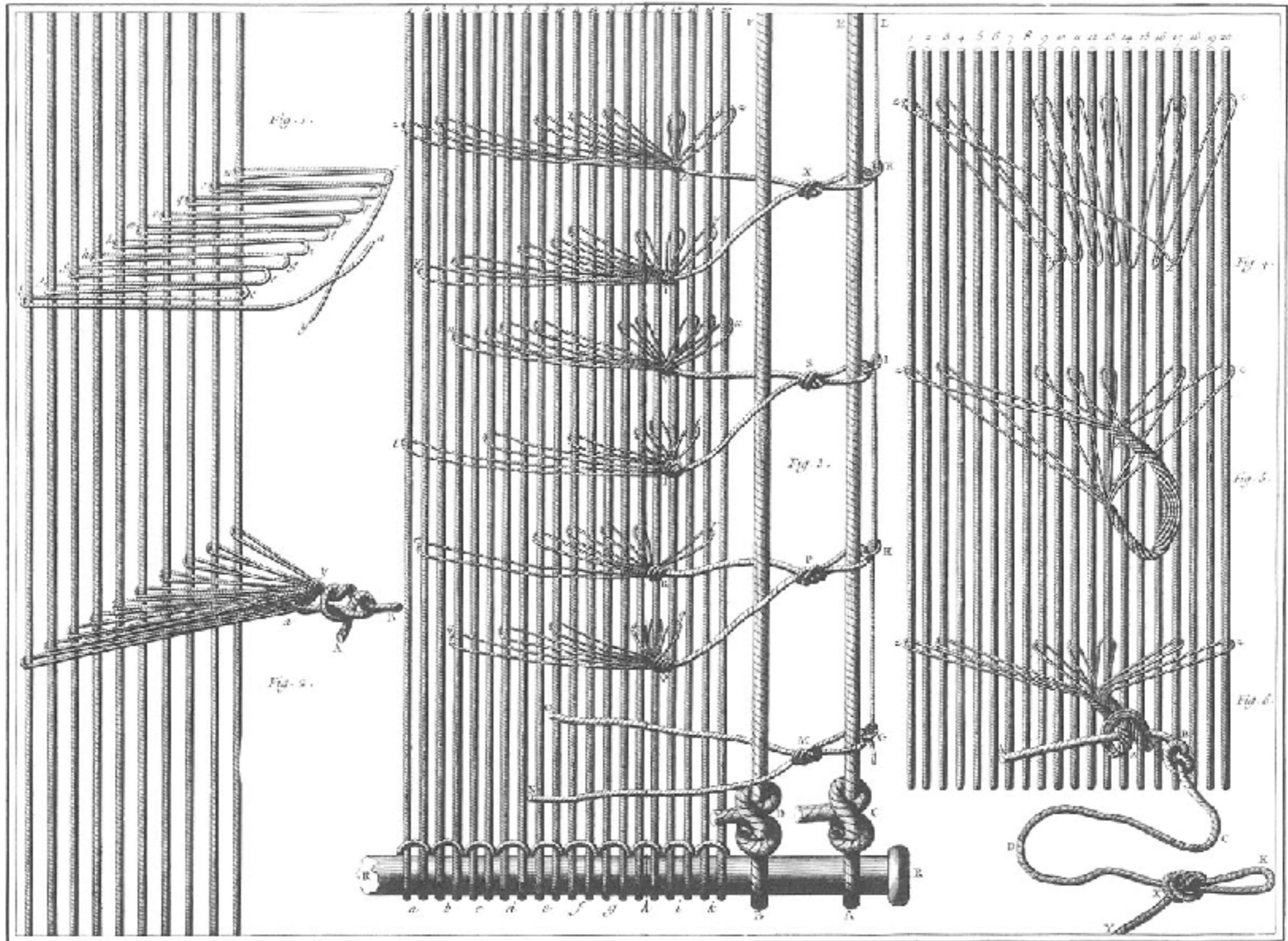
Soierie, Lacqs. Lacq à l'Angloise, Lacqs du Simple, Cavassine et formation d'un Lacq.
