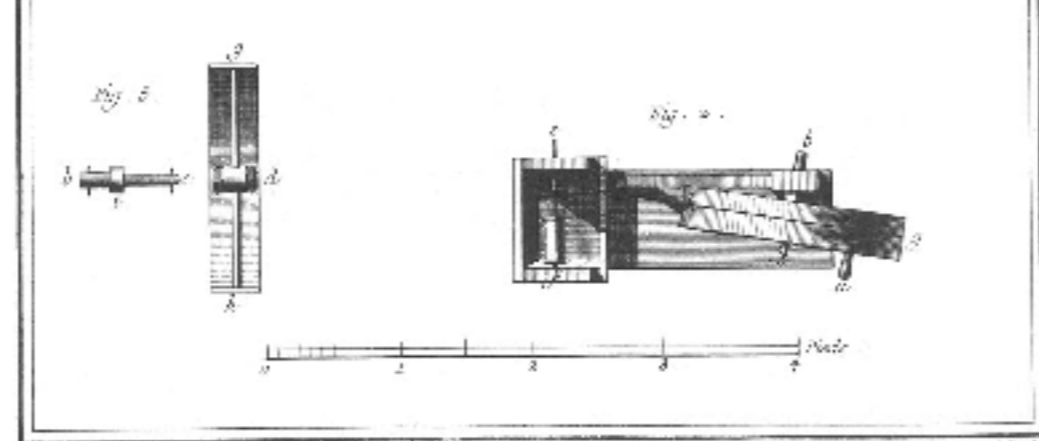
Soierie, Doublage des Soies, Construction du Rouet. G
