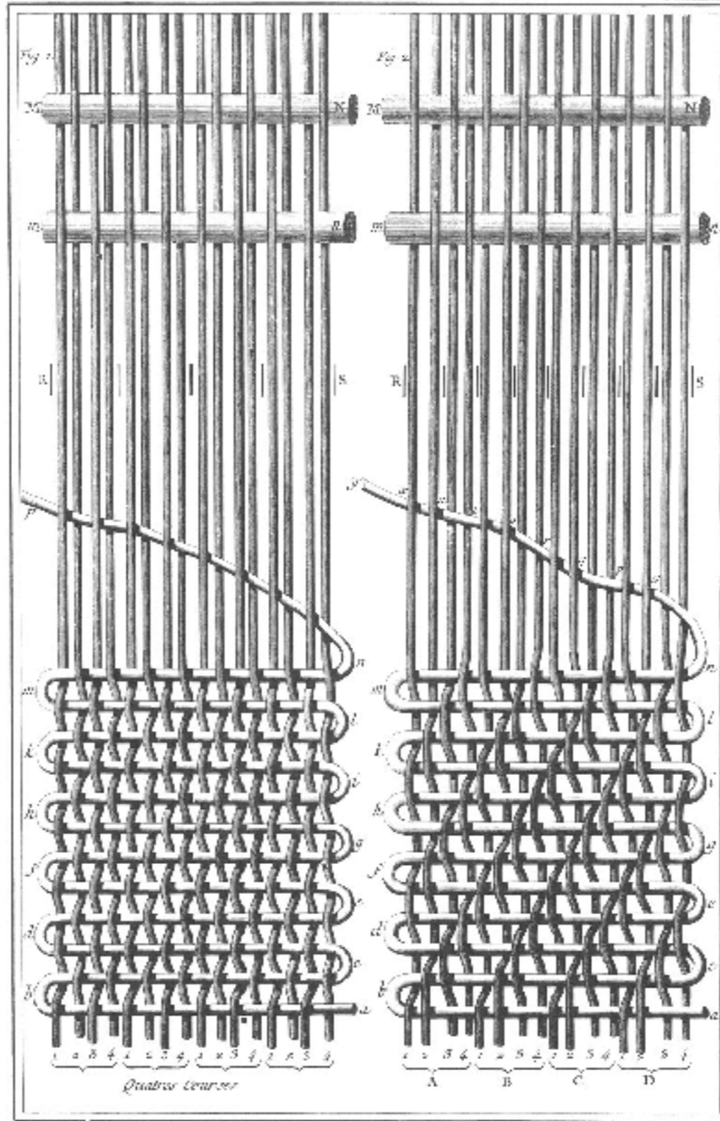
Soierie, Ruffes en Plain, le Taffetas et le Ras de St. Sire.
