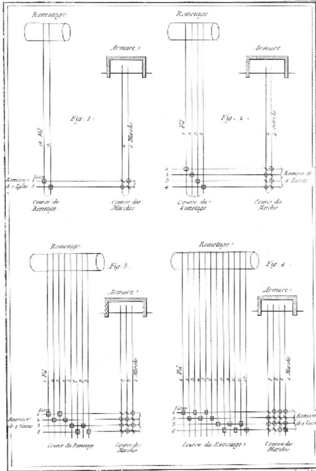
Soierie, Armures du Taffetas à 2 Lisses ou Armures, autre Armure générale pour toutes sortes de Taffetas et Gros de Tours: Armure de l'Ettoffe nommée Vrai de Poille, et Armure pour la Siamoise.
