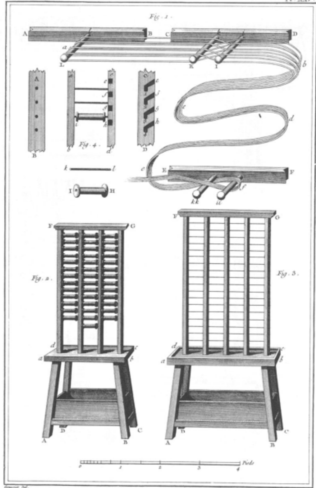
Soierie, Développement de la Canthre ou Banque et de l'Encroix par Fils et par Portées B.B
