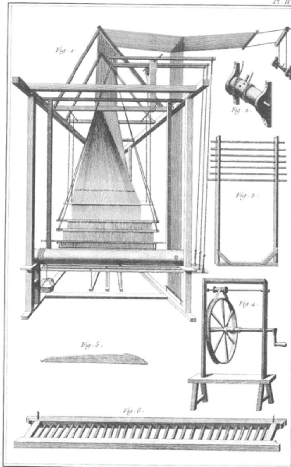
Gazier, Métier à Gaze vu en face.
