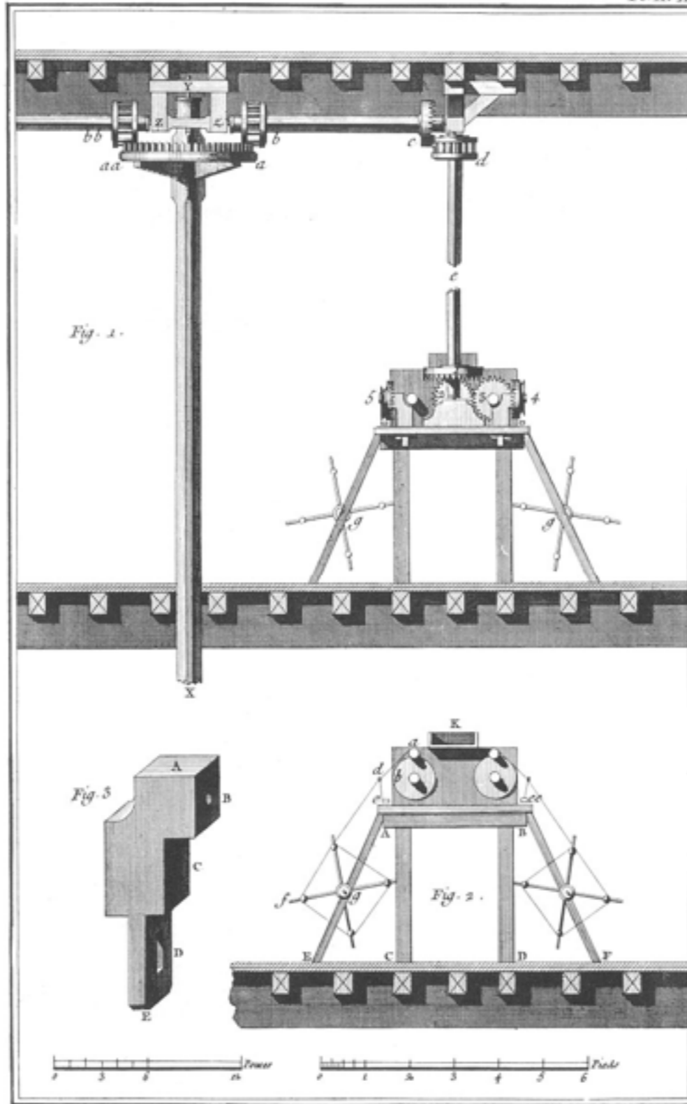
Soierie, Profile du Devidage qui est au dessus des Moulins à Organiser les Soies. R
