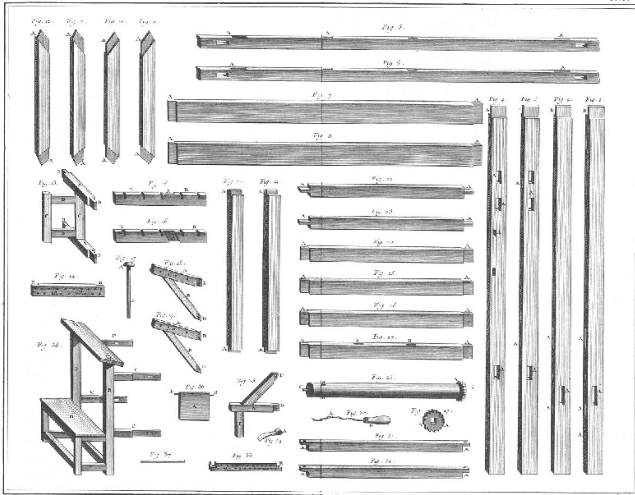
Passenterie, détail de Meuble à faire le Galon.
