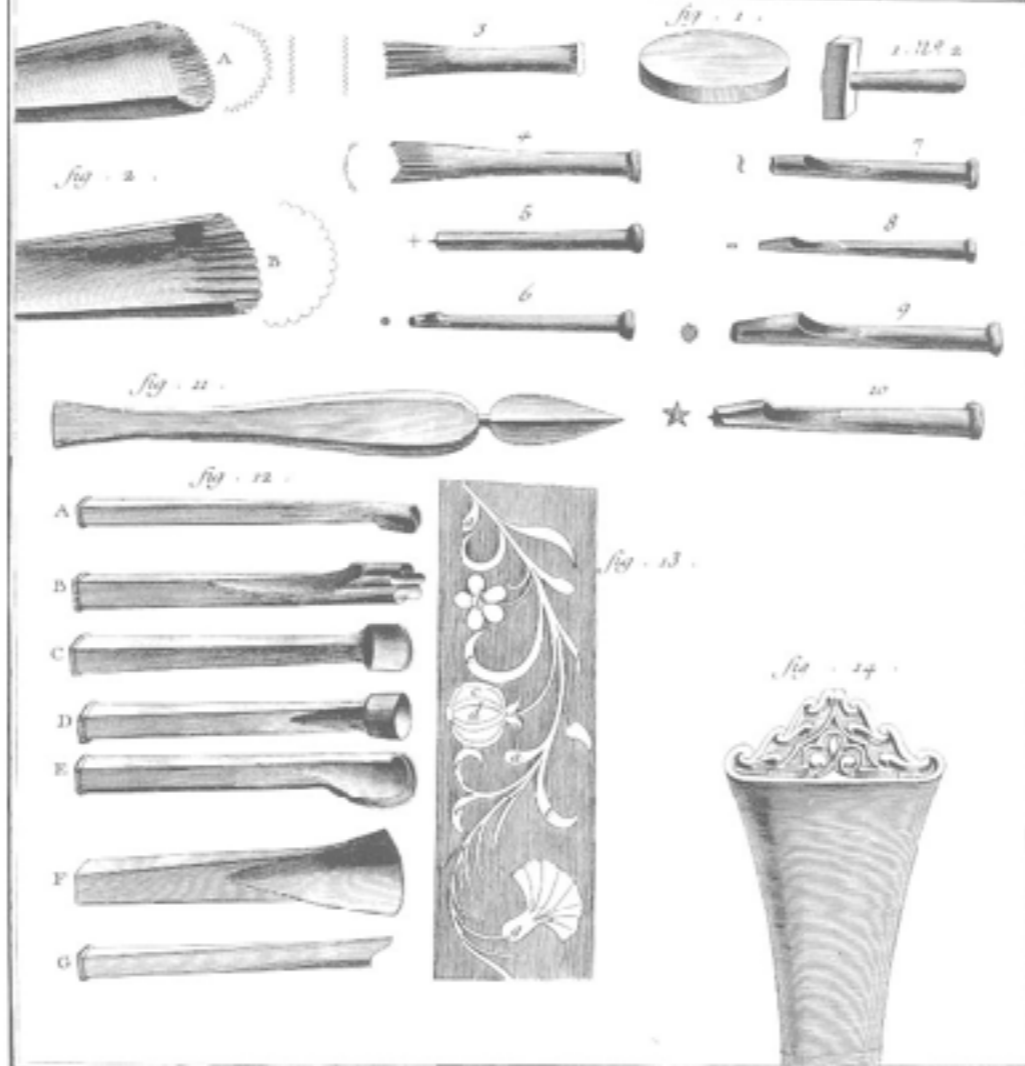
Découpeur et Gausseur.
