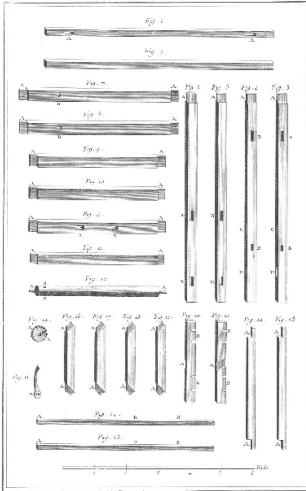
Passementerie, Détails du Metier à la Basée Liffée.
