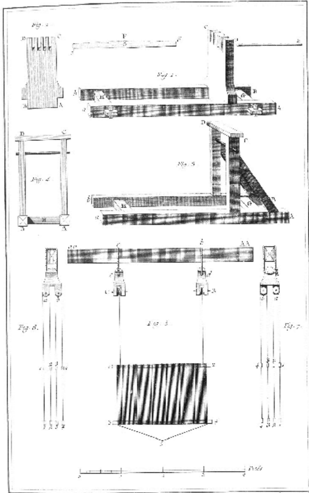
Soierie, Développement de la Cuculle et du Porte-Licse.
