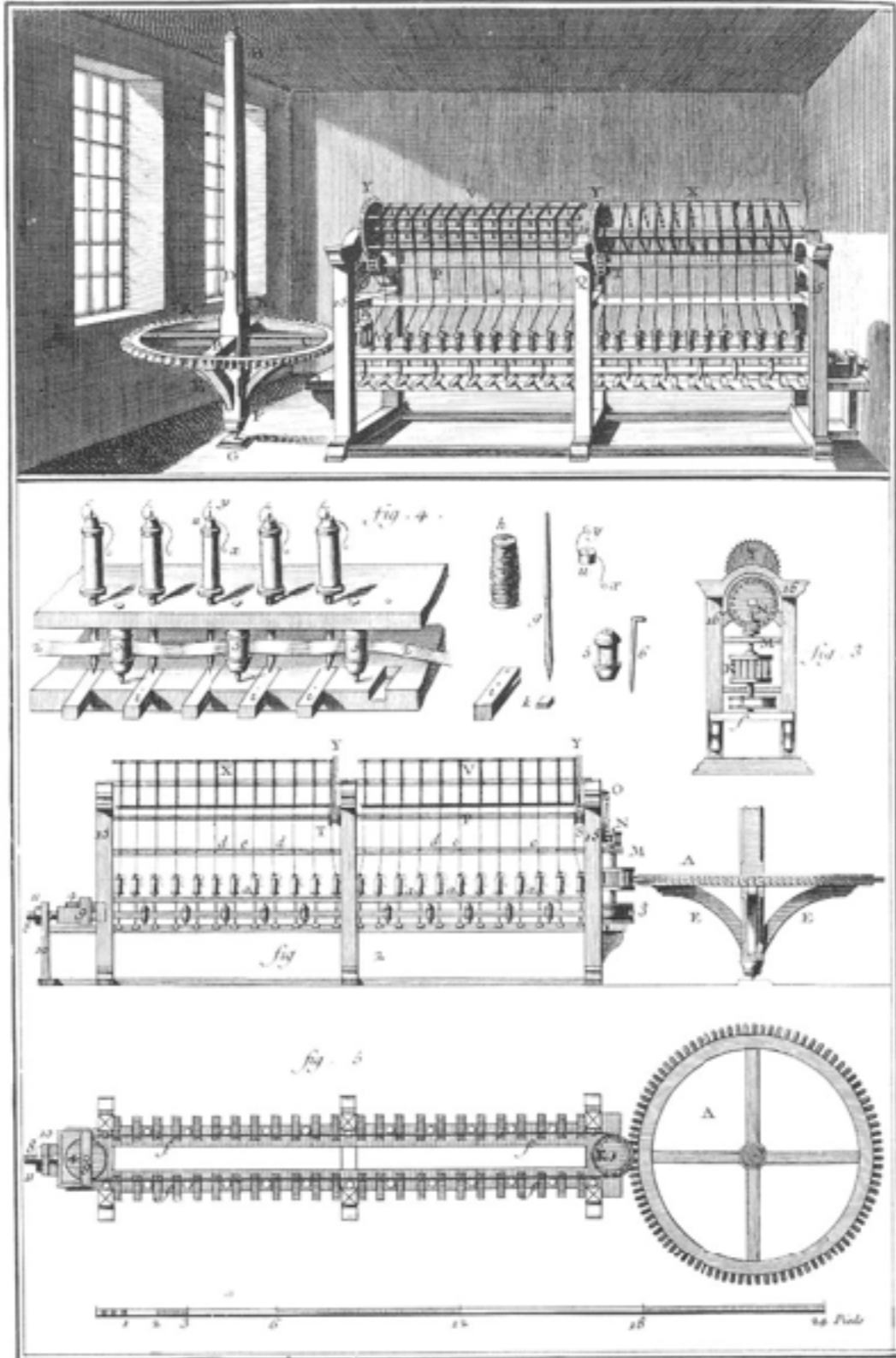
Fil, Moulin Quarré.
