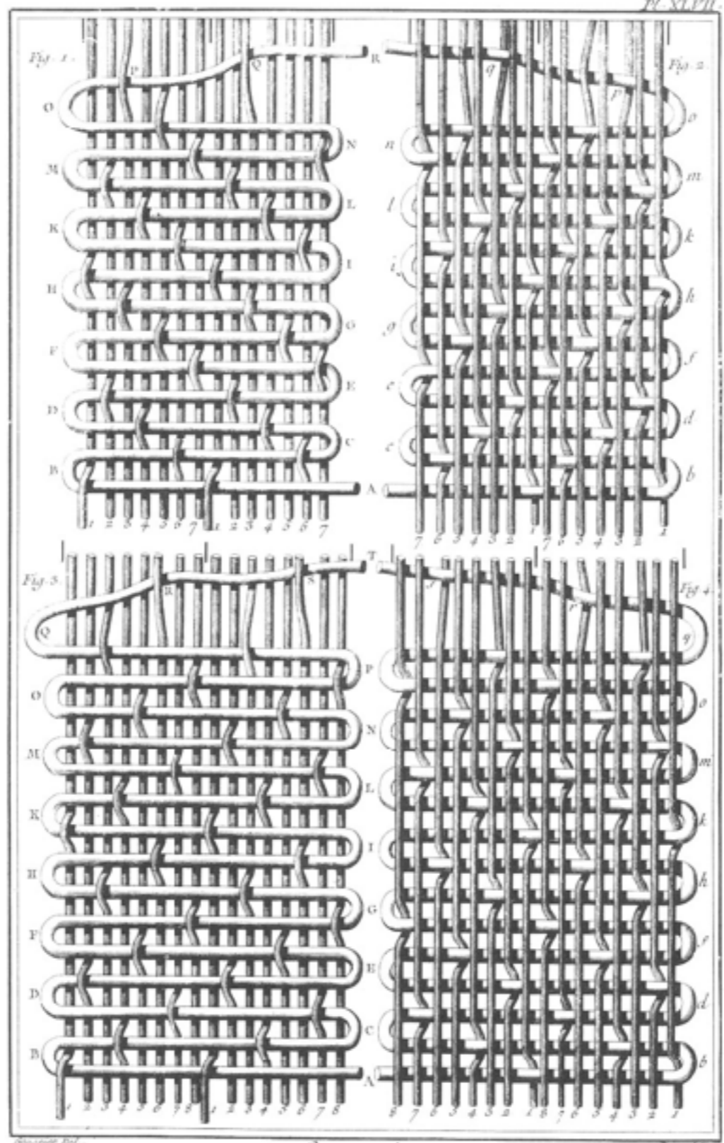
Soierie, Étoffes en Plein, Satin à 7 Torsas et Satin à 8. Vus par l'Envers et l'Endroit.
