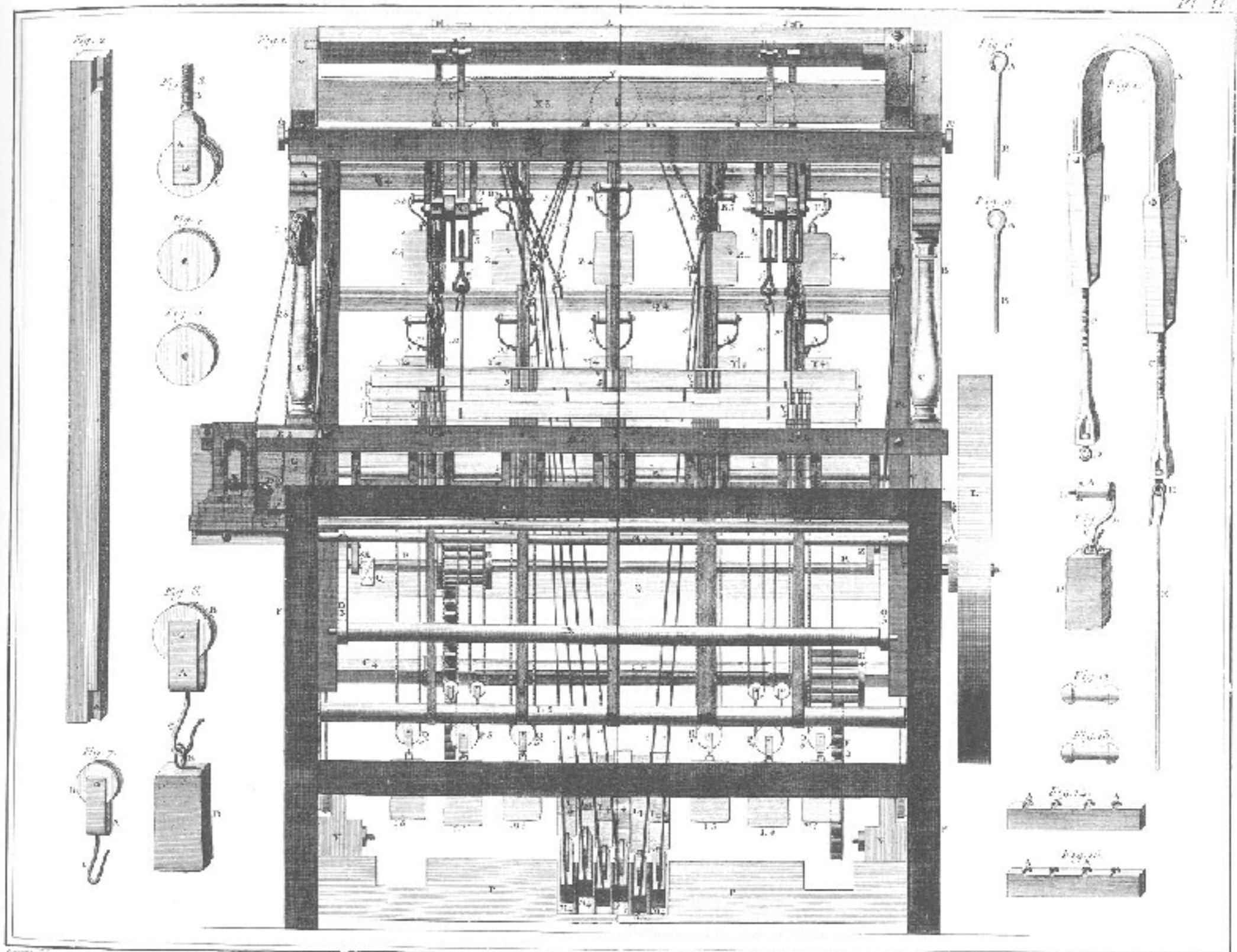
Métier à faire le Ruban, Étendue en face.
