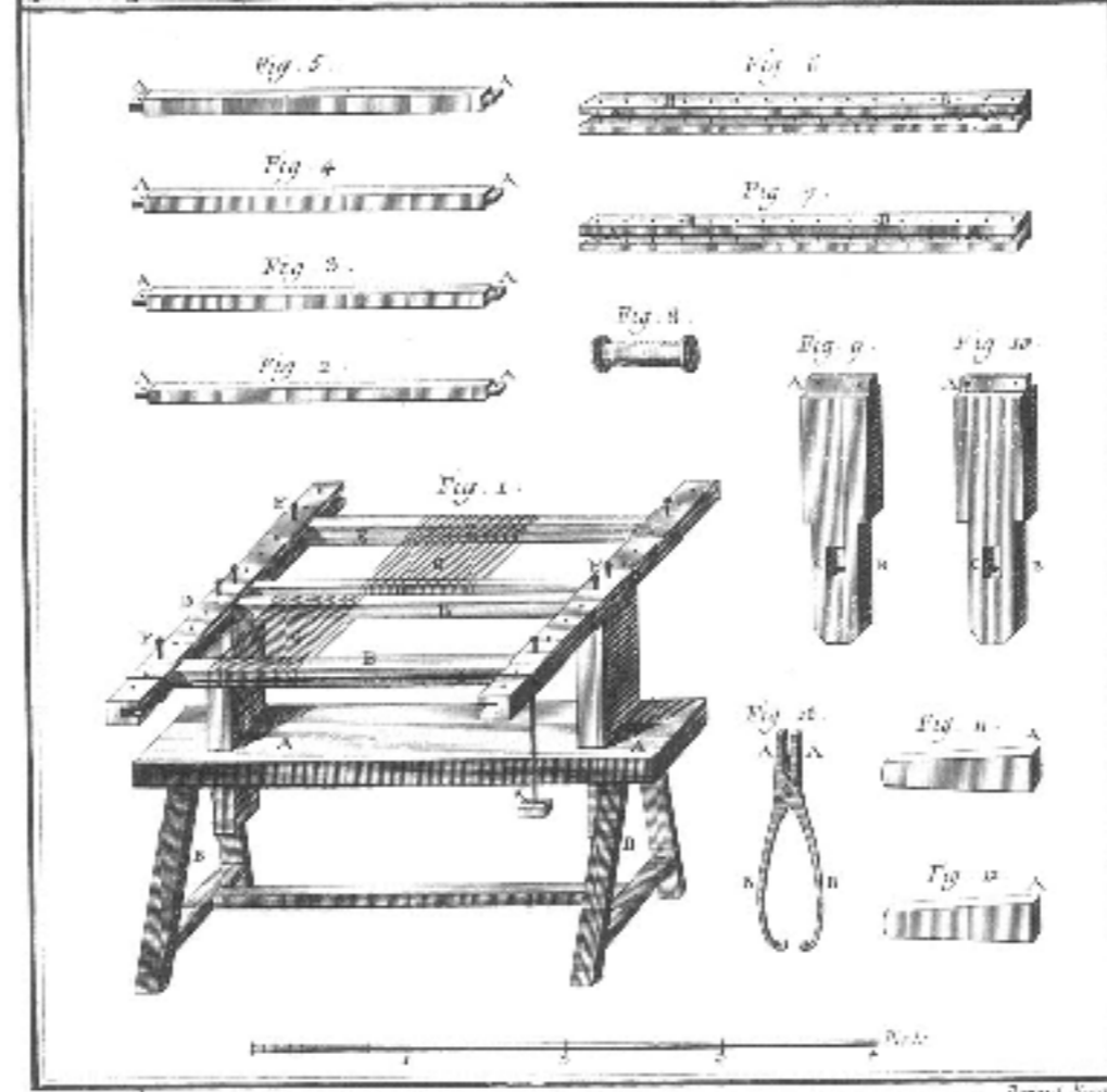
Passementerie , Façon des Laffes .
