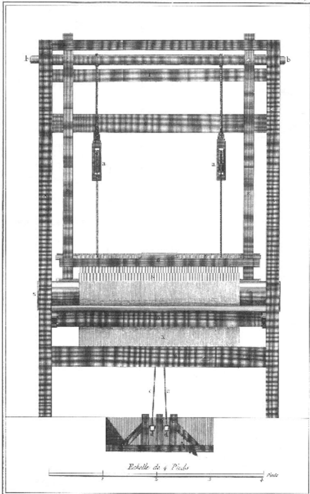
Tisserand, Elevation en face du Metier à faire la Toile.
