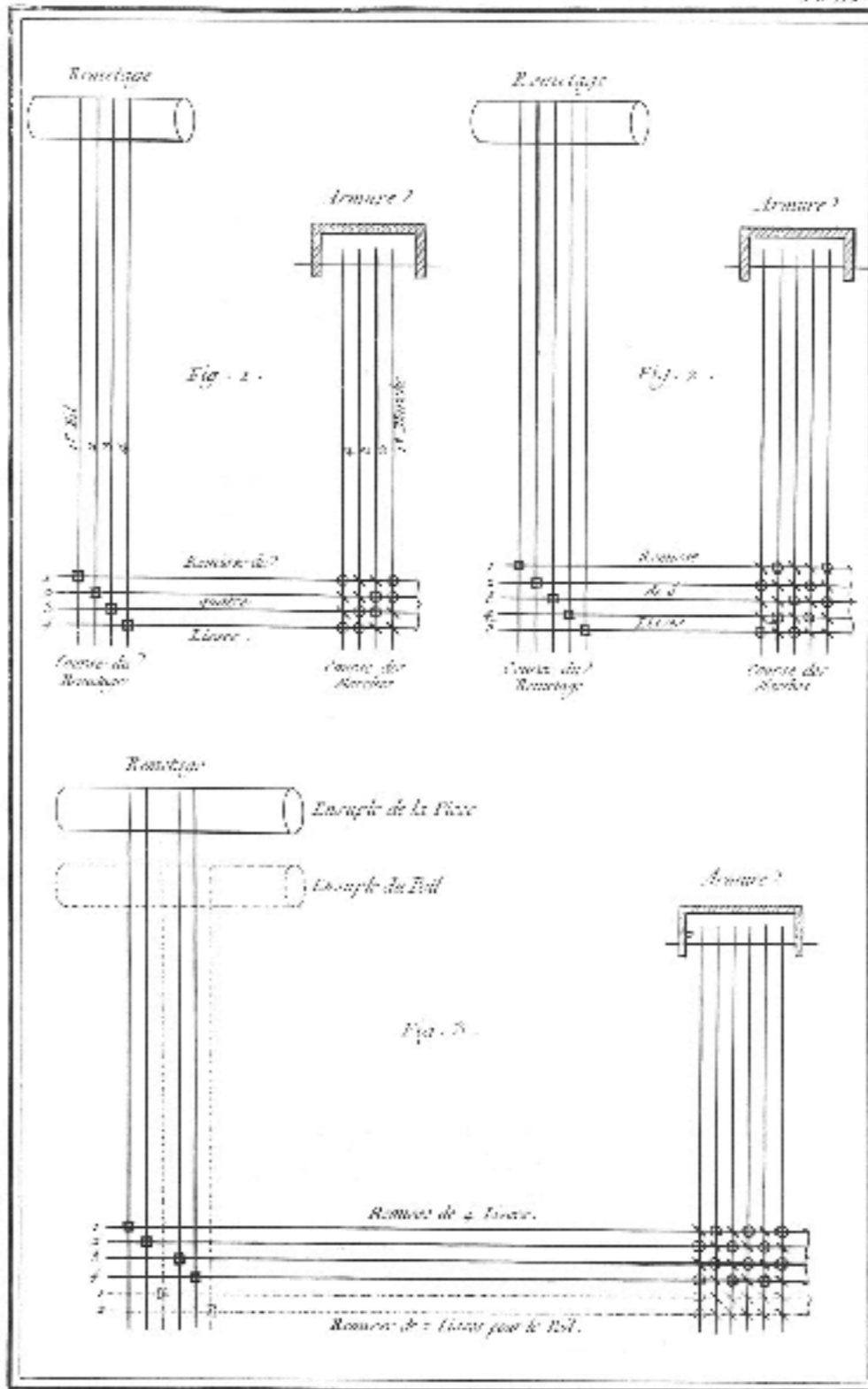
Soierie . RR 1. Raz de St. Maur, 2. Stoffe qui est Gros de Naples d'un côté et Raz de St. Maur de l'autre, 3. Canelé à Poil.
