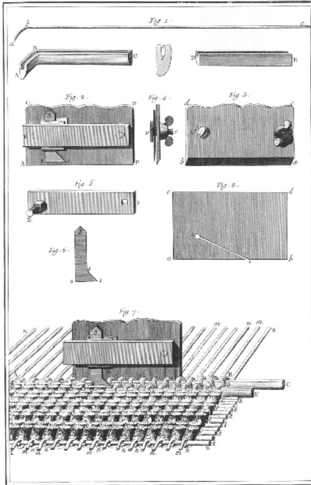
Soierie; Velours Coupé. Fens de Coupé, Rabot, m.m.m Vullerolle: Voage du Rabot et Velours Coupé Vu au Microscope et en perspective
