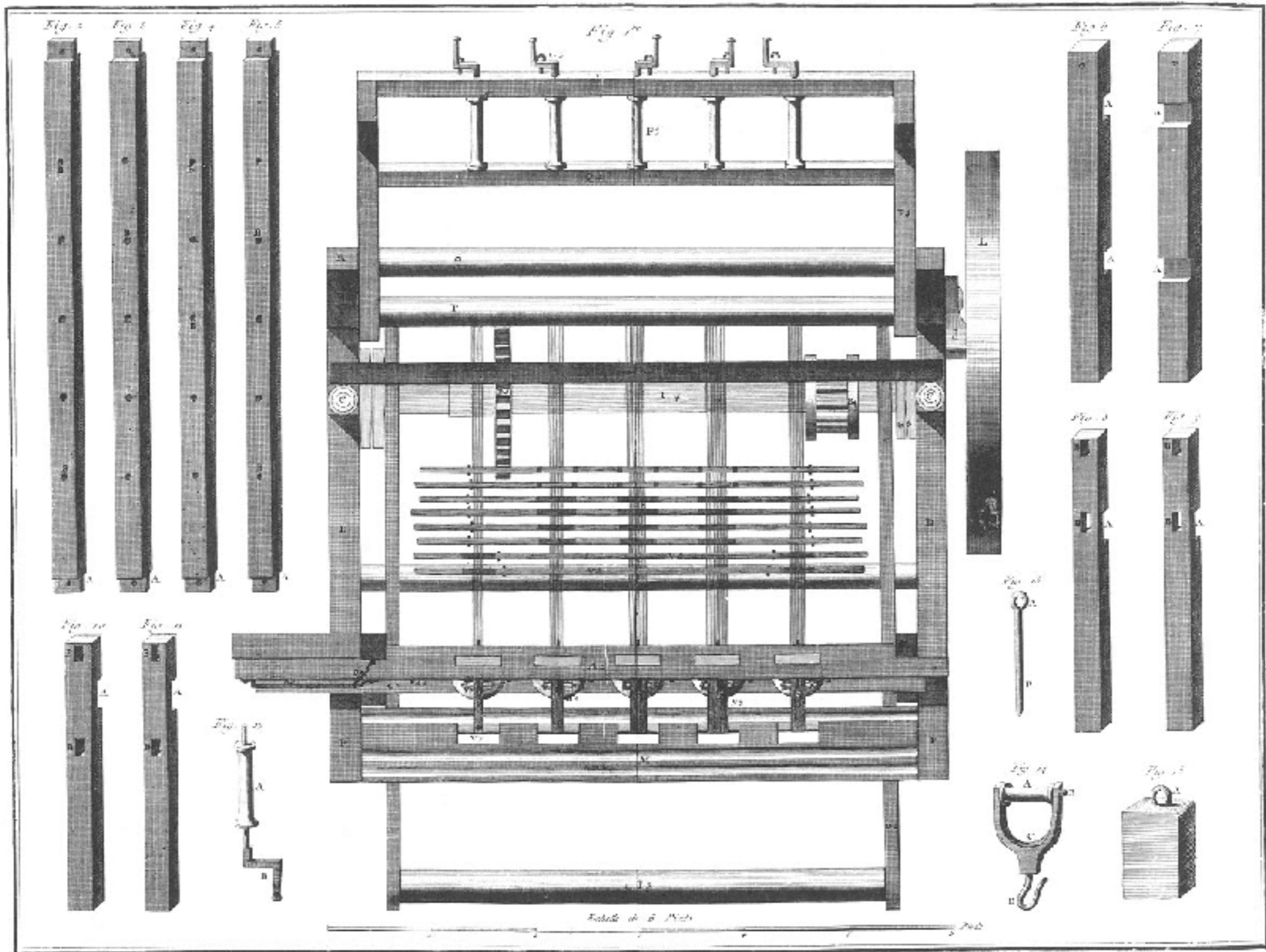
Métier à Ruban, Plan 300 Lances.
