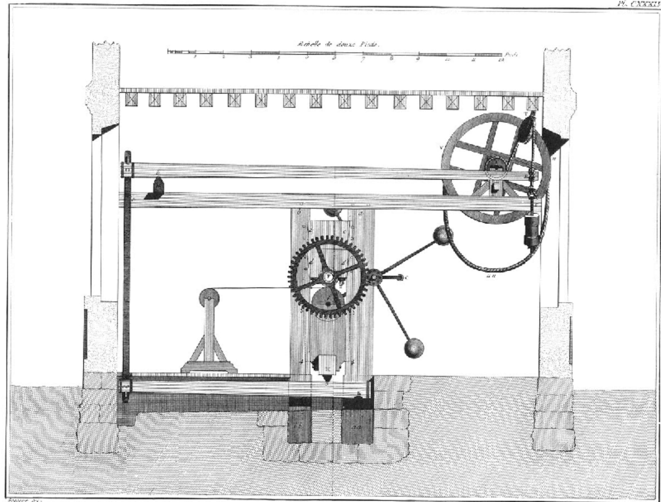
Soierie, Élevation Latérale de la Machine servant à cylindrer les Étoffes.
