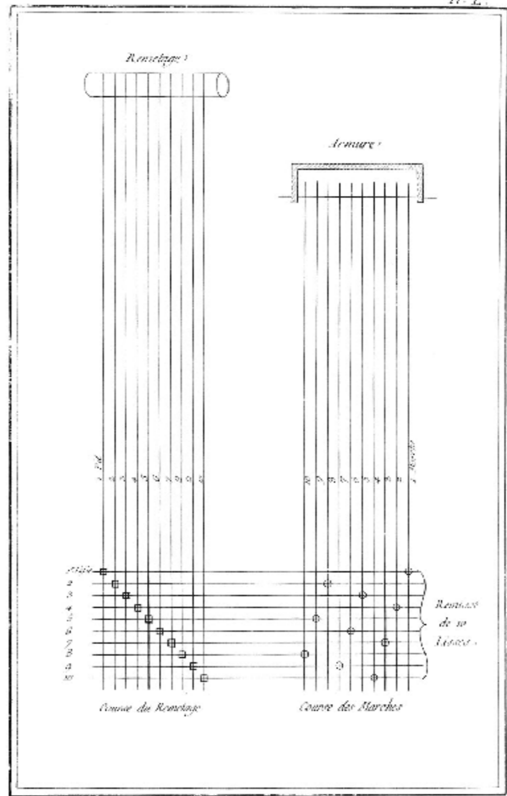
Soierie, Satin à Dix Lisses.
