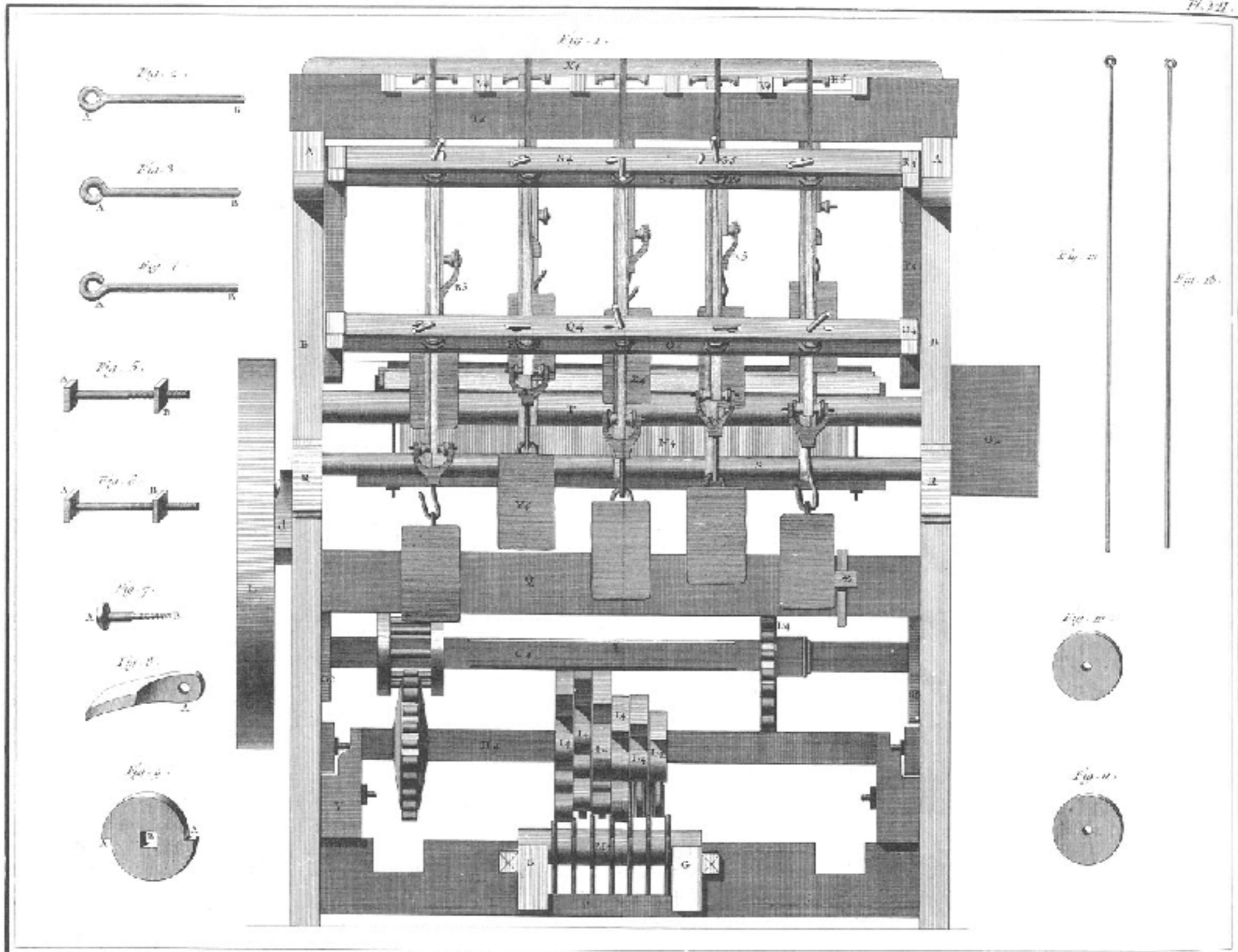
Métier à faire le Ruban, élévation par derrière.
