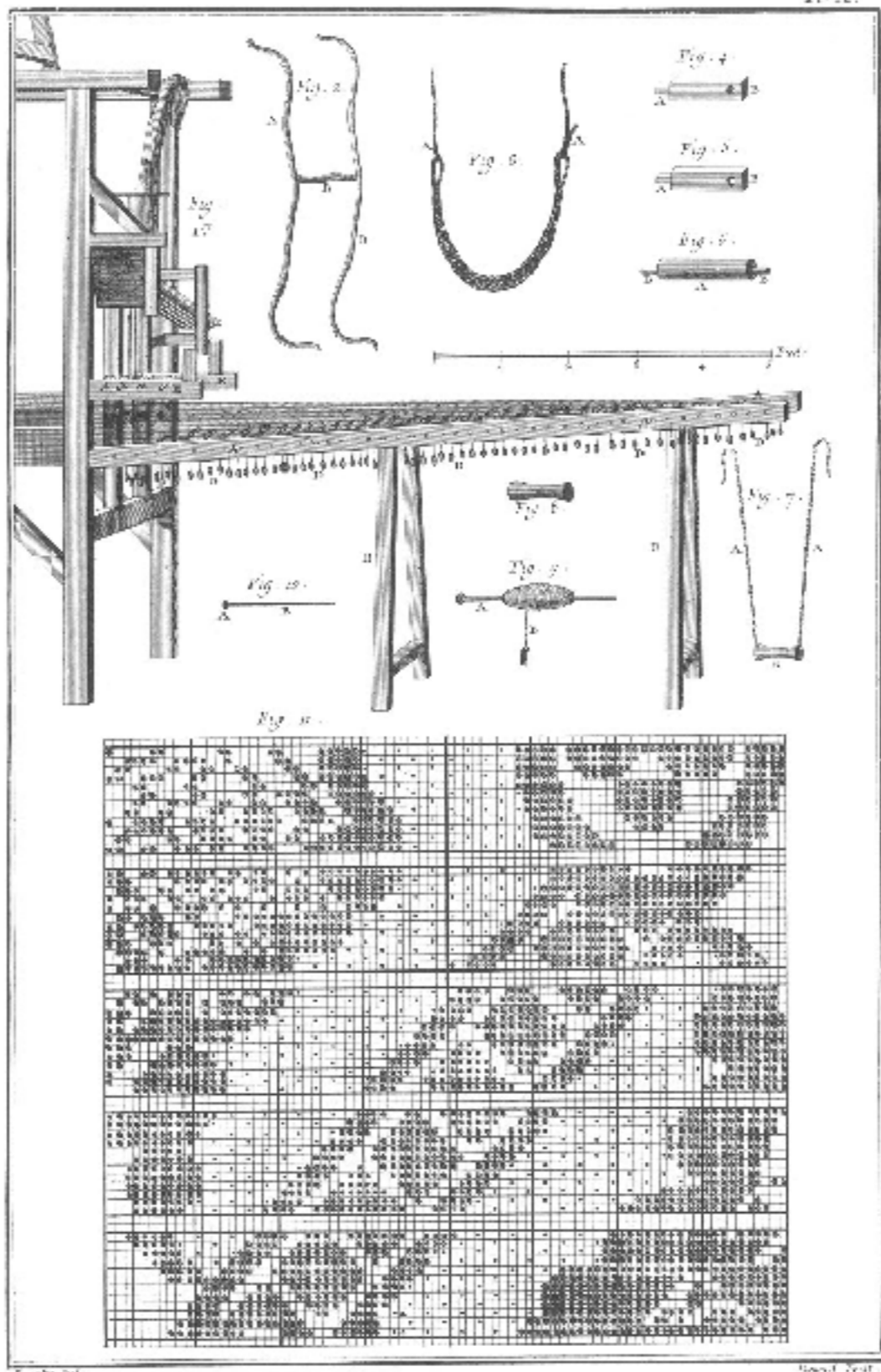
Passementerie, Mâtier et Laminé et Patron.
