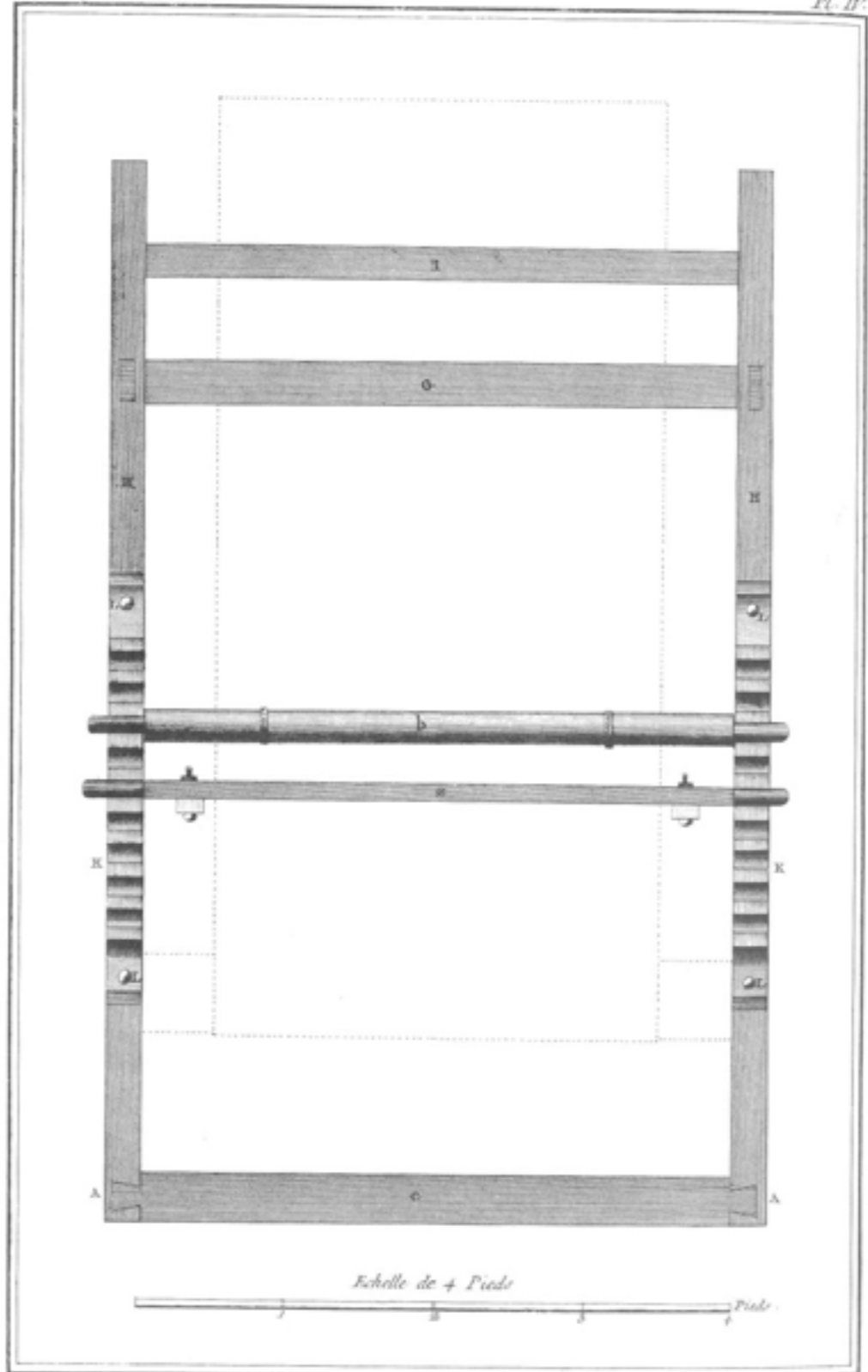
Tisserand, Plan du haut du Mètier à faire la Toile
