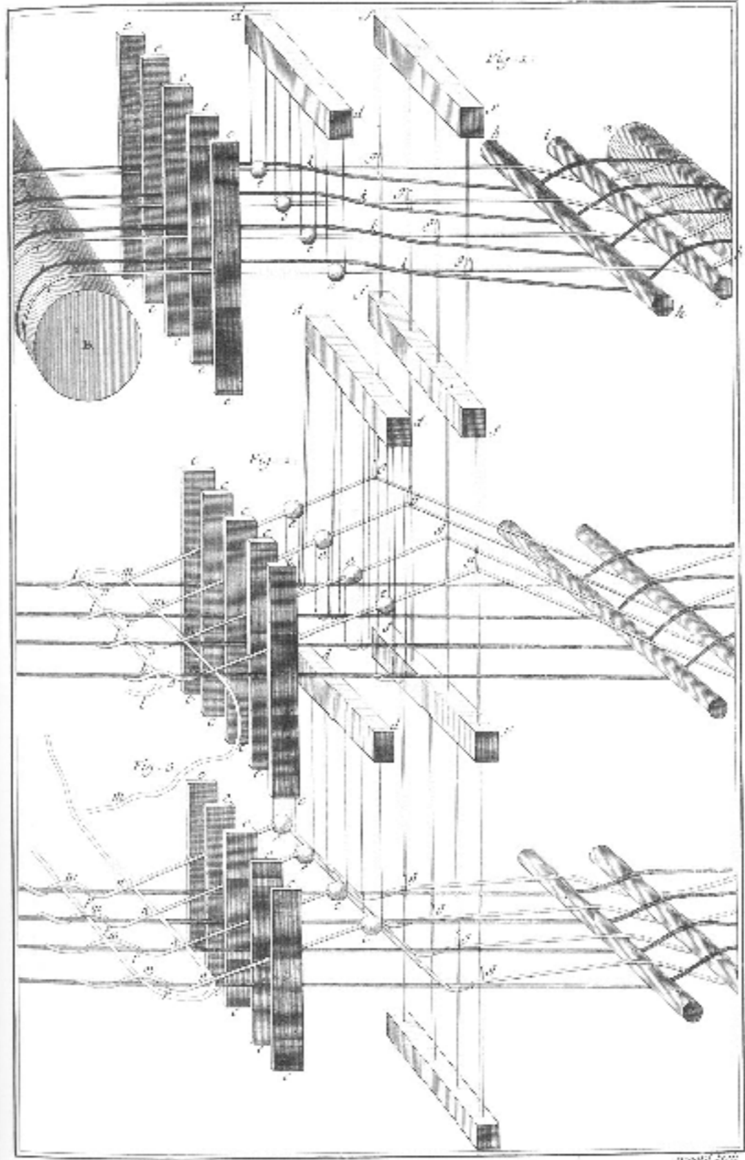
GAZIER, Fonctions des Lasses du Méier à Gaze.
