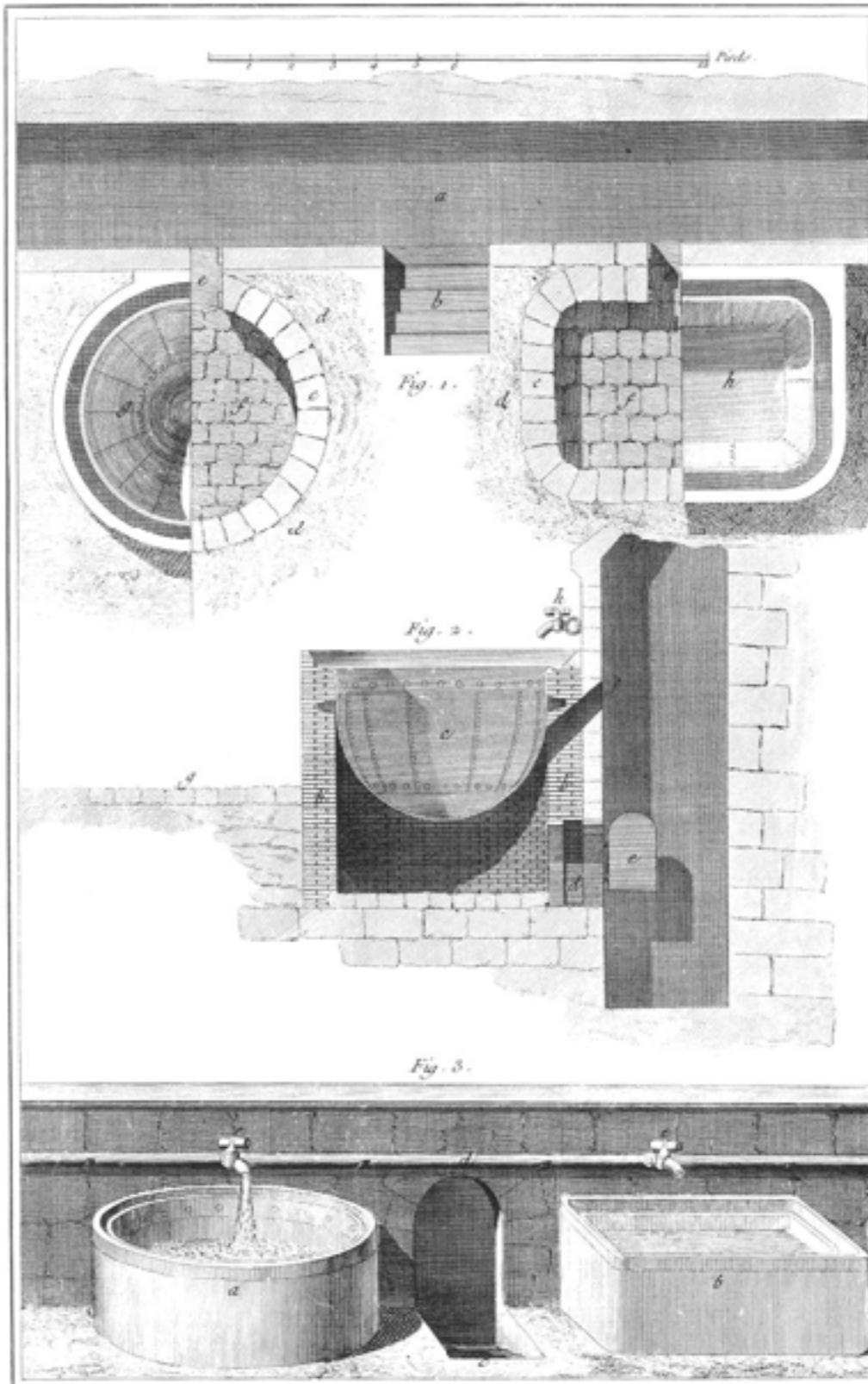
Teinturier de Riviere, plans, coupe et élévations de différentes Chaudières.
