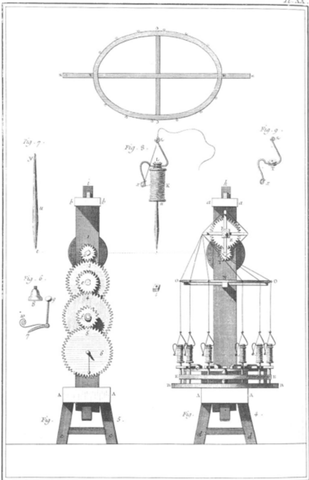
Soierie; Ovale, Coupes Transversalles et Developpemens de plusieurs Parties.
