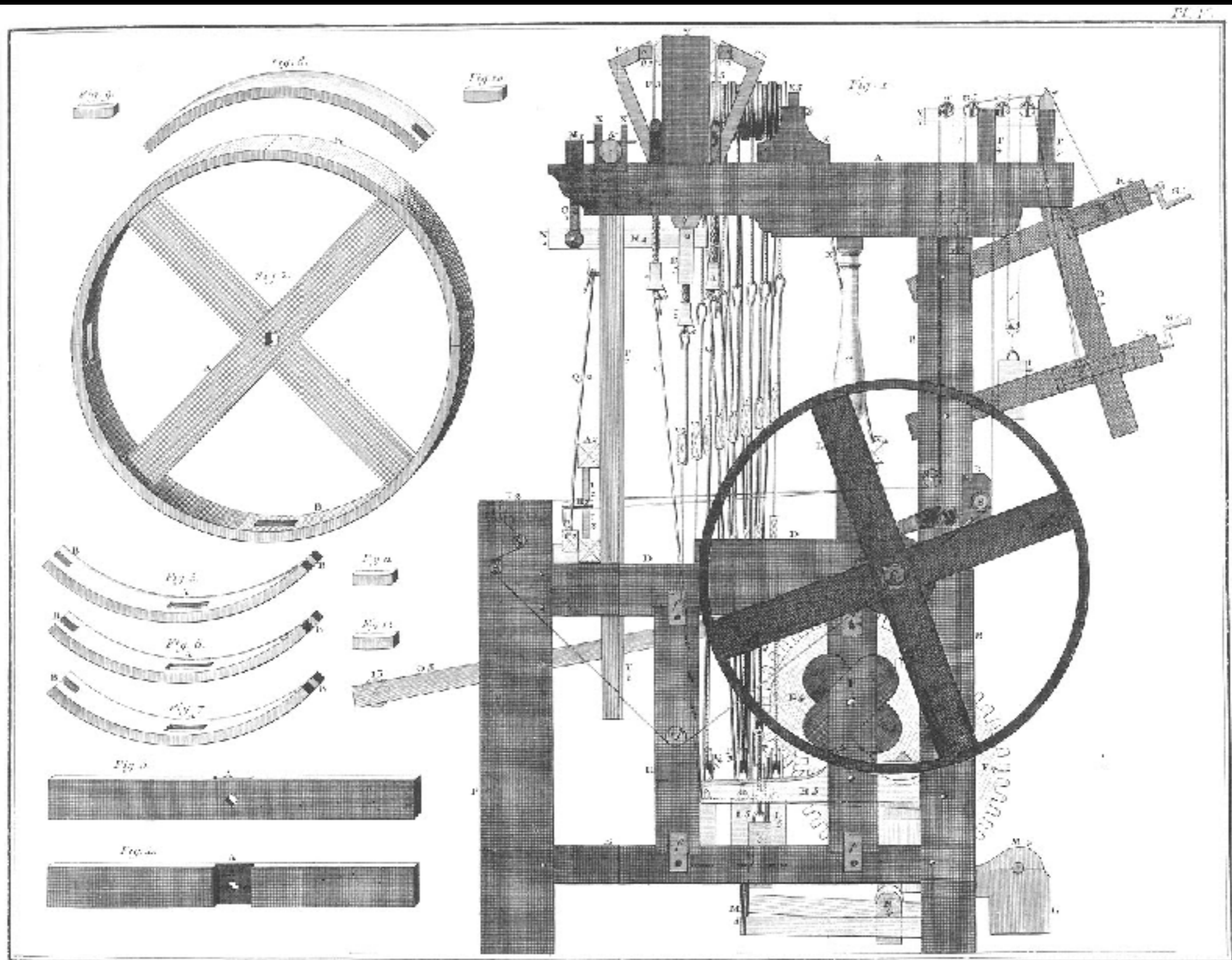
Métier à faire le Ruban, invention récente.
