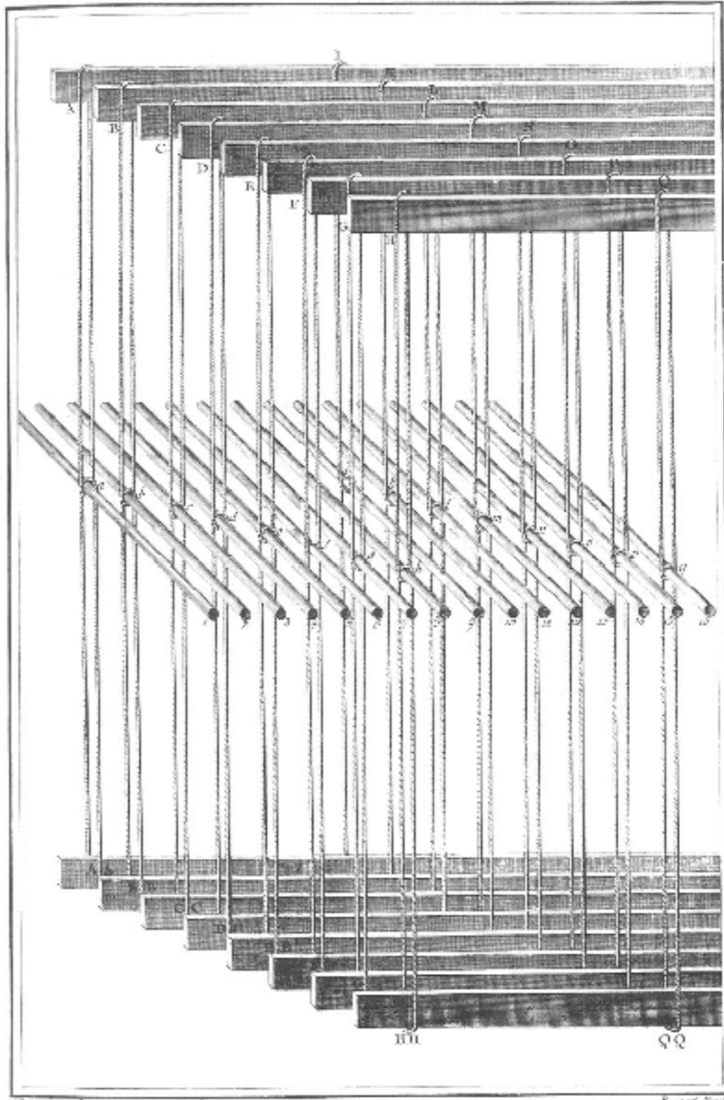
SOIERIE, Remettage ou Passage des Fils de la Chaîne dans les Taffets.
