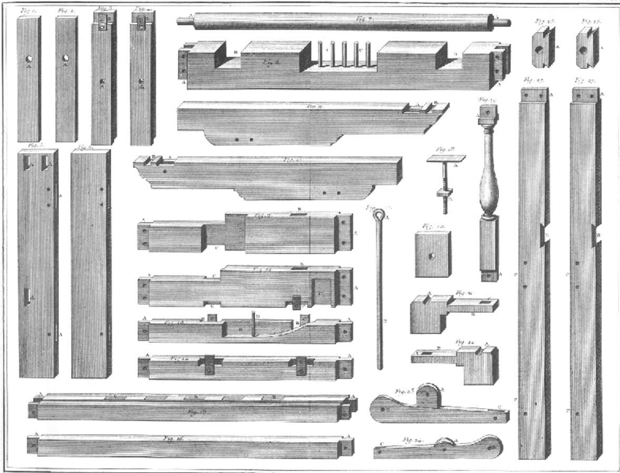
Métier à faire le Ruban, Développement.
