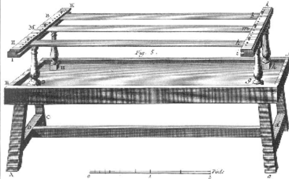
Soierie, Fabrication des Verses et le Lissoir en Perspective.
