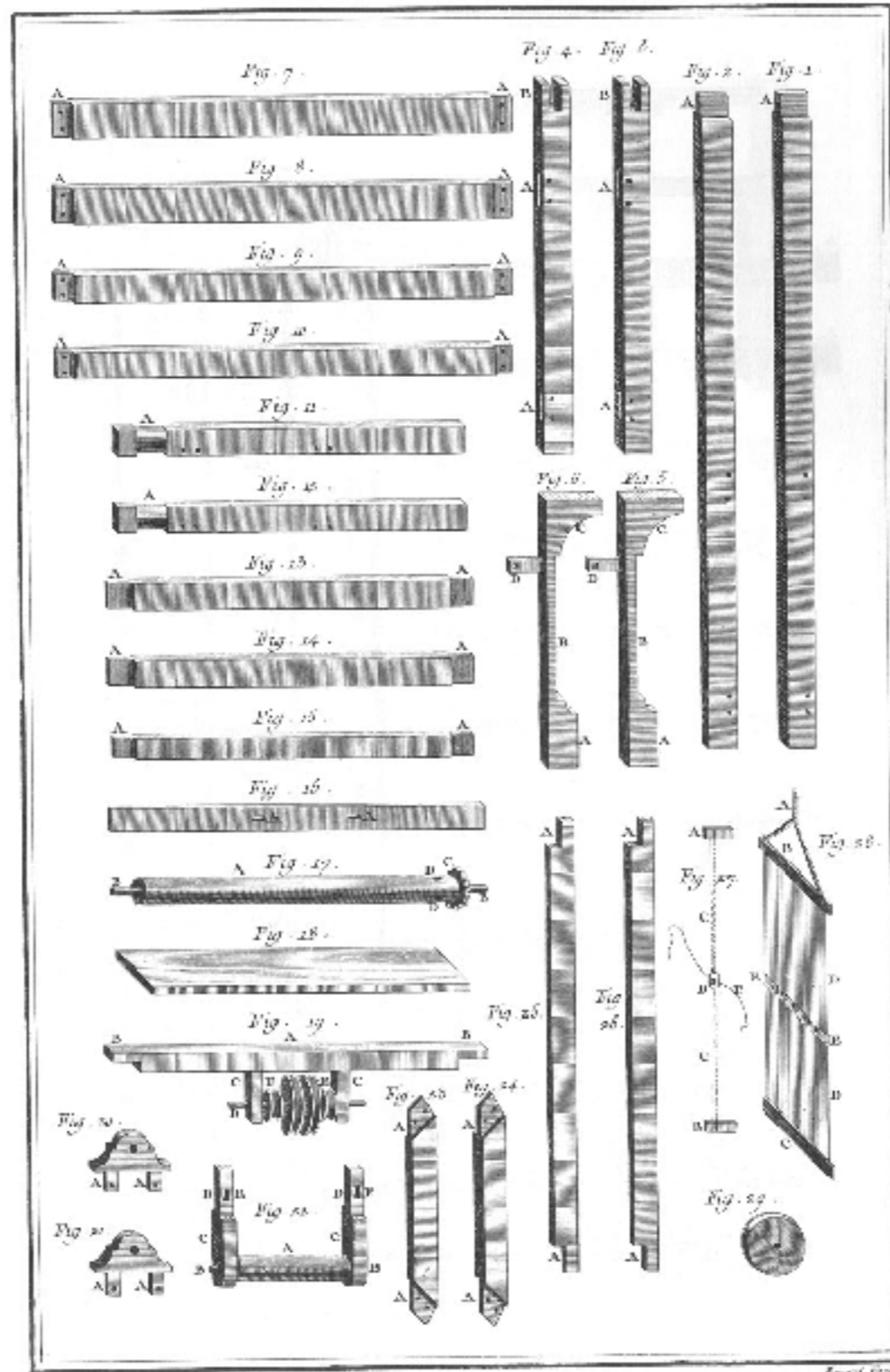
Passementerie, détail du Meier a Frapper.
