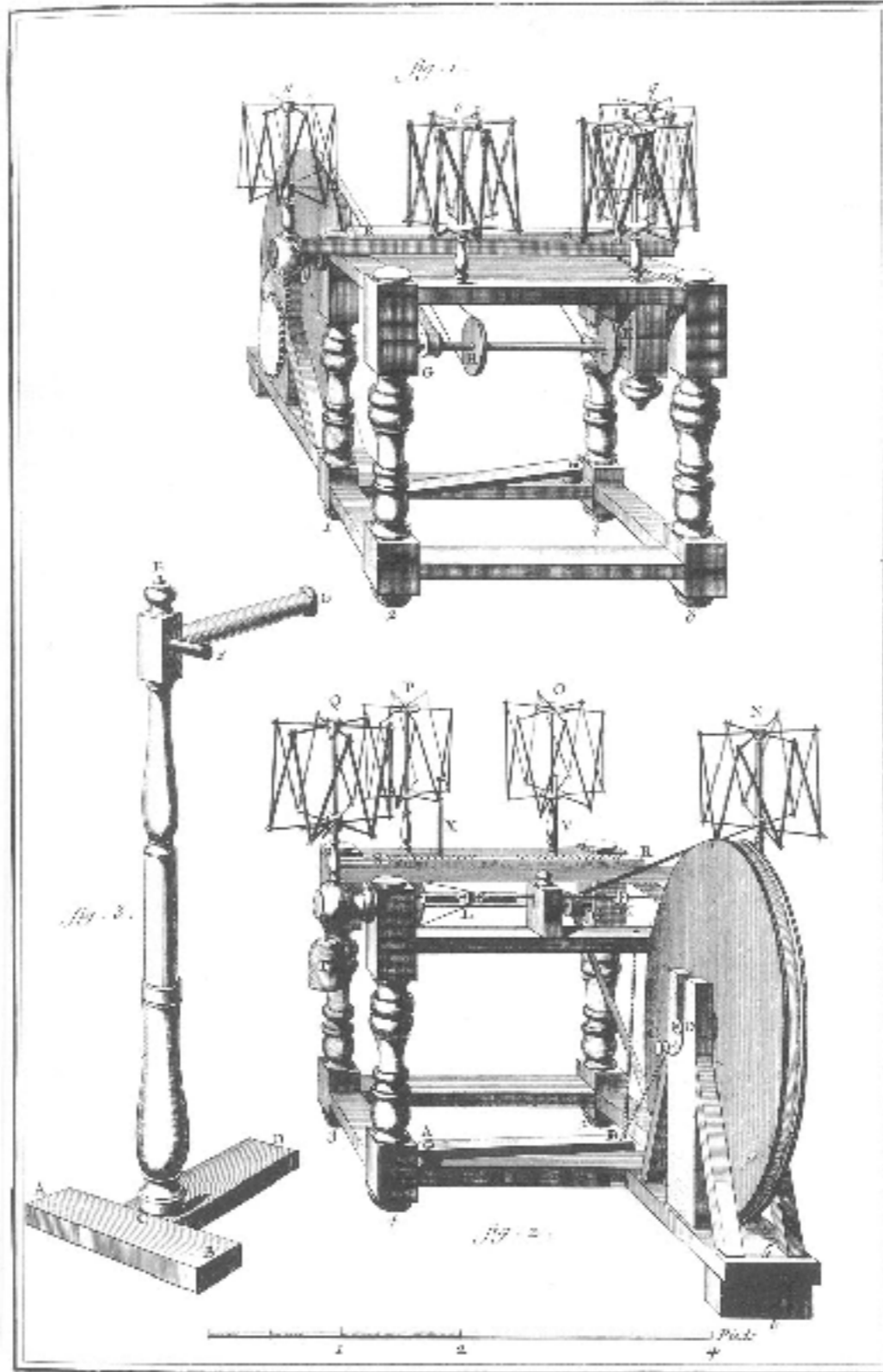
Soierie, Rouet de Lion en Perspective vu des deux côtés. X
