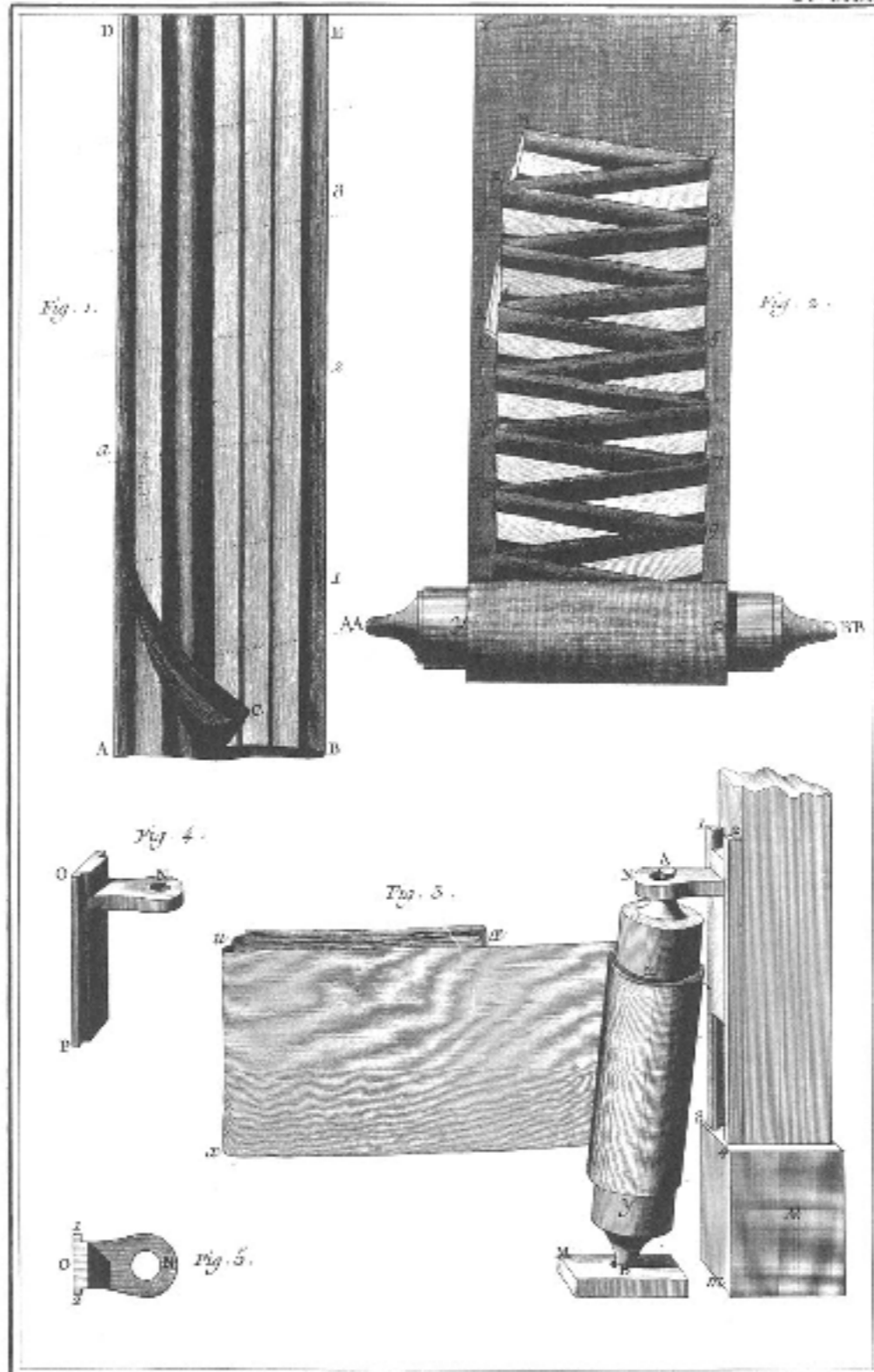
Soierie, Calandre. Maniere de Ployer les Etoffes qui doivent être Mairées et Développement et usage du Valet.
