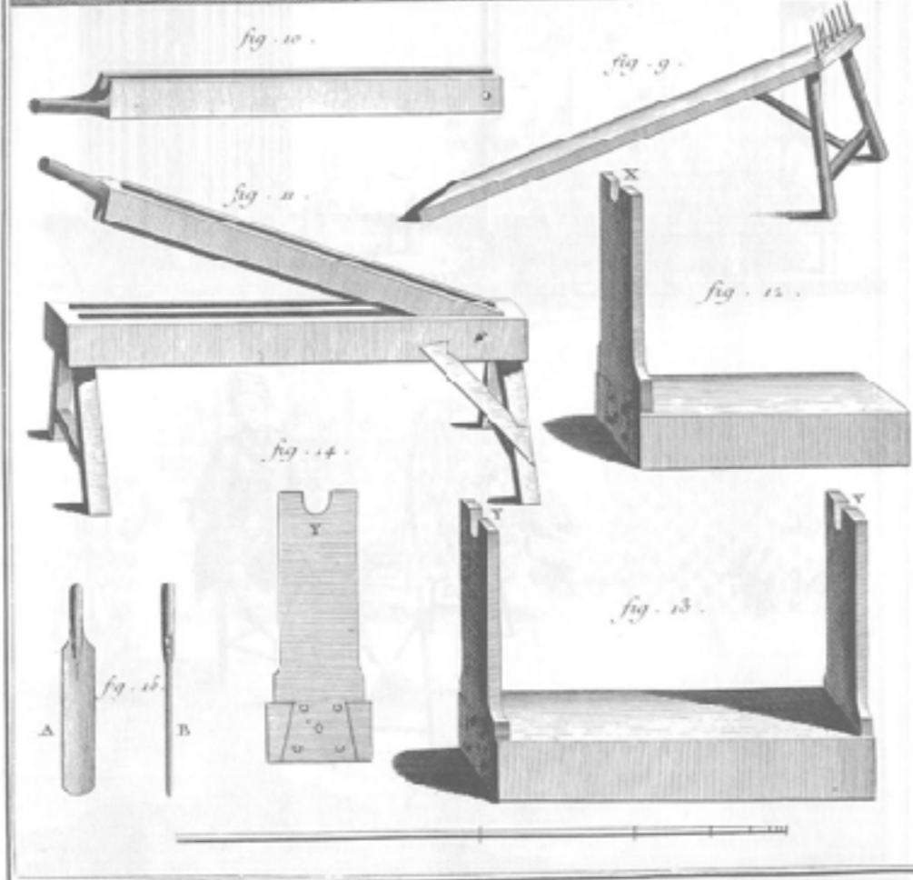
OEconomie Rustique, Culture et Travail du Charreux.
