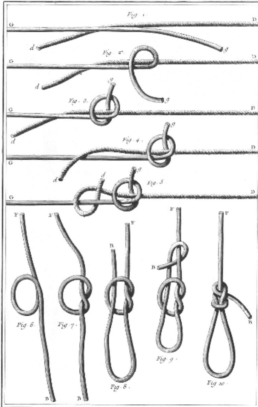
Soierie, Noeud Tirant et Noeud Coulant, les différents temps de leur formation.
