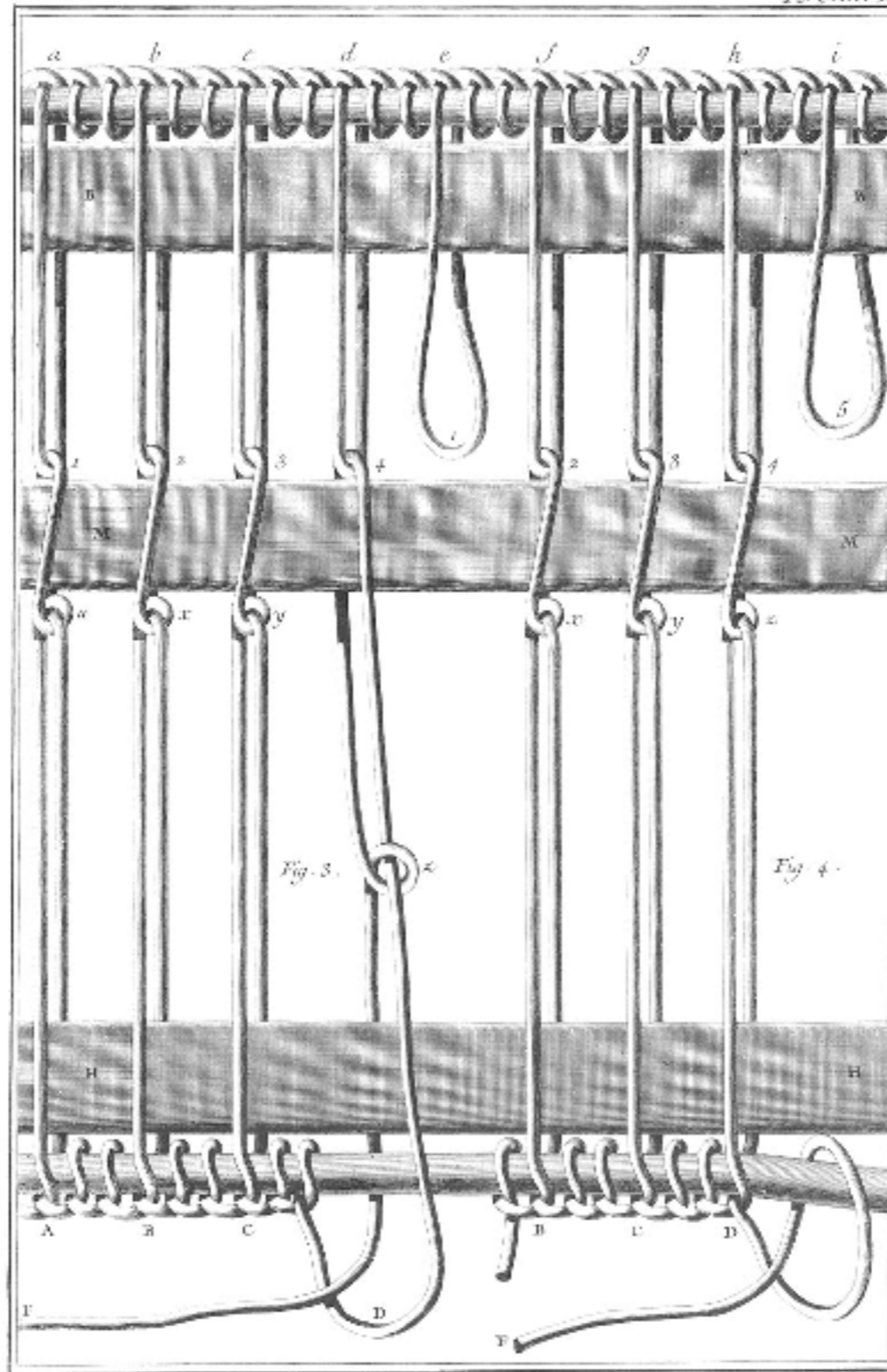
Soierie, Lissas à Nœuds, troisième et quatrième temps de la formation de la maille. R. R. R. R.
