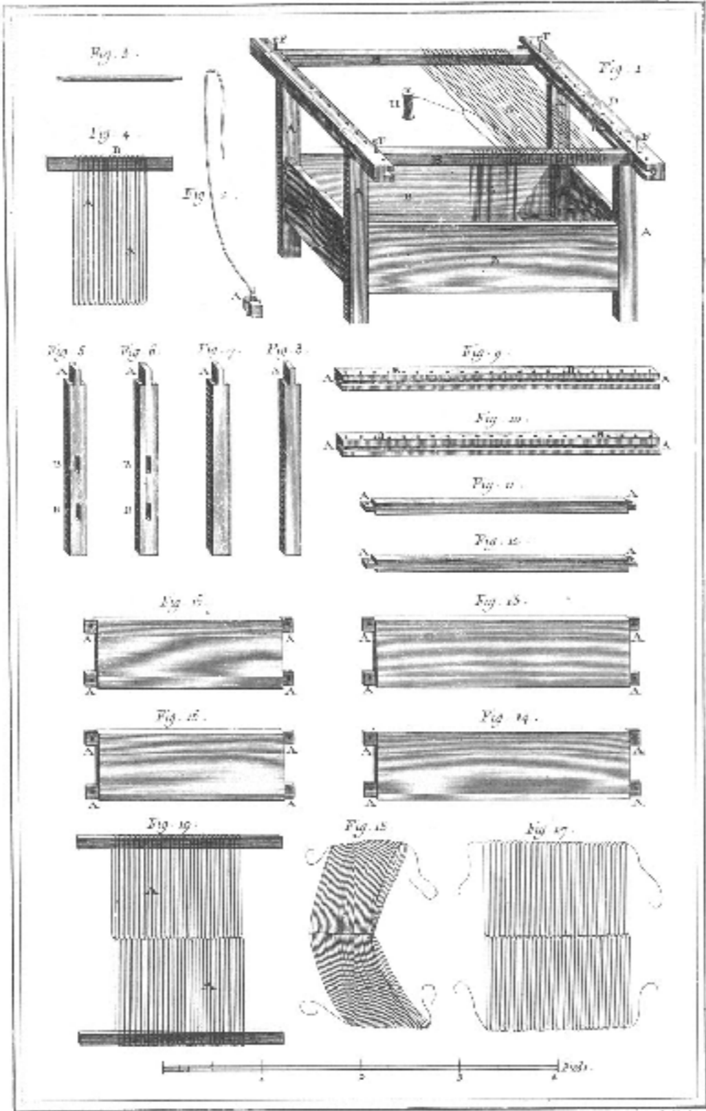
Passenterie, Détails pour la façon des Liffes.
