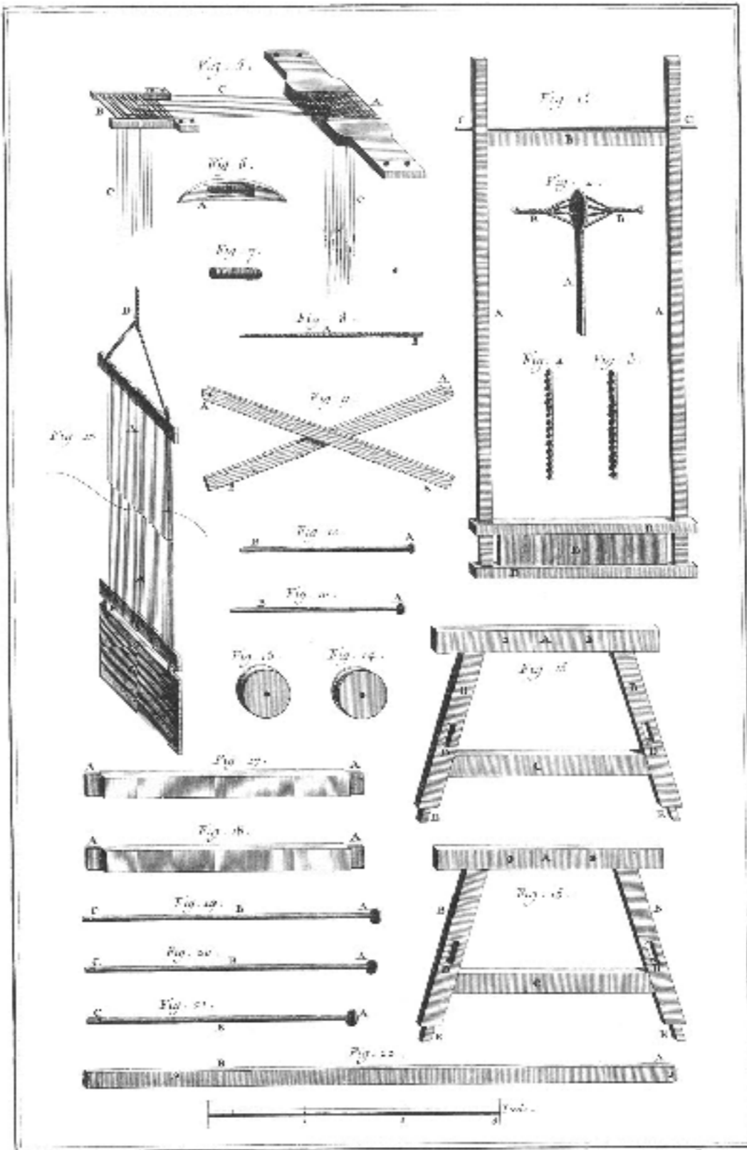
Passementerie, détail du Mètre à Galon
