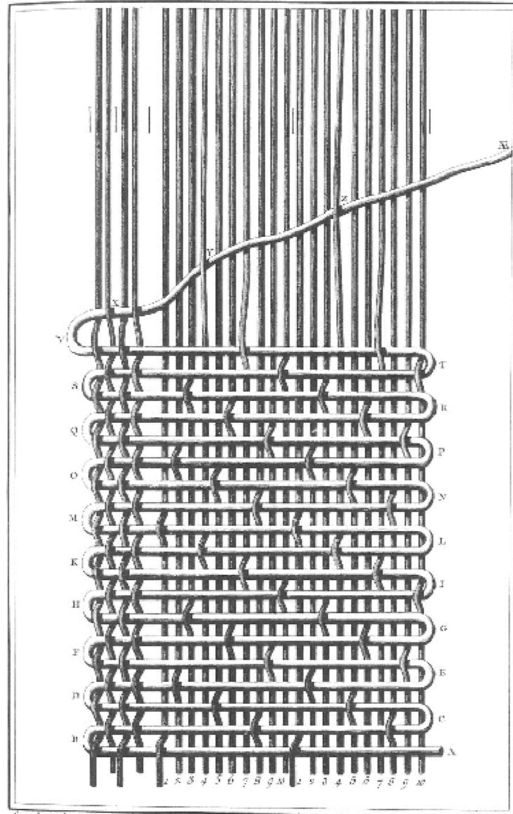
Soierie, Etoffe en Plein, Satin à dix Lisses Vu du côté de l'envers.
