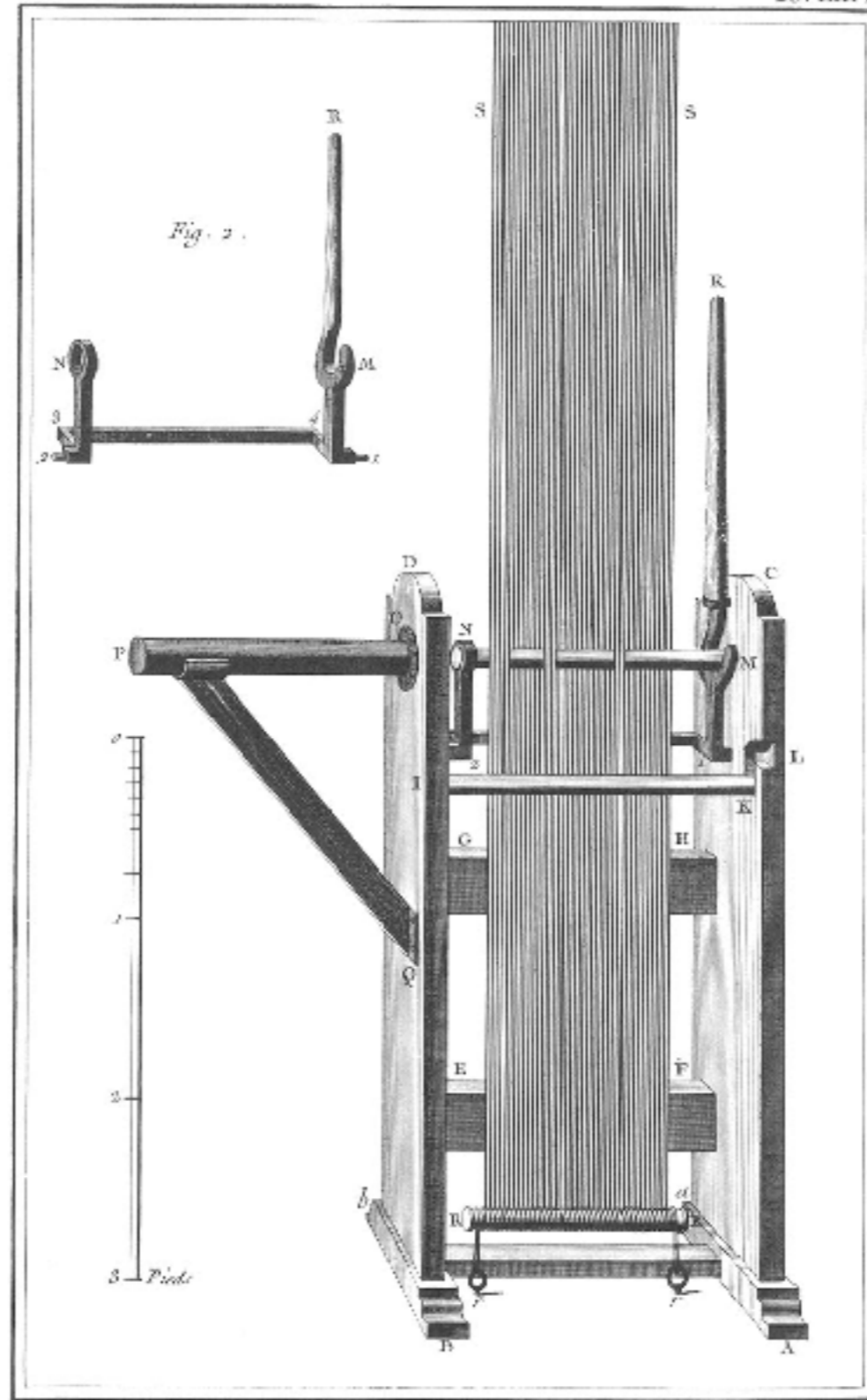
Soierie, Nouvelle Machine pour la Tirc.
