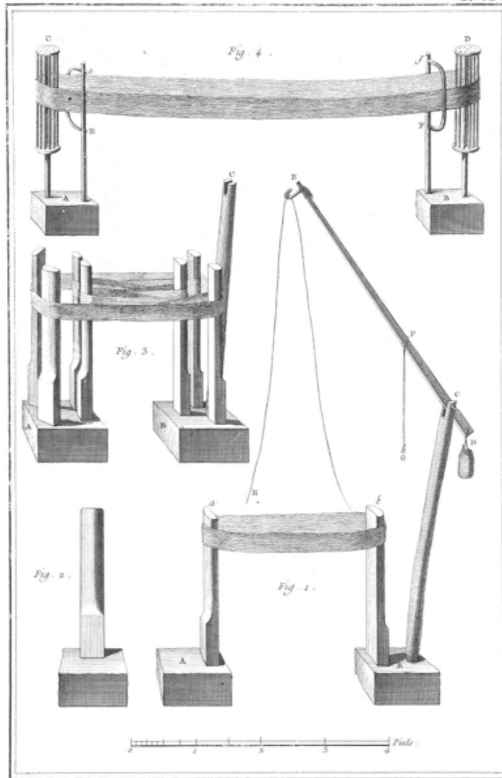
Soierie, Dévidage de la Soie, Tour d'Espagne, Campanas &c. F
