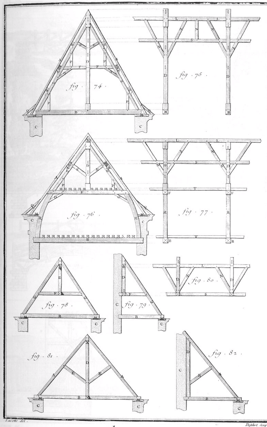
Charpente, Combles à un et deux égouts.
