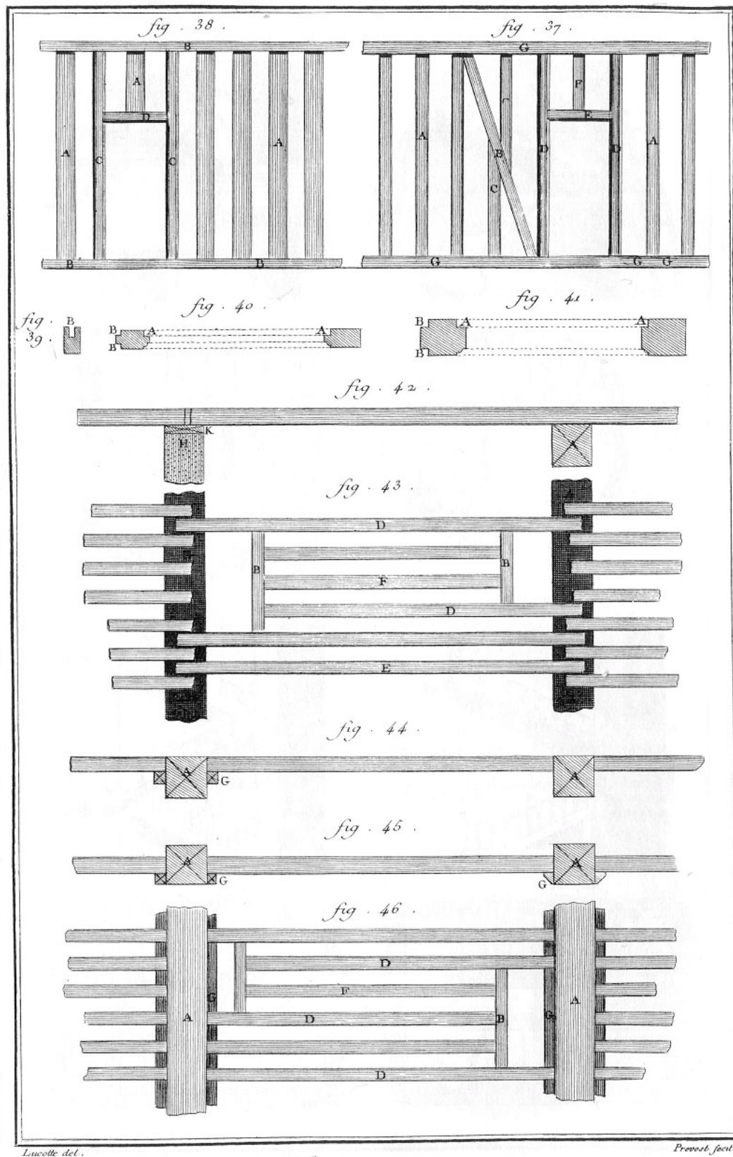
Charpente, Cloisons et Planchers .
