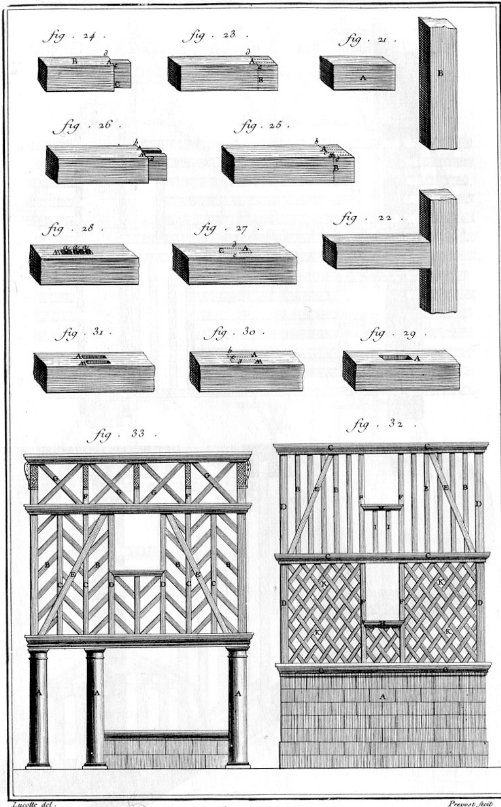
Charpente, Assemblages et pans de bois anciens.
