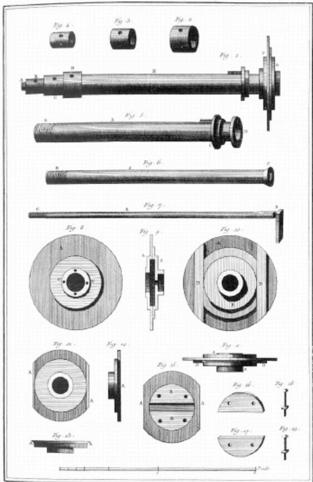
Tourneur, Arbres pour les Tours Ovales.
