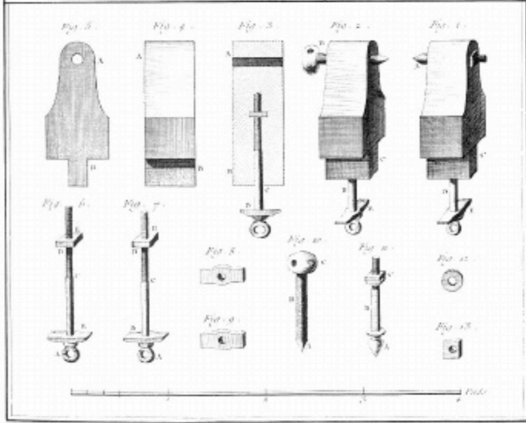
Tourneur, Tour en Fer
