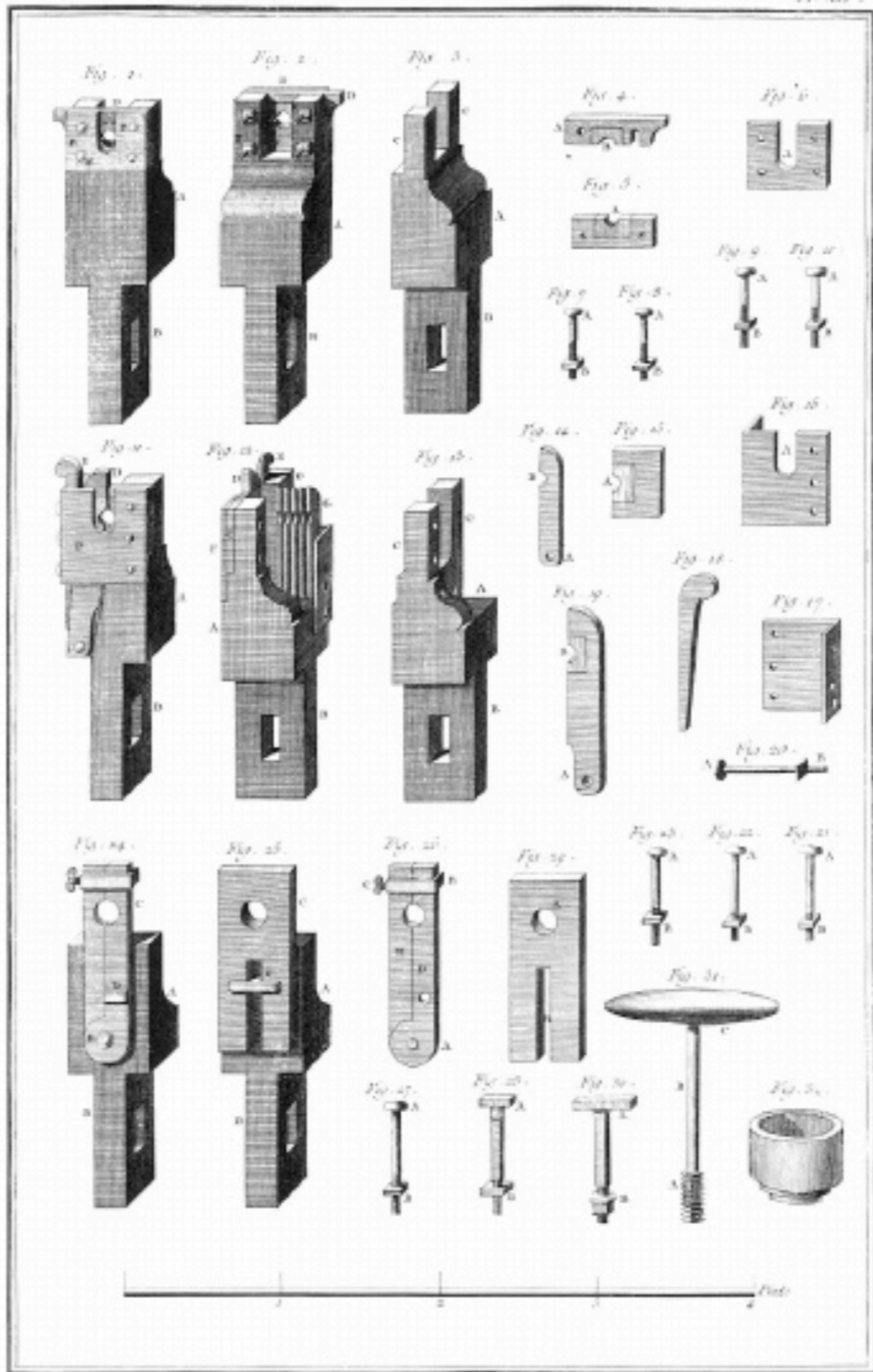
Tourneur, Propriété de Leclercq pour Tour en Lait.
