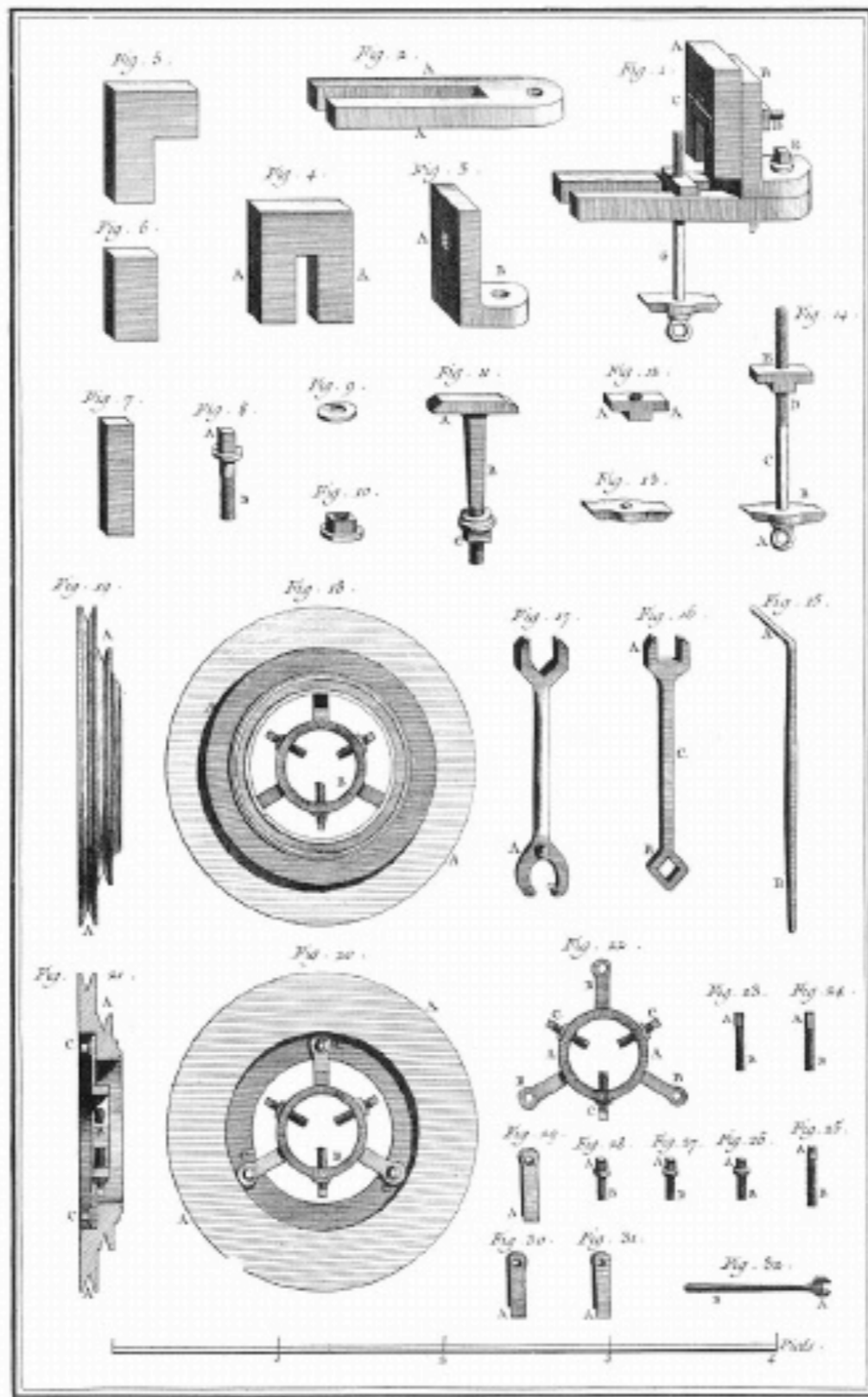
Tourneur, Tour en Per.
