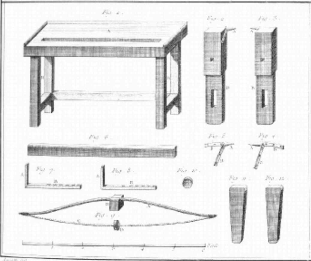
Tourneur, Tour en Bois.
