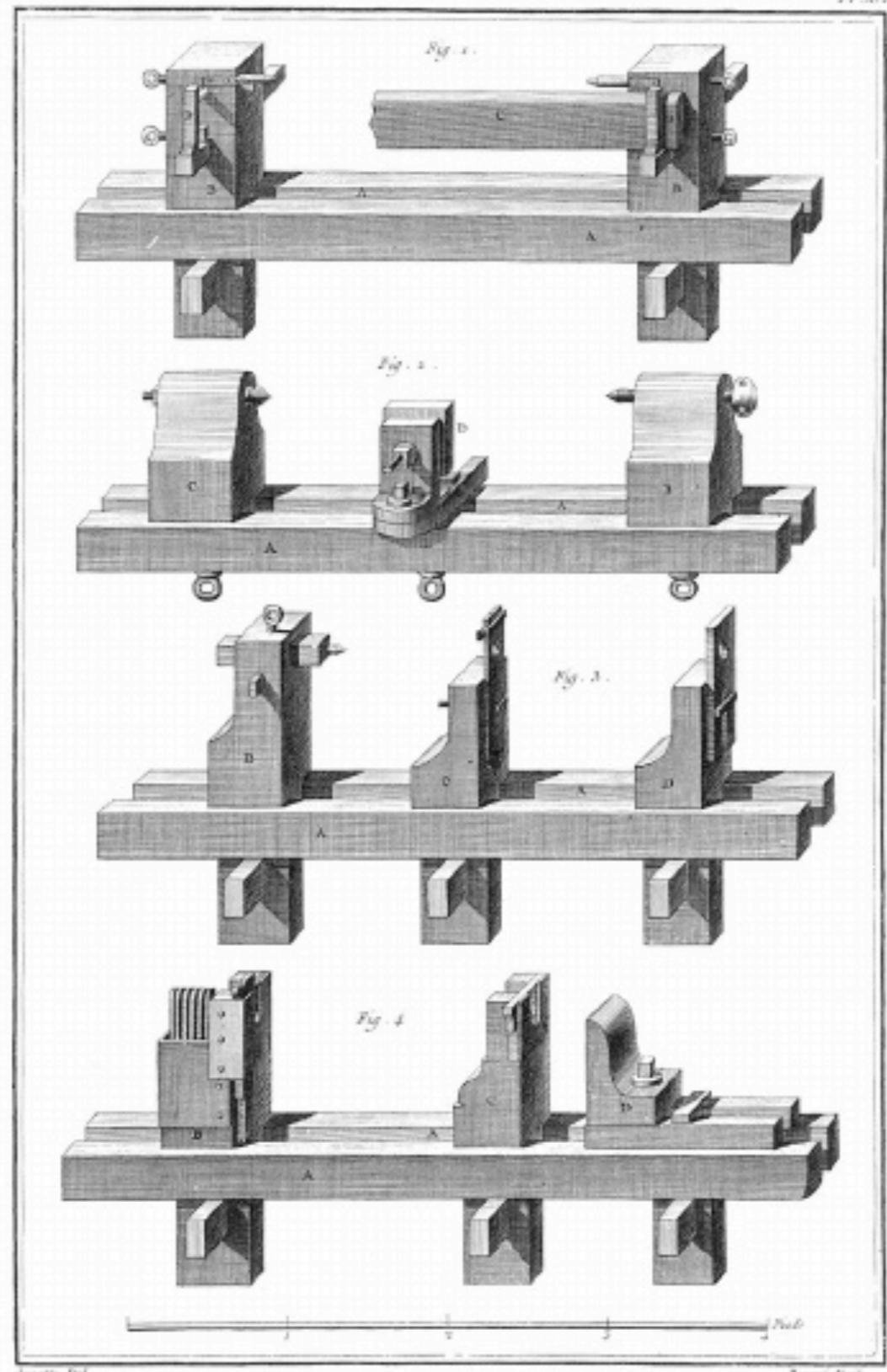
Tourneur, Tour de Menuisier.
