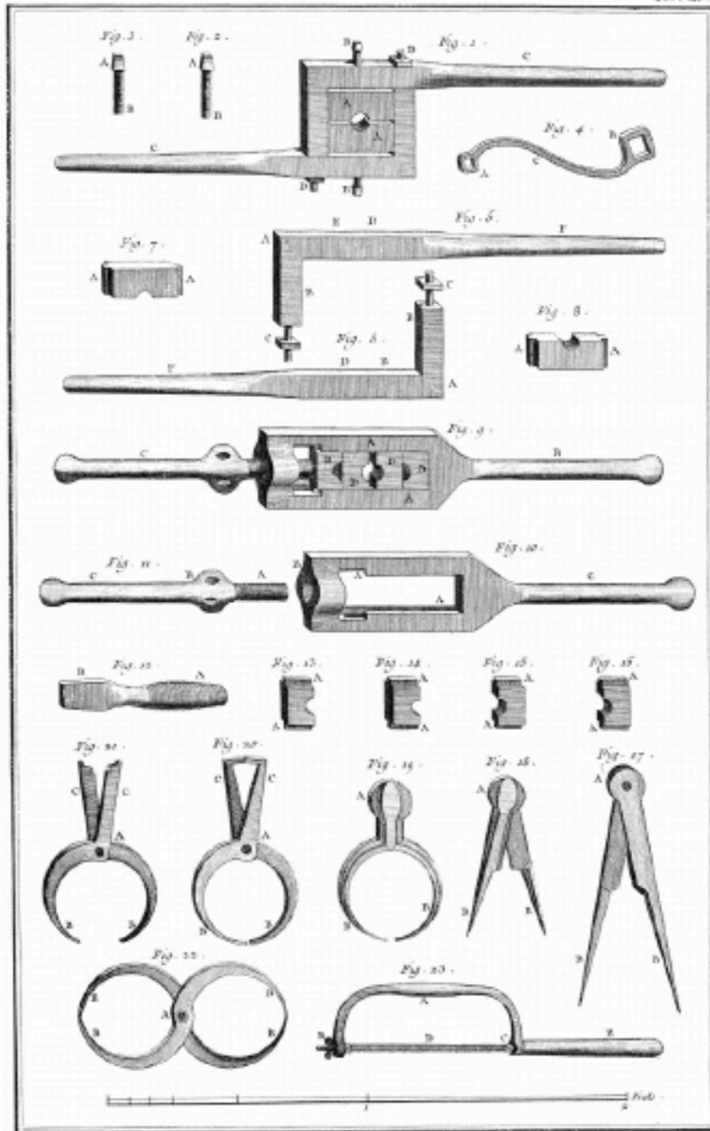
Tourneur, Filères, Tarots et Compas.
