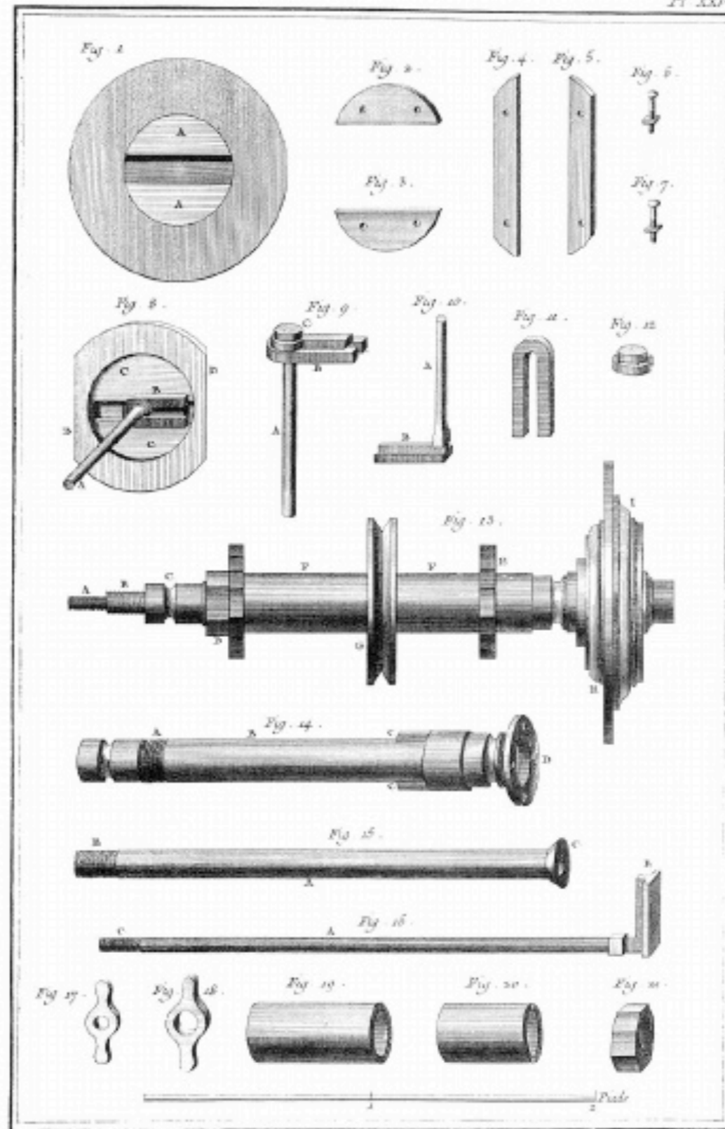
Tourneur, arbres pour les Tours creale.
