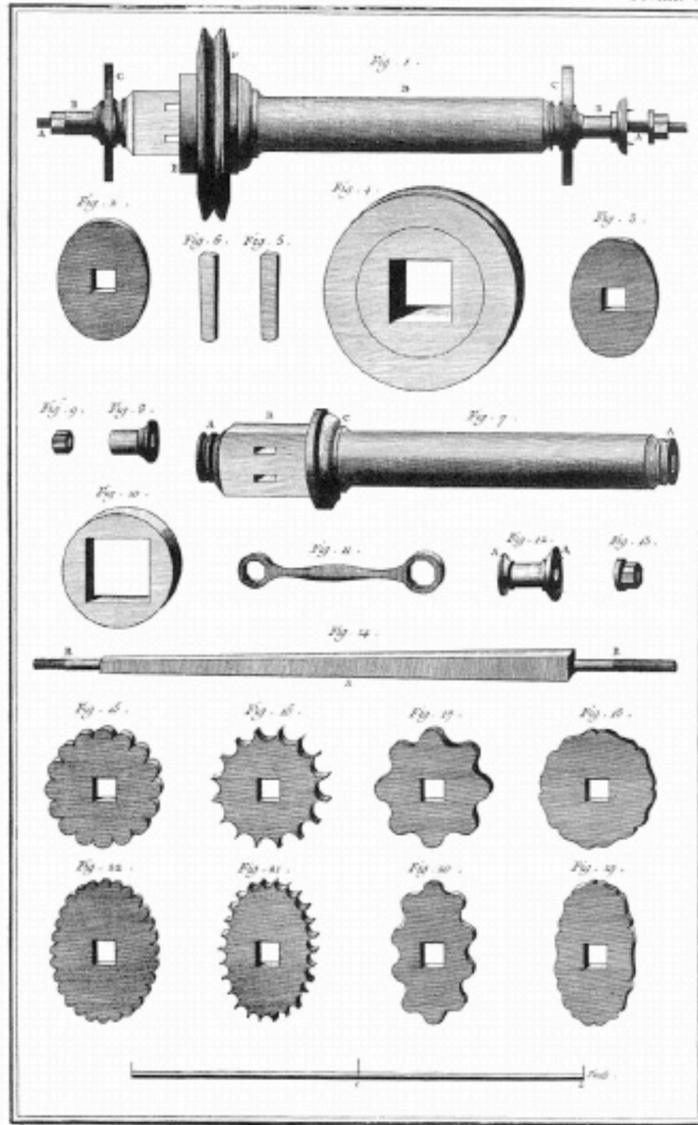
Tourneur, Arbre et dépendances.
