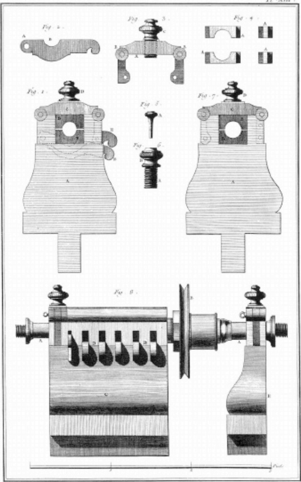
Tourneur, Tour en l'air.
