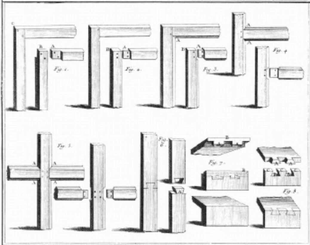
Menuiserie.
