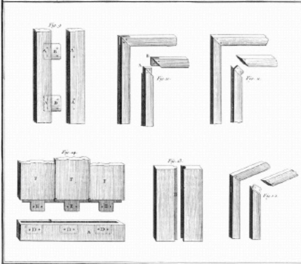
Menuiserie.
