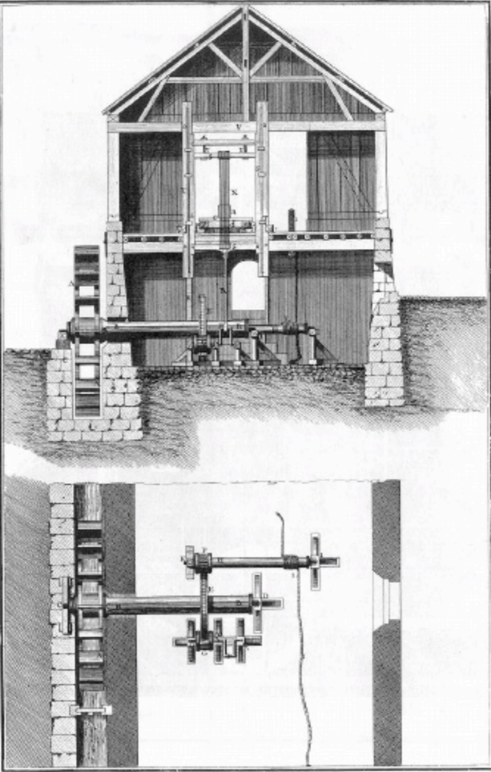
Charpente, Moulin pour Scier le Bois.
